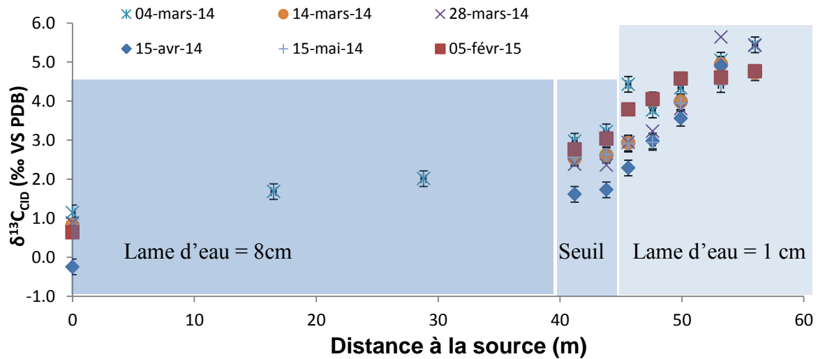
Figure III-32 Evolution du δ 13 C du CID en fonction de la distance à la source.
