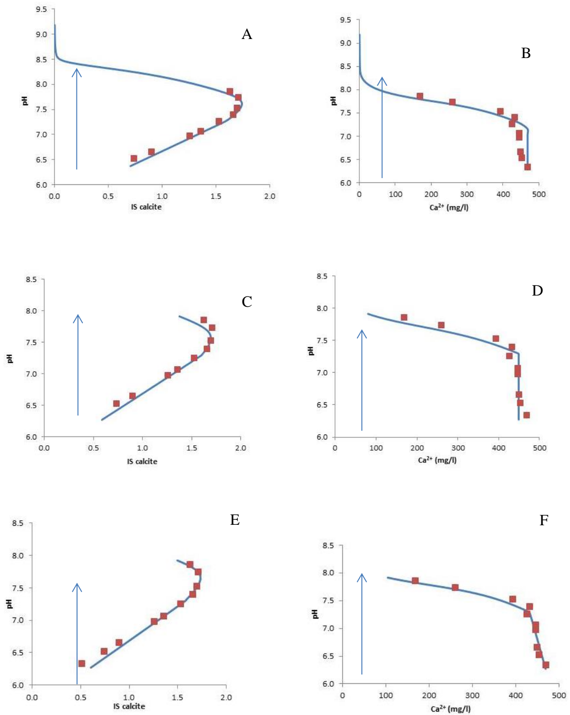
Figure IV-2 Calage du modèle de Plummer sur l'évolution pH en fonction de Ca 2+ et pH en fonction de l'IS calcite, pour la campagne du 4 mars 2014. En haut avec un modèle unique, avec les mêmes valeurs de k et A/V. En C, D, E et F avec un A/V différent au bout de 40 m, pour C et D, k=5.10 -5 m 3 .s -1 et A/V=9 cm -1 , pour E et F, k=5.10 -6 m 3 .s -1 et A/V=0,9 cm -1 .
