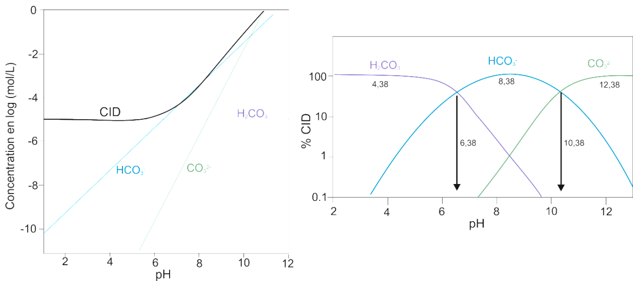
Figure I-4 Equilibre calco-carbonique (diagramme de Sillen). Evolution des trois espèces de carbone inorganique dissout en fonction du pH, à gauche en système ouvert, à droite en système fermé.
