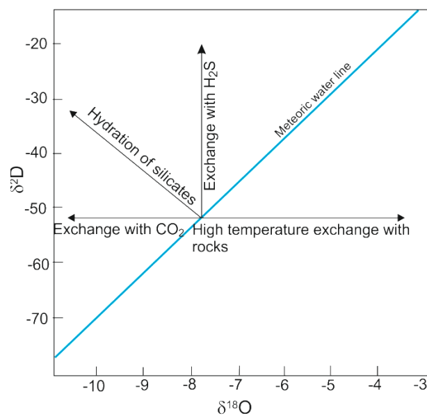
Figure III-17 Evolution de la signature isotopique de l'eau en fonction des principaux processus géologique (extrait de Clark et Fritz, 1997)
