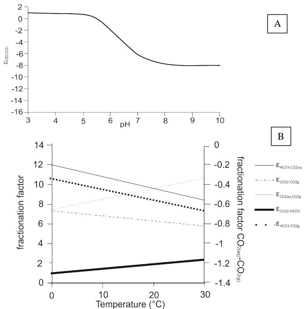
Figure II-3 A. Evolution du facteur de fractionnement \text{CO}_2 -CID en fonction du pH. B. Evolution des différents facteurs de fractionnement du carbone 13 des espèces de CID en fonction de la température.
