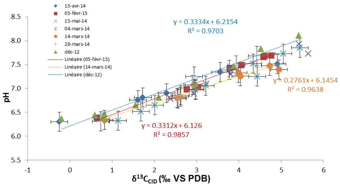
Figure III-33 Evolution du pH en fonction du δ 13 C du CID avec les trois droites de tendances (moyenne, minimale et maximale)
