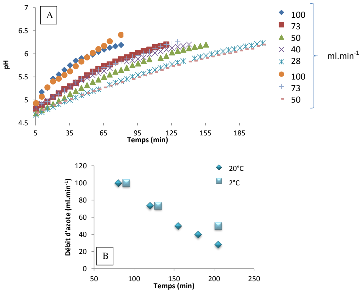
Figure II-30 A. Evolution du pH en fonction du temps et en fonction des différents débits d'azote. B. Temps de fin des expérimentations en fonction des débits d'azote et pour les deux températures.
