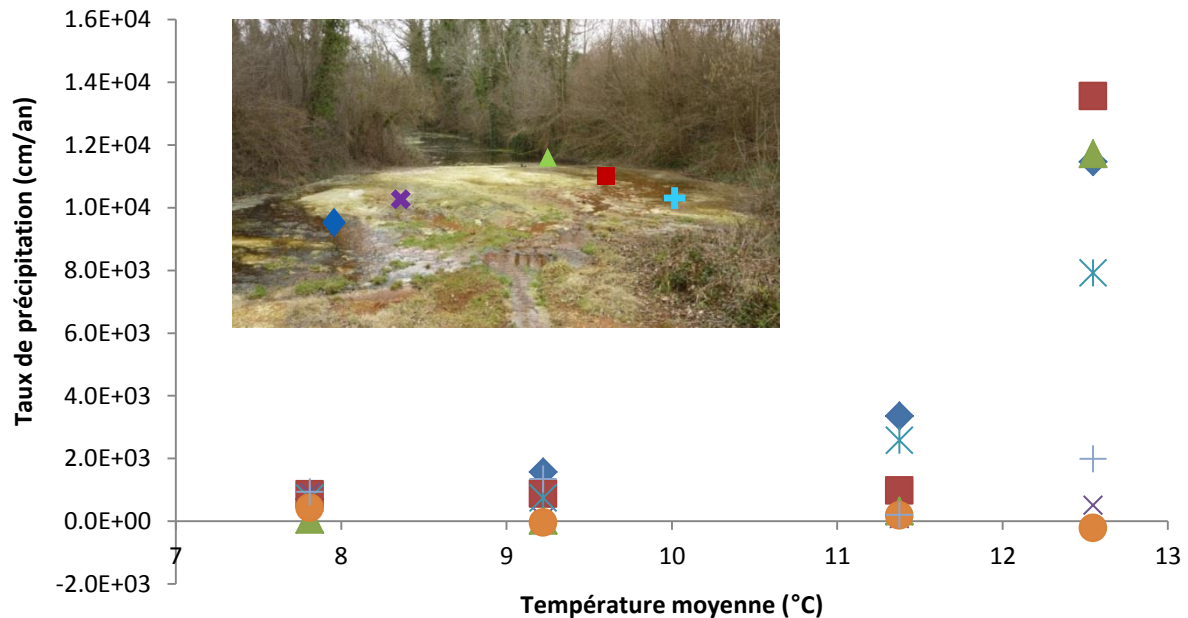
Figure III-24 Variation du taux de précipitation en fonction de la température moyenne de la période de précipitation. Les différents points correspondent aux différentes localisations de prélèvement.
