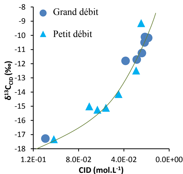
Figure II-26 Evolution du \delta^{13}\text{C} du CID en fonction de la perte de carbone, pour les deux vitesses de dégazage (80 et 28 \text{ml} \cdot \text{min}^{-1} ).
