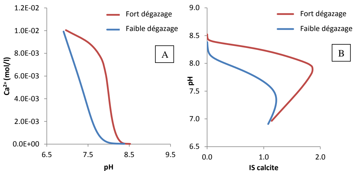
Figure II-9 Variation de la vitesse de dégazage sur l'évolution de [Ca^{2+}] (A) et du pH (B).
