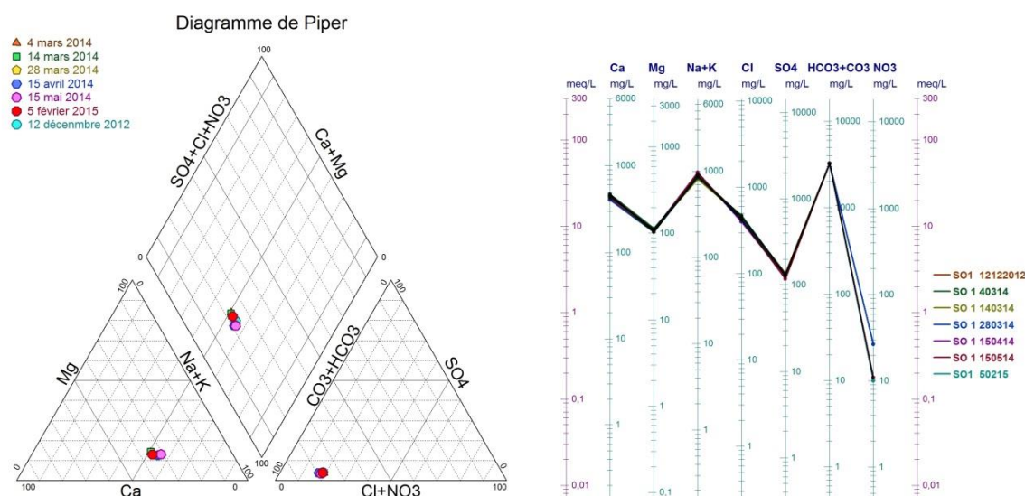
Figure III-11 Diagramme de Piper avec l'eau de la Source de l'Ours. A droite diagramme de Schöeller Berkloff avec les proportions relatives de chaque élément
