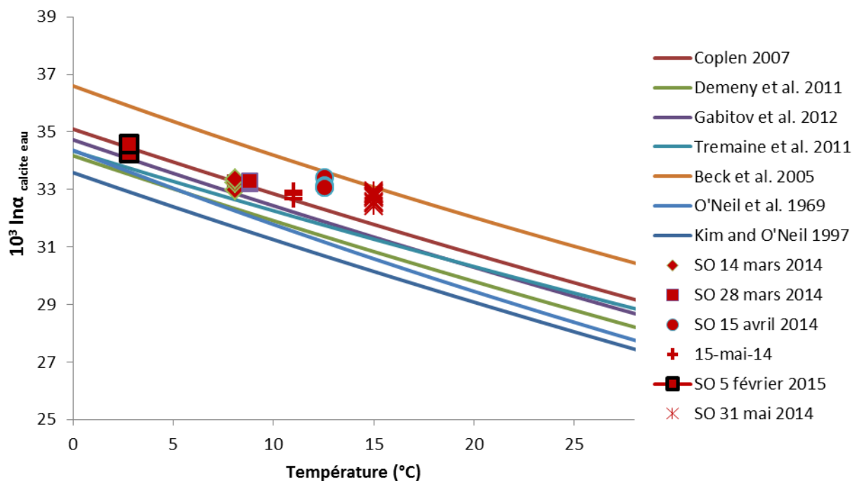
Figure III-47 1000 \ln \alpha en fonction de la température avec les droites d'équilibre et les points de la source de l'Ours.
