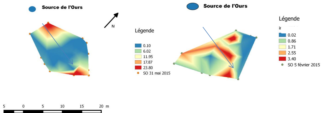
Figure III-26 Comparaison de l'évolution spatiale du taux de précipitation (en \text{cm}\cdot\text{an}^{-1} ). A droite, prélèvement le 5 février 2015, à gauche le 31 mai 2014. La flèche représente la ligne d'écoulement.
