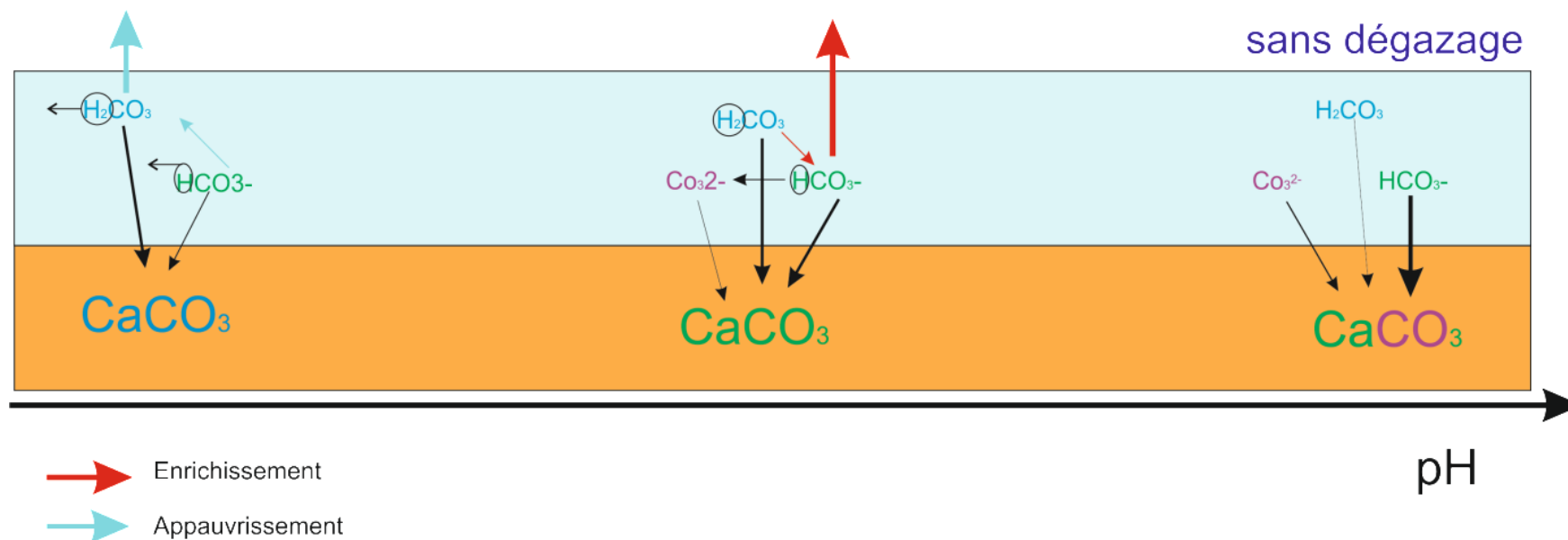
Figure IV-9 Schéma récapitulatif des mécanismes de précipitation pour les espèces de carbone portant le carbone 13. La taille des flèches noire est proportionnelle à la quantité de l'espèce incorporée.
