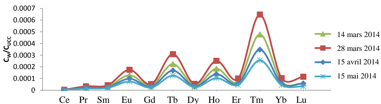
Figure III-14 Variation de la concentration en ETR.
