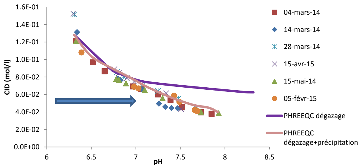
Figure III-21 Evolution du CID en fonction du pH avec les modèles réalisés sous PHREEQC et la flèche représentant le début de la précipitation.
