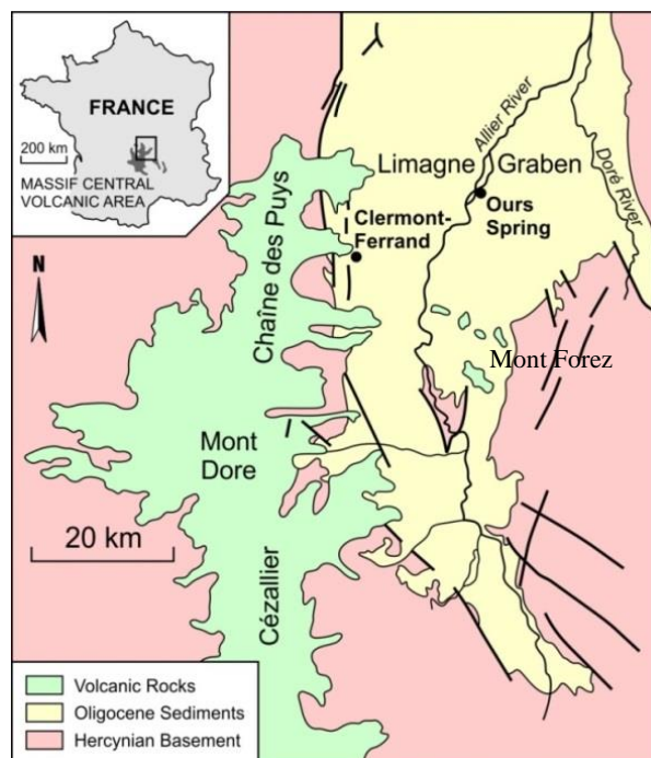
Figure III-3 Carte géologique simplifiée du Massif Central (modifiée de Condomines and Rihs (2006))
