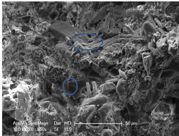
Figure IX-3 Image au MEB représentant les diatomées. La structure est détritique.
