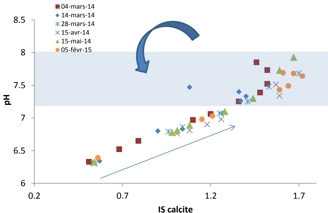
Figure III-22 Evolution du pH en fonction de l'indice de saturation. La ligne bleue marque le début de la précipitation.
