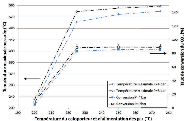
FIGURE II.10 – Evolutions de la température maximale mesurée et du taux de conversion de \text{CO}_2 en fonction des températures d'alimentation de gaz et du caloporteur sous différentes pressions avec le réacteur-échangeur à lit fixe annulaire. (Débits \text{H}_2 ; \text{CO}_2 ; \text{Ar} : 20; 5; 50 \text{NL}/\text{min} )
