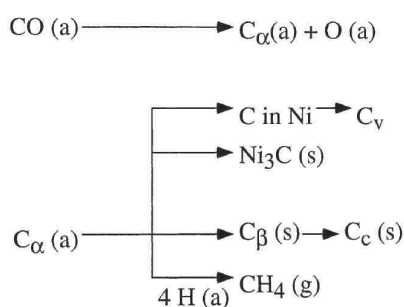
FIGURE I.8 – Mécanisme de formation et de transformation des dépôts de carbone à partir de la dissociation du CO (Bartholomew 2001).
