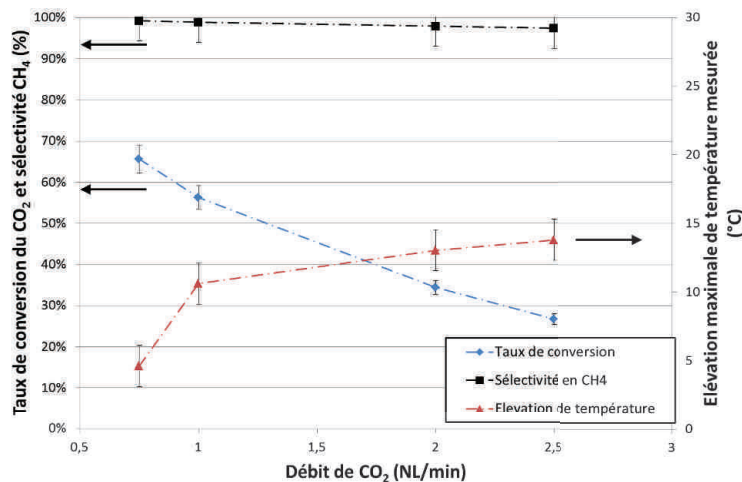
FIGURE II.31 – Evolution du taux de conversion de CO 2 , de la sélectivité en CH 4 et de l'élévation de température maximale mesurée en fonction du débit d'alimentation de CO 2 (H 2 stœchiométrique). (Conditions : P=15 bar - T=325°C)
