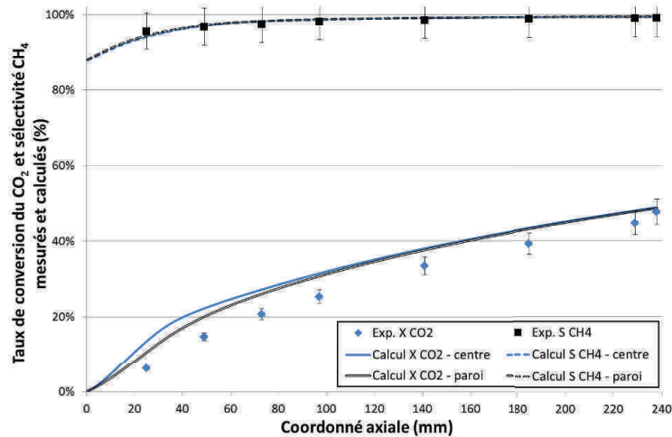
FIGURE III.25 – Profils de conversion du \text{CO}_2 et de sélectivité en \text{CH}_4 mesurés et calculés le long du réacteur-échangeur à lit fixe milli-structuré lors du premier essai avec prélèvement de gaz. (Conditions : P=4 bar - T=265^\circ\text{C} - Débits \text{H}_2 ; \text{CO}_2 : 20 ; 5 NL/min)
