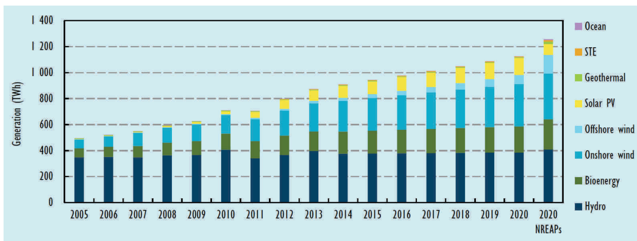
FIGURE 1 – Evolution de la production annuelle d'électricité à partir de sources renouvelables dans l'Union Européenne de 2005 à 2013 et prévisions de l'Agence Internationale de l'Energie (AIE) et de la commission européenne (NREAPs : National Renewable Energy Action Plans) (AIE 2014).
