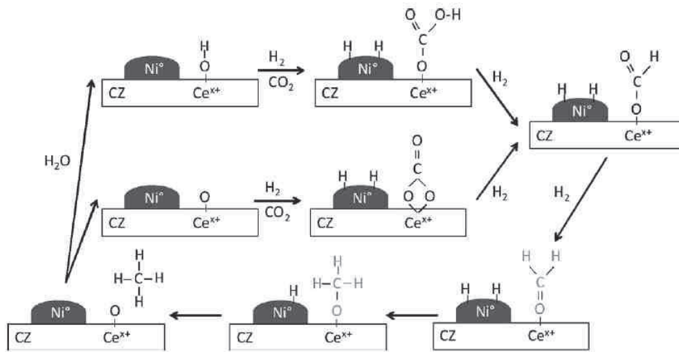
FIGURE I.4 – Mécanisme de la réaction d'hydrogénation du CO 2 proposé par Aldana et al. (2013).
