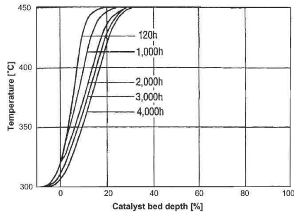
FIGURE I.17 – Profil de température dans le premier réacteur du procédé de méthanation Lurgi en fonction du temps d'utilisation (Kopyscinski 2010).
