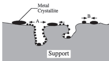
FIGURE I.12 – Illustration des mécanismes de frittage des cristallites métalliques : (A) - par migration atomique ; (B) - par migration et coalescence des cristallites (Bartholomew 2001).
