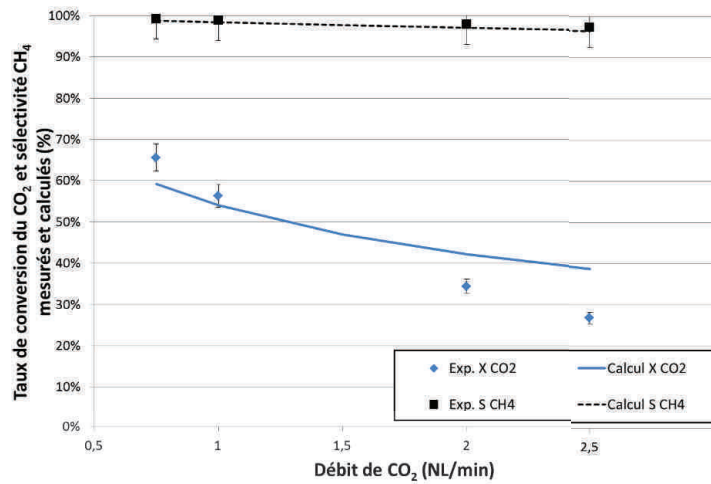
FIGURE III.44 – Evolution du taux de conversion du CO 2 et de la sélectivité en méthane calculés et mesurés en fonction du débit d’alimentation de CO 2 (H 2 stœchiométrique). ( Conditions : P=15 bar - T=325°C )
