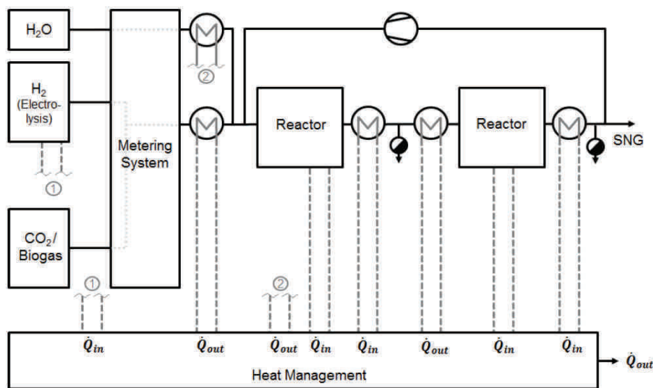
FIGURE I.28 – Schéma du procédé de Power-to-SNG d'ETOGAS dans le démonstrateur de 25 kW (2009) (Zuberbühler et al. 2015).
