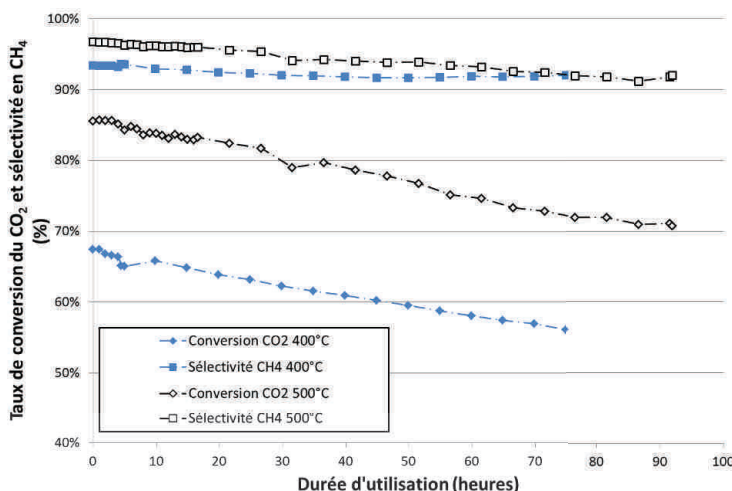
FIGURE II.32 – Evolution du taux de conversion de \text{CO}_2 et de la sélectivité en \text{CH}_4 en fonction du temps d'utilisation lors des essais de vieillissement réalisés à petite échelle. (Conditions : P = 2,5 \text{ bar} - Débits \text{H}_2 ; \text{CO}_2 ; \text{N}_2 = 70 ; 13,2 ; 3,5 \text{ NmL/min} )
