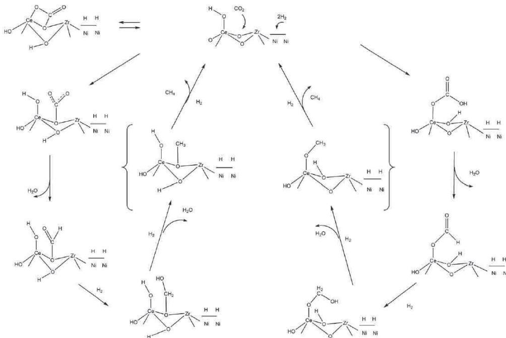
FIGURE I.5 – Mécanisme de la réaction d'hydrogénation du CO 2 proposé par Pan et al. (2014).
