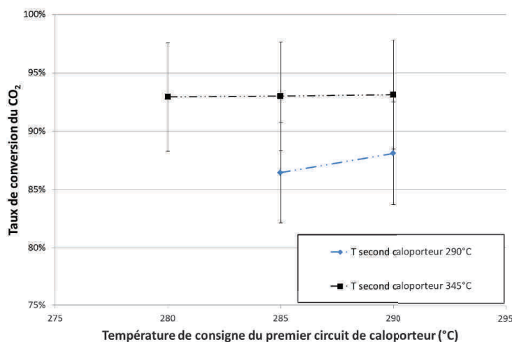
FIGURE II.25 – Evolution du taux de conversion de CO 2 en fonction de la température du premier circuit de caloporteur lors de l’essai de simulation de la désactivation du catalyseur.
