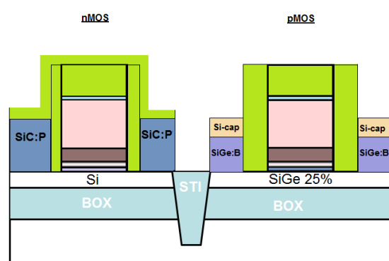
10) Drive-in anneal
