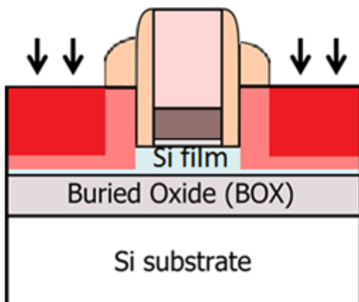
7) HDD Implantation
