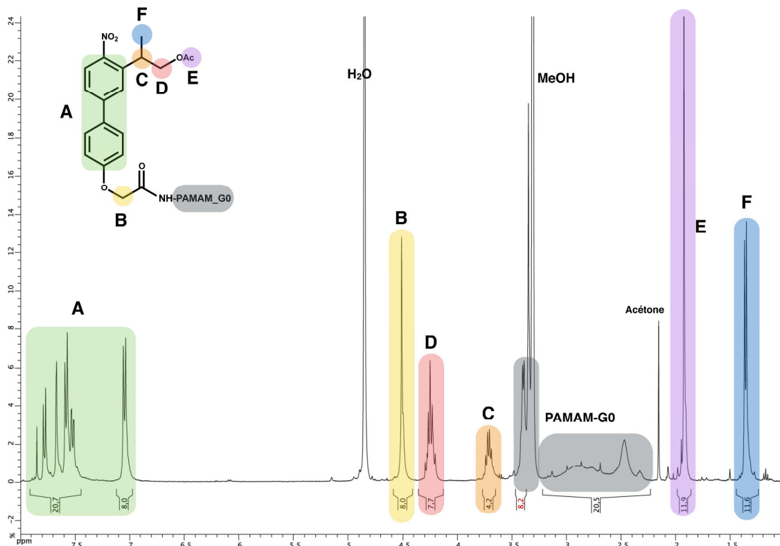
Figure 50. Spectre RMN ^1\text{H} dans \text{MeOD}_4 du NPG0 (18G0).
