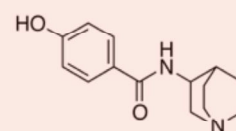
Figure 81. Molécules soumises au « docking » avec le récepteur \alpha 7^{L141F} .
