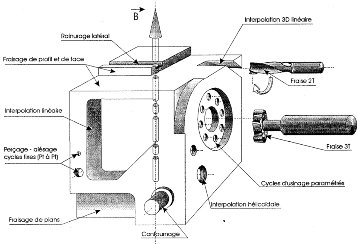
FIGURE 2.1 – Possibilités d'usinage à l'aide d'un centre 4 axes [ACMV97]
