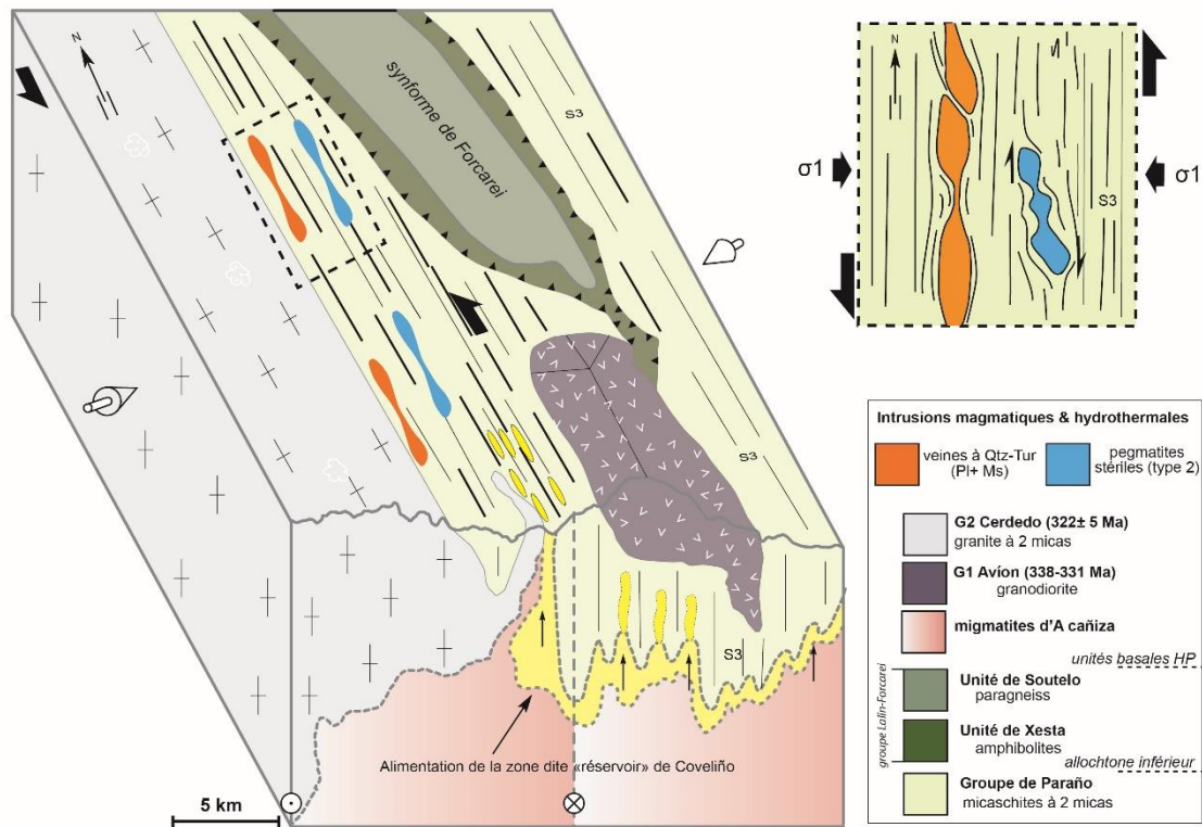
Figure III-32: Remontée du front de fusion partielle et mise en place des pegmatites de type 2' dans la zone Sud de Coveliño pendant le raccourcissement horizontal E-O. Les veines hydrothermales et magmatiques au préalable consolidées sont déformées par l'activation du décrochement planaire senestre.
