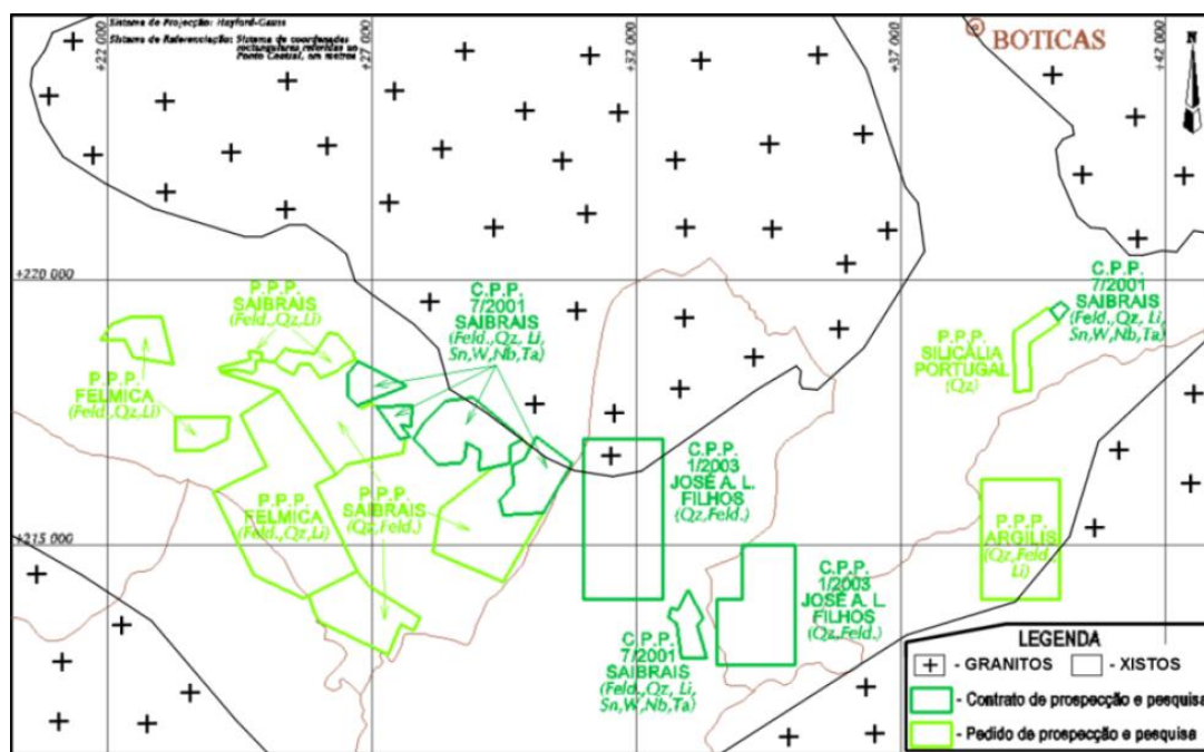
Figure II-17: Répartition et délimitation des concessions attribuées pour la prospection des pegmatites granitiques lithinifères dans la région de Barroso - Alvão (Nord-Portugal). Carte disponible sur site du Laboratório Nacional de Energia e Geologia (LNEG).
