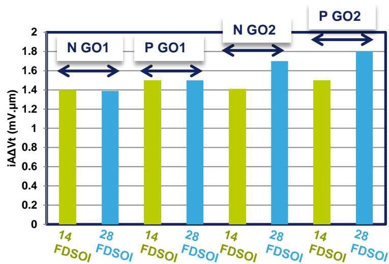
Figure B.24: Les valeurs moyennes de i\Delta V_t ( mV \cdot \mu m ) pour les technologies 28 et 14 nm
