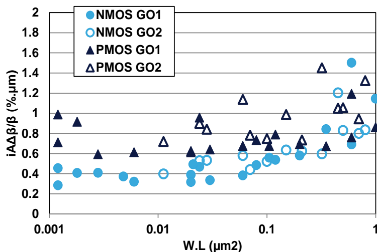
Figure B.22 : Comparaison de i\Delta\Delta\beta/\beta ( \%\cdot\mu\text{m} ) en fonction de la surface des transistors W.L ( \mu\text{m}^2 ) entre les GO1 et GO2 pour les dispositifs NMOS et PMOS de la technologie 14nm FD SOI
