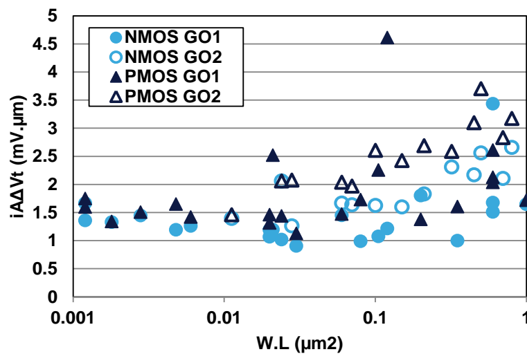
Figure B.21 : Comparaison de i\Delta\Delta V_t ( \text{mV}\cdot\mu\text{m} ) en fonction de la surface des transistors W.L ( \mu\text{m}^2 ) entre les GO1 et GO2 pour les dispositifs NMOS et PMOS de la technologie 14nm FD SOI
