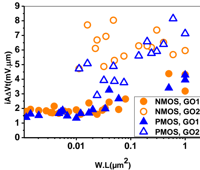
Figure B.17 : Comparaison de iA_{\Delta V_t} ( \text{mV} \cdot \mu\text{m} ) en fonction de la surface des transistors ( W.L ( \mu\text{m}^2 )) entre les dispositifs GO1 et GO2 pour les transistors NMOS et PMOS de la technologie 20nm Métal-Gate-Last
