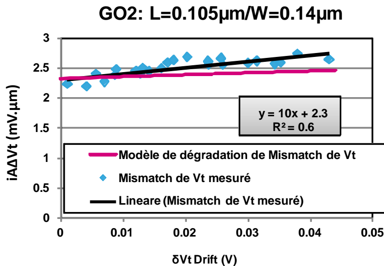
Figure B.27 : L=0.105\mu\text{m} and W=0.14\mu\text{m} : la constant individuelle de désappariement de Vt en fonction du drift de Vt : Comparaison entre les valeurs mesurées et le modèle théorique de l'équation B.8
