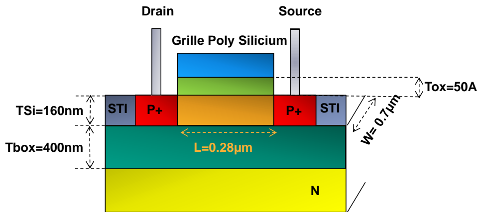
Figure B.5 : Transistor PMOS partiellement dépleté, contient un oxyde épais ( T_{ox}=50\text{Å} ) avec la géométrie L=0.28\mu\text{m} and W=0.7\mu\text{m}
