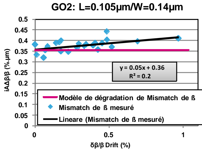
Figure B.28 : L=0.105\mu\text{m} and W=0.14\mu\text{m} : la constant individuelle de désappariement de \beta en fonction du drift de \beta : Comparaison entre les valeurs mesurées et le modèle théorique de l'équation B.9
