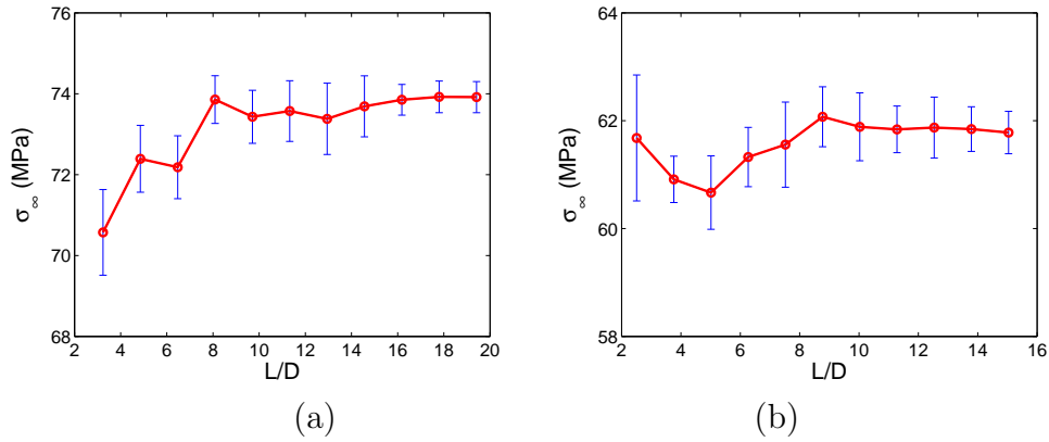
FIGURE 2.15 – Composite élasto-viscoplastique : convergence du paramètre \sigma_\infty par rapport au volume du VER, ou de manière équivalente par rapport à L/D ; (a) fraction volumique f = 0.3 ; (b) fraction volumique f = 0.5 .
