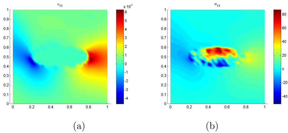
FIGURE 4.13 – Champs de contrainte et de déformation dans le VER anisotrope : (a) \varepsilon_{11} et (b) \sigma_{11} .
