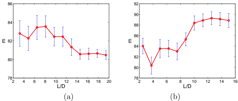
FIGURE 2.17 – Composite élasto-viscoplastique : convergence du paramètre m par rapport au volume du VER, ou de manière équivalente par rapport à L/D ; (a) fraction volumique f = 0.3 ; (b) fraction volumique f = 0.5 .
