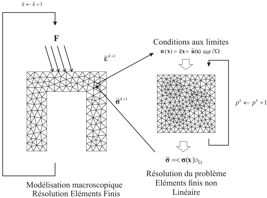
FIGURE 1.3 – Représentation schématique de la méthode (FE 2 ).
