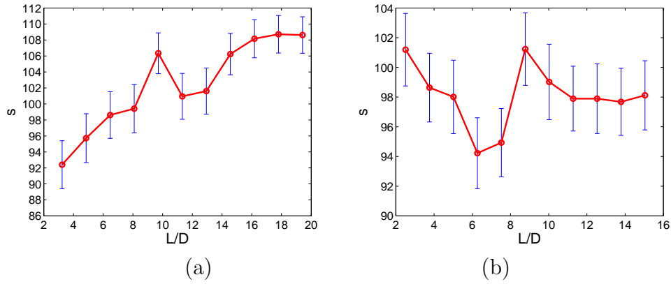
FIGURE 2.16 – Composite élasto-viscoplastique : convergence du paramètre s par rapport au volume du VER, ou de manière équivalente par rapport à L/D ; (a) fraction volumique f = 0.3 ; (b) fraction volumique f = 0.5 .
