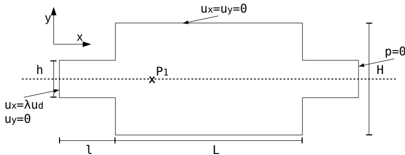
FIGURE 7.19 – Cas de l'écoulement dans une expansion soudaine suivi d'une contraction soudaine : h = 10, H = 30, l = l_{in} = l_{out} = 3h, L = 8h
