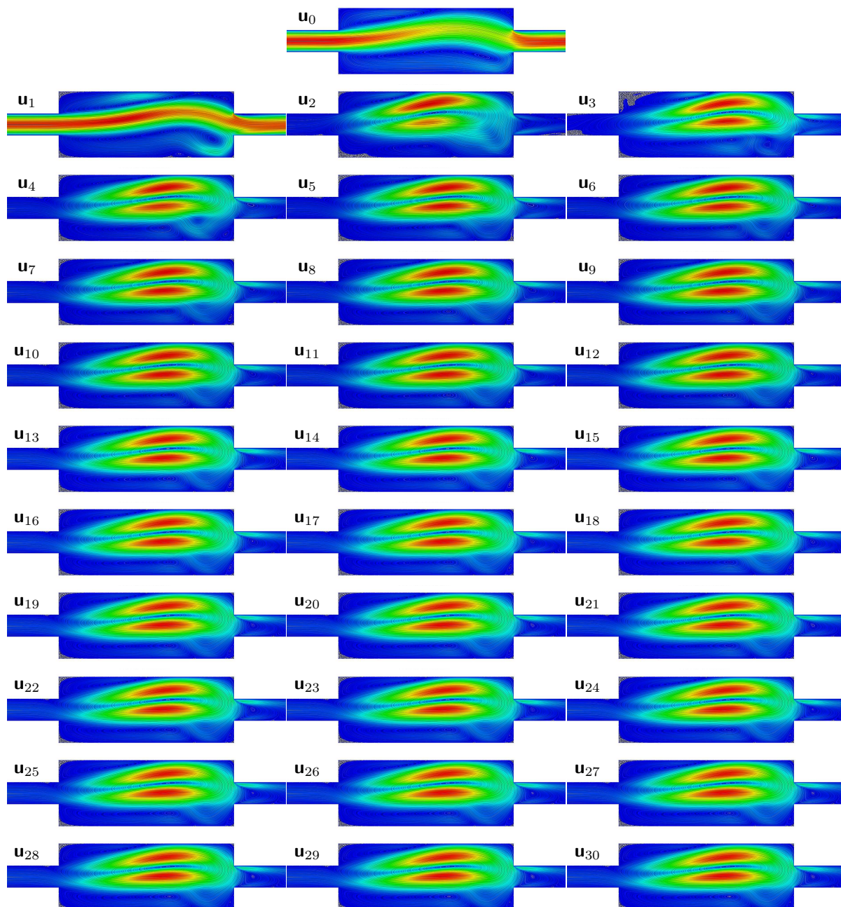
FIGURE 7.32 – Lignes de courants des champs de vitesse normés pour tous les termes de série obtenus au point solution (c) Fig.(7.20) sur la branche BB11 à l’approche du point limite et avant le point tournant à Re = 90 .
