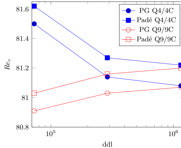
FIGURE 7.11 – Évolution du nombre de Reynolds critique en fonction du nombre de degrés de liberté pour deux types d'éléments fini. Cas de l'expansion soudaine E = 3 avec les paramètres MAN N = 30, \eta = 10^{-14} .
