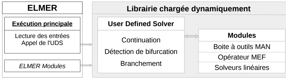
FIGURE 4.5 – Principe d'implémentation de techniques MAN dans ELMER.
