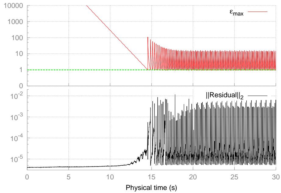
FIGURE 8.6 – Comportement de la méthode HPt utilisant la représentation polynomiale. La borne supérieure du domaine de validité [0, \varepsilon_{max}] des séries \{\mathbf{W}_{n+1}\} et la norme du résidu sont tracées en fonction du temps. Le maillage M1 est utilisé avec N = 30 , \eta = 10^{-6} .
