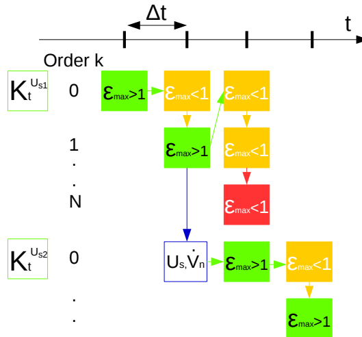
FIGURE 6.4 – Comportement de la méthode tHP utilisant un ordre de troncature adaptatif des séries MAN.
