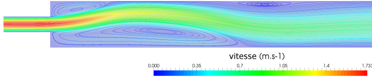
FIGURE 7.18 – Champ de vitesse pour un nombre de Reynolds Re=173 avec une nouvelle zone de recirculation.
