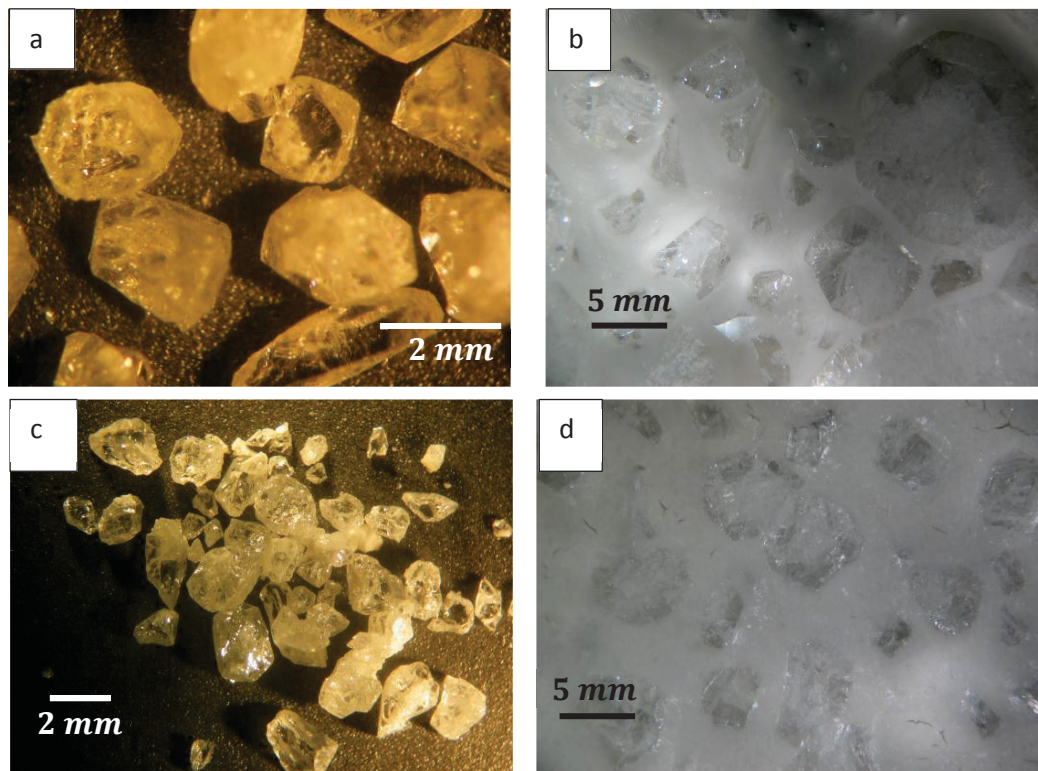
Figure 4.7 : Cristaux observés à la loupe binoculaire suite aux essais de refroidissement lent des mélanges (La_{0,6}Gd_{0,4})_{1+x}Sc_{3-x}(BO_3)_4 pour x = 0 (a), x = 0, 1 (b), x = 0, 2 (c) et x = 0, 3 (d).
