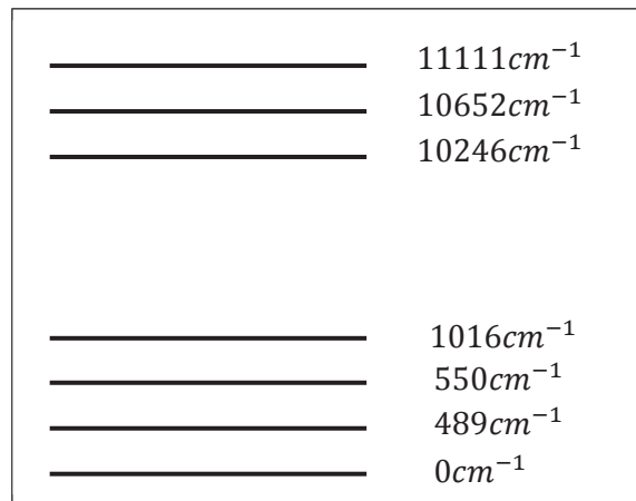
Figure 3.38 : Proposition des niveaux d'énergie de l'ion Yb^{3+} dans la matrice de YCOB [4].
