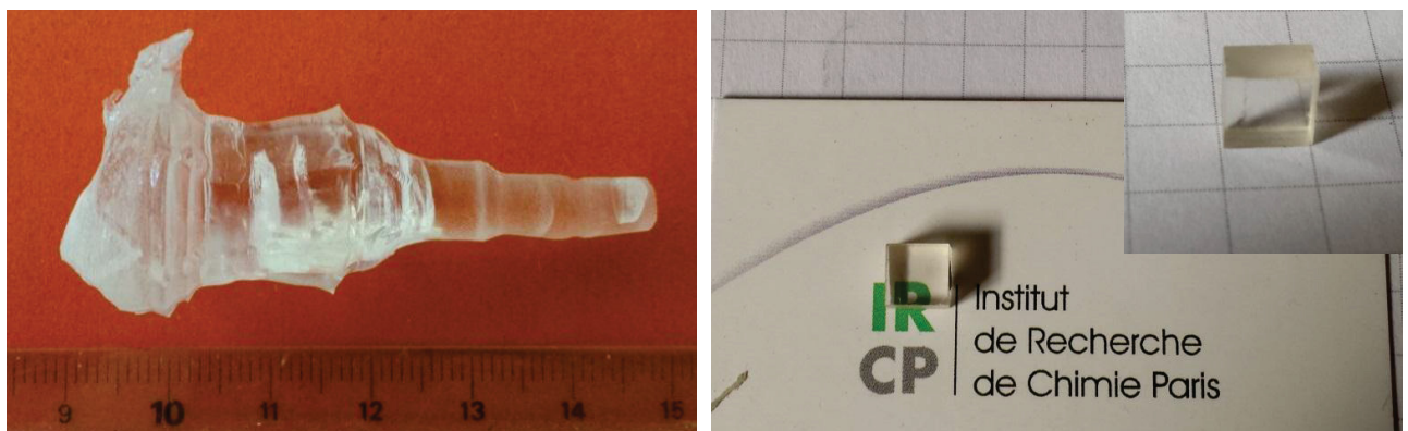
Figure 3.57 : Cristal de BCBF: Sr; Yb CZ 05 (gauche) et pièce orientée \sigma (axe \vec{c} perpendiculaire à la face polie) utilisée pour caractériser l'émission laser autour de 1 \mu\text{m} (droite).
