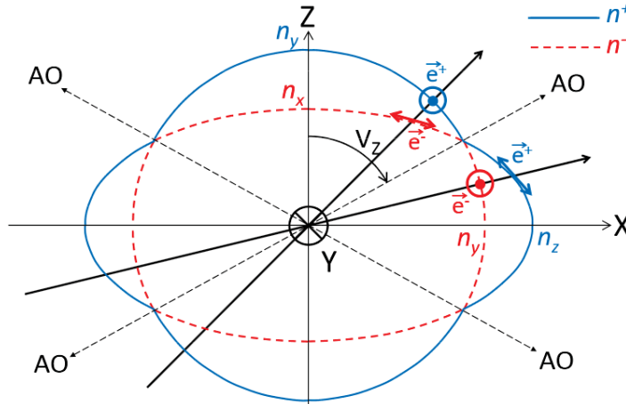
Figure 1.9 : Section dans le plan (X, Z) de la surface des indices d'un milieu biaxe. ⊙ et ↻ dénotent les directions des modes propres de polarisation e^+ et e^- relatifs aux différentes portions de nappes [26].
