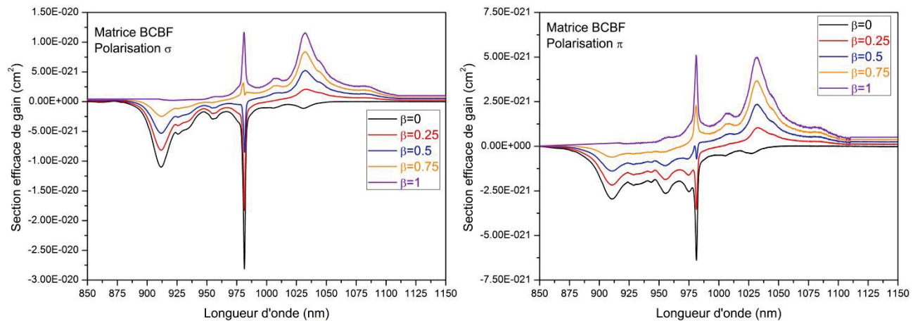
Figure 3.53 : Sections efficaces de gain en lumière polarisée \sigma (gauche) et \pi (droite) dans la matrice de BCBF ( 2\%Sr - 2\%Yb ) pour différents taux d'inversion de population \beta .
