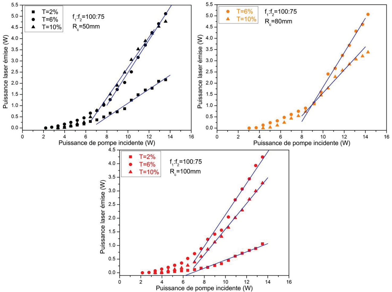
Figure 3.75 : Performances laser en régime continu de l'échantillon N°7 de YCOB: Yb(15\%at) pour différents miroirs de sortie.
