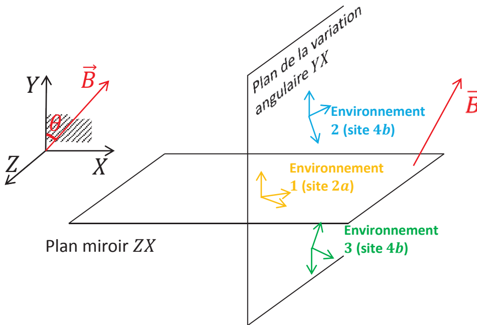
Figure 3.16 : Représentation schématique des différents environnements de l'ion ytterbium observés par RPE, et des axes propres de leurs tenseurs \hat{g} .
