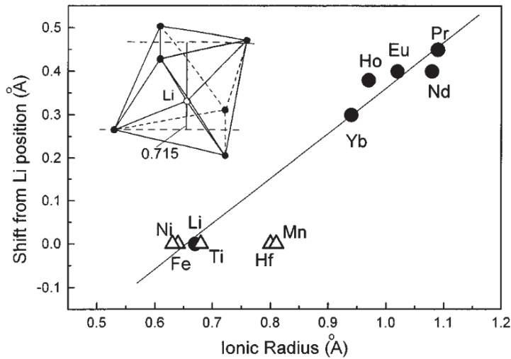
Figure 1.28 : Ecart en position entre l'ion dopant et l'ion lithium au sein du site cristallographique du lithium dans la matrice LiNbO_3 , en fonction du rayon ionique de l'ion dopant [77].
