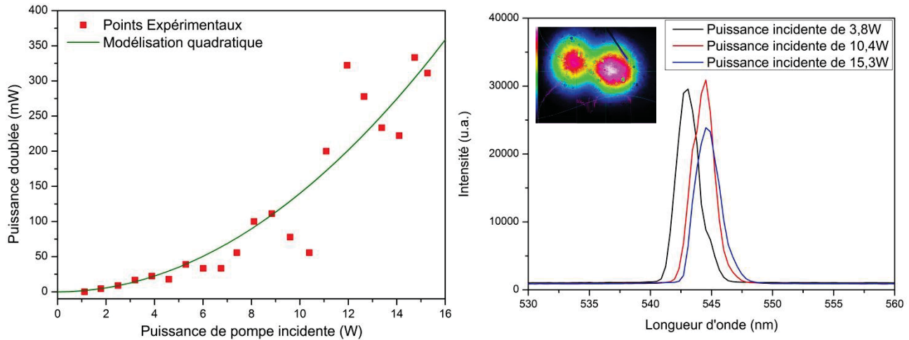
Figure 3.81 : À gauche, résultat de l'expérience d'auto-doublage de fréquence dans l'échantillon de YCOB:Yb(15%at) N°2 . À droite, spectre d'émission du faisceau laser doublé vert pour différentes valeurs de puissance incidente. En encadré, profil 2D typique du faisceau laser vert.
