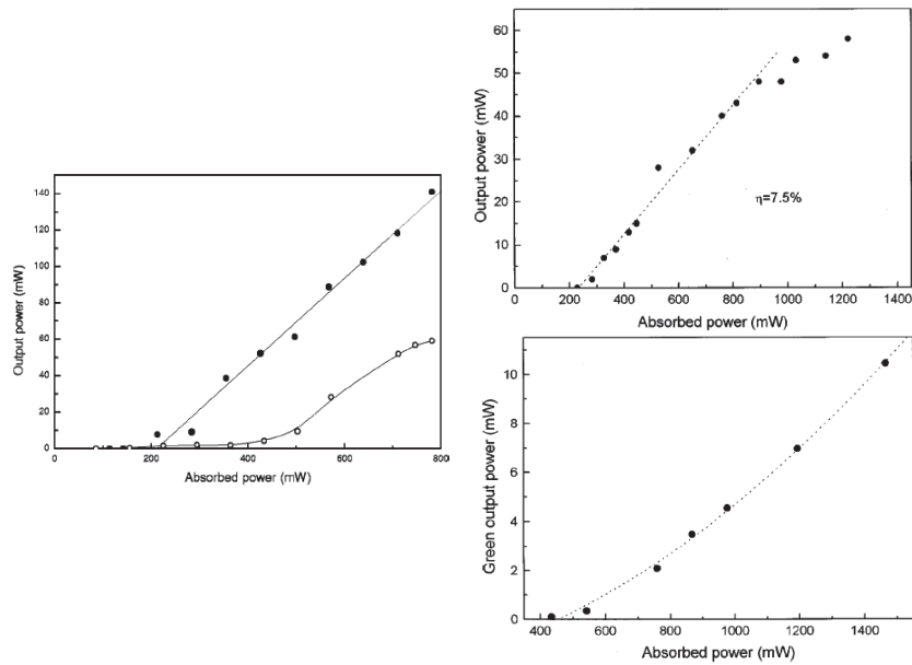
Figure 1.29 : Résultats d'auto-doublage dans le cas d'un cristal de LiNbO_3:MgO(6\%at):Yb^{3+}(1\%at) mono-domaine (gauche) [80] et périodiquement alterné (droite, bas) [79].
