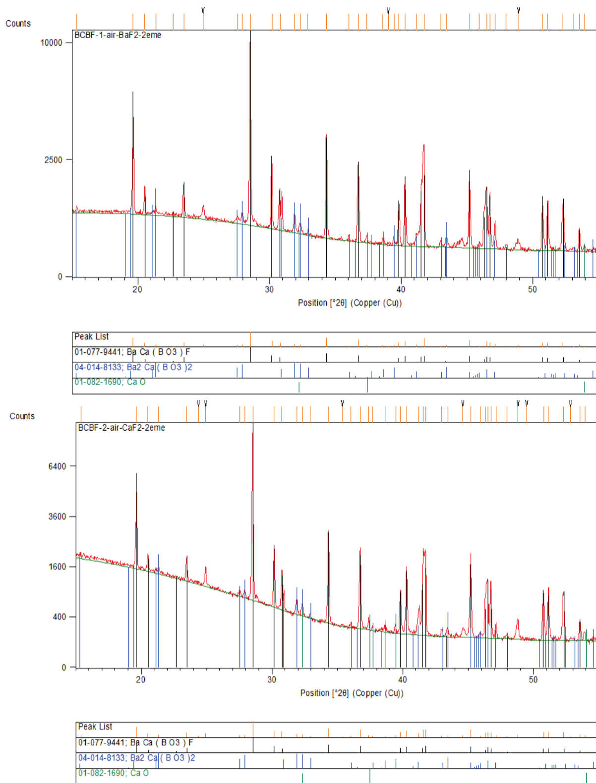
Figure 2.4 : Diffractogrammes des pastilles de BCBF synthétisées sous air, à partir de BaF_2 (haut) et CaF_2 (bas) avec leur identification.
