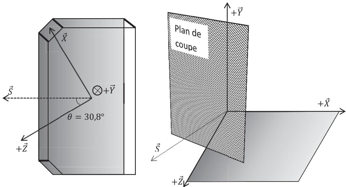
Figure 8.20 : À gauche, représentation schématique de l'échantillon de YCOB avant découpe, et position du repère diélectrique associé. À droite, schéma du repère diélectrique et du plan de coupe. \vec{S} correspond à la direction de propagation pour l'accord de phase de GSH en type I à 1064nm dans le plan principal ZX : (\theta_{ZX}; \varphi_{ZX}) = (30,8^\circ; 180^\circ) . L'échantillon est collé sur la face grisée.
