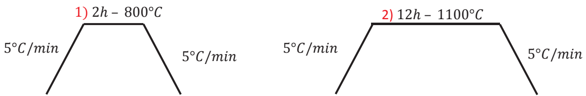
Figure 2.40 : Traitement thermique subit par les mélanges (La_yGd_{1-y})_{1+x}Sc_{3-x}(BO_3)_4 [22].
