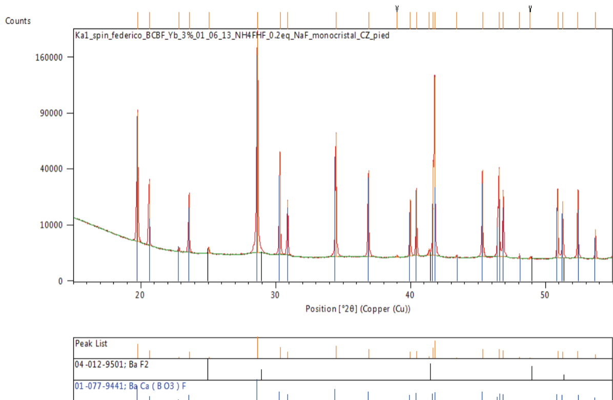
Figure 2.24 : Diffractogramme d'une partie du pied du cristal CZ02 broyé.
