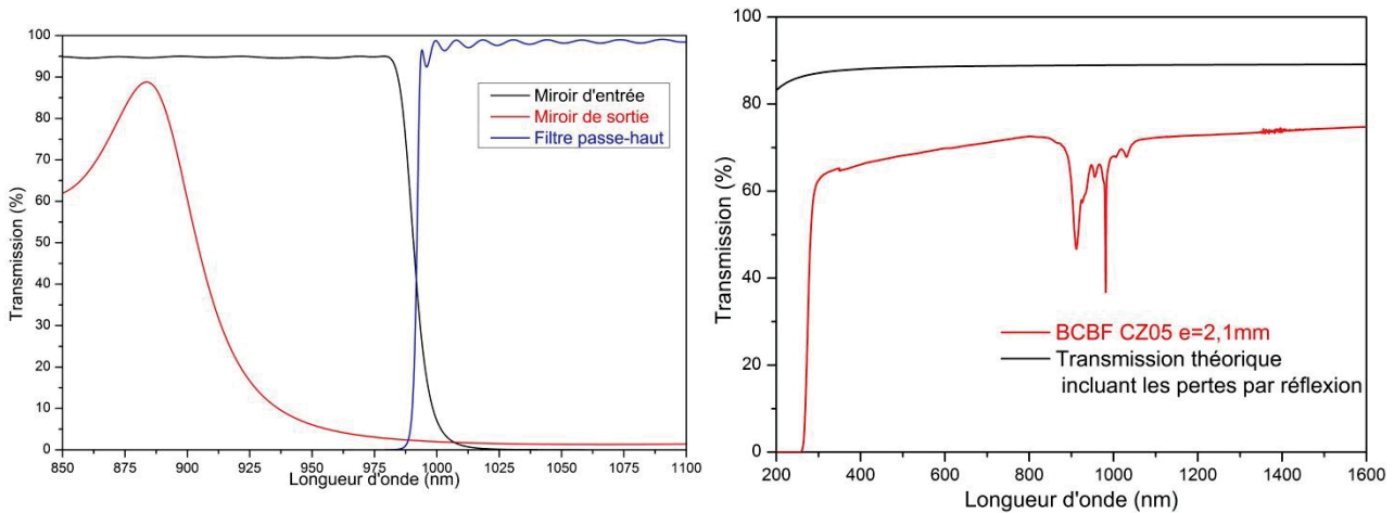
Figure 3.59 : À gauche, spectres de transmission des miroirs d'entrée (courbe noire) et de sortie (courbe rouge), et du filtre passe-haut (courbe bleue) utilisés pour caractériser l'émission laser autour de 1µm dans la matrice de BCBF(2%Sr – 2%Yb). À droite, spectre de transmission de l'échantillon de BCBF(2%Sr – 2%Yb) utilisé pour les tests laser (traits pleins) et transmission théorique du cristal en ne tenant compte que des pertes par réflexion aux interfaces air/cristal (traits pointillés).
