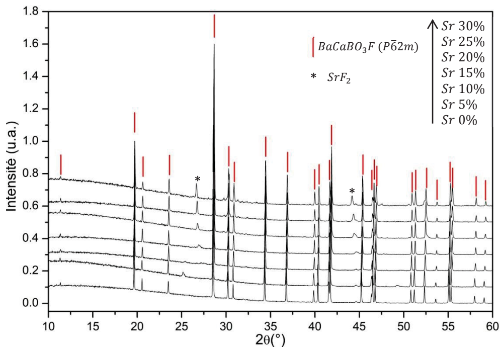
Figure 2.17 : Diffractogrammes comparés des pastilles de (\text{Ba}_{1-x}\text{Sr}_x)(\text{Ca}_{0,94}\text{Yb}_{0,03}\text{Na}_{0,03})\text{BO}_3\text{F} pour différents teneurs en strontium.
