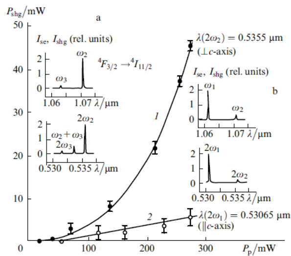
Figure 1.30 : Résultats d'auto-doublage colinéaire (a,1) et diffus (b,2) dans le cas d'un échantillon de Ba_2NaNb_5O_{15}:Nd^{3+} . Les spectres d'émission correspondants sont donnés dans les encadrés [93].
