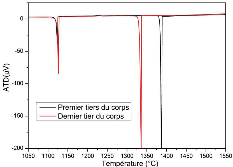
Figure 2.63 : Thermogrammes en refroidissement ( 10^{\circ}\text{C}/\text{min} ) d'un échantillon broyé issu du premier (traits pleins) et dernier (traits pointillés) tiers du corps du cristal CZ01. Le creuset ATD utilisé est en Pt .
