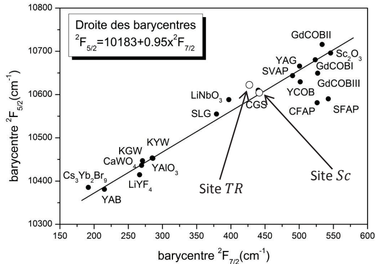
Figure 3.37 : Positionnement en énergie des barycentres des termes {}^2F_{7/2} et {}^2F_{5/2} de l'ion Yb^{3+} dans plusieurs matrices. Les cercles vides représentent les deux sites identifiés pour la matrice de LGSB .
