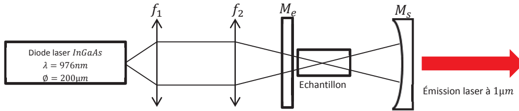
Figure 3.74 : Schéma expérimental du montage optique pour l'émission laser autour de 1\mu\text{m} dans les cristaux de YCOB: Yb(15\%at) taillés pour l'accord de phase à 1089\text{nm} .
