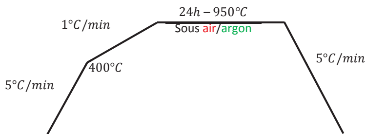
Figure 2.2 : Traitement thermique subi par les pastilles de \text{BCBF} .
