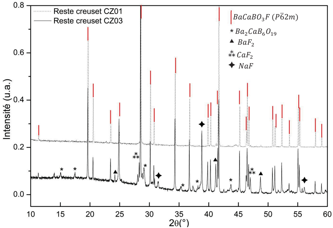
Figure 2.25 : Diffractogrammes comparés du bain restante dans le creuset après les croissances CZ01 (traits pointillés) et CZ03 (traits pleins). Les bâtonnets rouges représentent les pics caractéristiques de la phase de BCBF .
