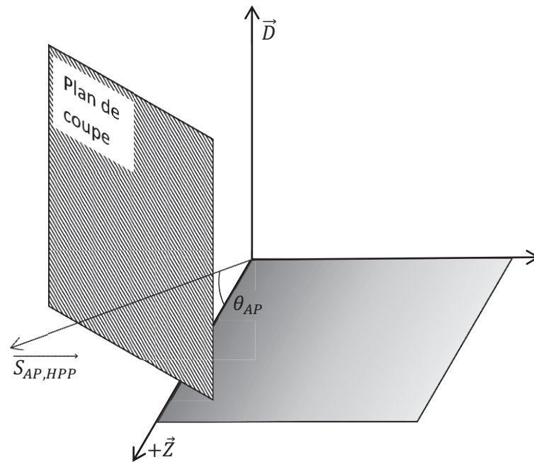
Figure 8.22 : Représentation du repère diélectrique et du plan de coupe associé à la troisième étape. La direction \overrightarrow{S_{AP,HPP}} correspond à la direction d'accord de phase hors des plans principaux permettant de maximiser le rendement de conversion pour la GSH en type I à 1064nm , définie par (\theta_{AP}; \varphi_{AP}) = (68^\circ; 143^\circ) . La direction \overrightarrow{D} est la même qu'en Figure 8.21. L'échantillon est collé sur la platine goniométrique par la face grisée.
