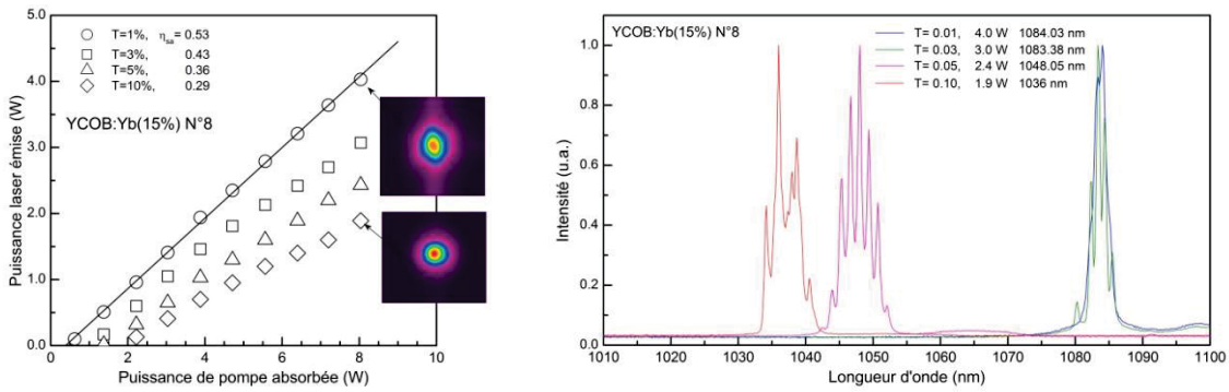
Figure 3.76 : Performances laser en régime continu de l'échantillon N°8 de YCOB:Yb(15%at) pour différentes transmission du miroir de sortie dans le cas d'une cavité plan (gauche) et spectres d'émission laser (droite). Résultats obtenus par Salamu au SSQEL. En encadré, profils 2D typiques obtenus pour le faisceau laser infra-rouge.
