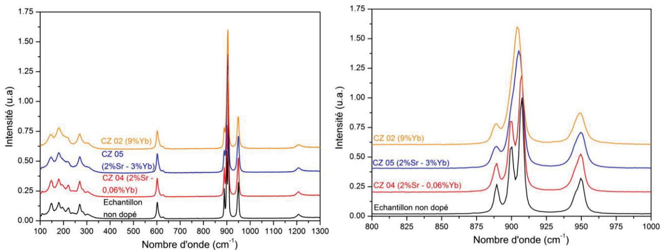
Figure 3.4 : Spectres Raman à température ambiante et en lumière non polarisée (gauche) pour quatre échantillons de BCBF monocristallin. Zoom dans la zone 800 - 1000 \text{ cm}^{-1} à droite.
