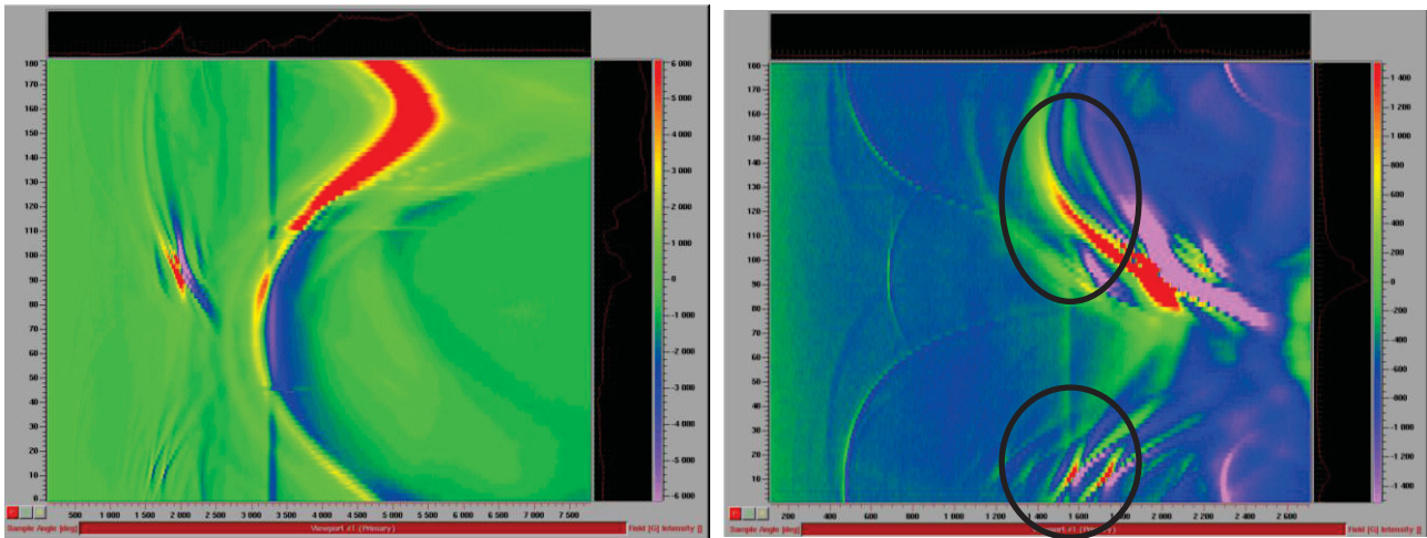
Figure 3.18 : Représentation 2D des spectres RPE enregistrés par variation angulaire de l'échantillon de YCOB: Yb(0,05\%) dans le plan ZX . L'axe des abscisses représente la valeur du champ B en Gauss et l'axe des ordonnées à gauche représente l'angle de rotation du porte échantillon dans la cavité RPE. L'intensité du signal RPE est alors reportée en intensité de couleur (échelle à droite).
