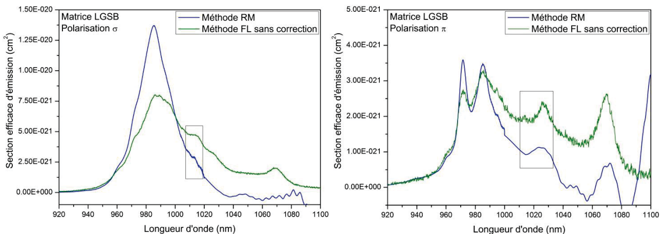
Figure 3.48 : Comparaison des sections efficaces d'émission calculées par les méthodes RM et FL pour l'état de polarisation \sigma (gauche) et \pi (droite) de l'échantillon LGSB:Yb (4,7%) CZ02 . Zone de raccorder potentielle entre les deux méthodes en encadré.
