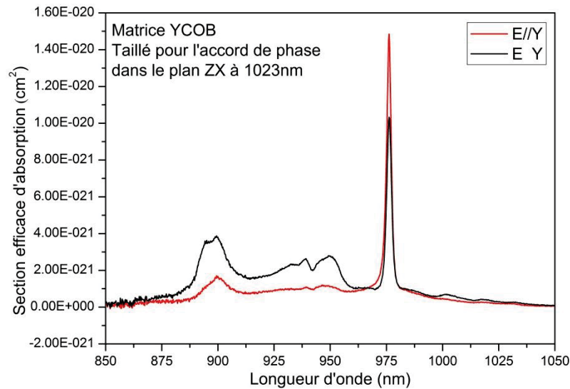
Figure 3.45 : Section efficace d'absorption pour les polarisations parallèle et perpendiculaire à l'axe diélectrique Y pour un échantillon de YCOB:Yb(13\%) taillé pour l'accord de phase dans le plan ZX à 1023nm [4].
