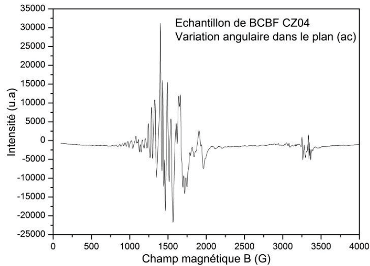
Figure 3.30 : Exemple de spectre RPE obtenu à 10K dans le plan ac pour un échantillon de CZ04 (2%Sr – 0,06%Yb).
