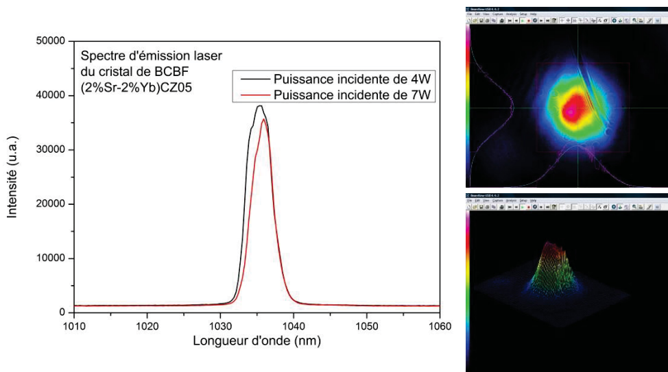
Figure 3.63 : Spectre d'émission laser du cristal de BCBF(2%Sr – 2%Yb) CZ05 pour deux valeurs de puissance incidente (gauche). Profils 2D et 3D du faisceau laser à 1034nm obtenu avec le logiciel Beamviewer (droite).
