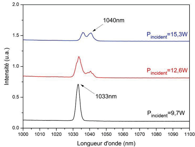
Figure 3.78 : Spectre d'émission laser pour différentes valeurs de puissance incidente au sein de l'échantillon de YCOB:Yb(15%at) N°7 avec le doublet achromatique f_1:f_2 = 100:150 .
