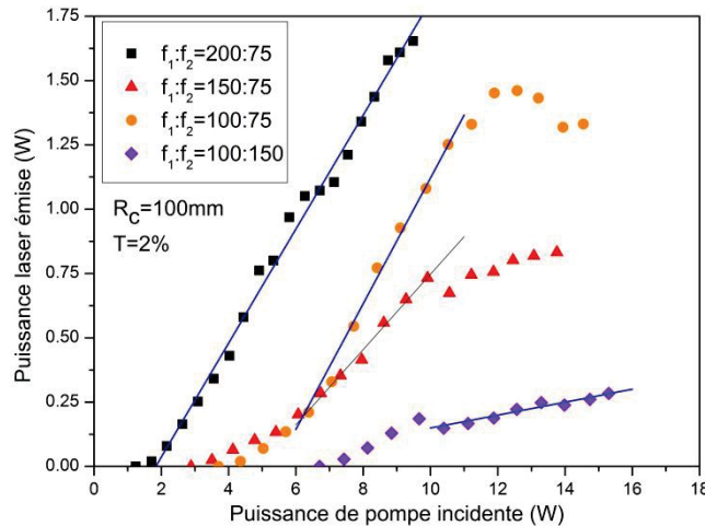
Figure 3.77 : Performances laser en régime continu de l'échantillon N°7 de YCOB:Yb(15%at) pour différents doublets achromatiques.
