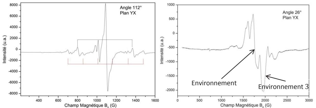
Figure 3.17 : Spectres RPE enregistrés à 10K dans le plan YX pour l'échantillon de YCOB: Yb(0,05\%) . En haut, signal relatif aux ions Yb^{3+} pour l'environnement 1 (site cristallographique 2a) pour un angle de rotation de 112^\circ . En bas, raies principales des ions Yb^{3+} pour les environnements 2 et 3 (site cristallographique 4b) pour un angle de rotation de 26^\circ .
