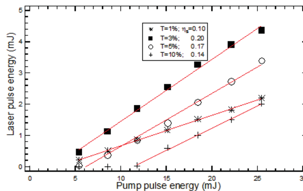
Figure 3.68 : Performances laser en régime quasi-continu dans l'échantillon N°1 de \text{LGSB:Yb} (orientation \sigma ) pour différentes valeurs de transmission du miroir de sortie. Résultats obtenus par Salamu au SSQEL.
