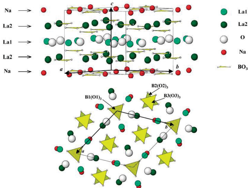
Figure 1.35 : Représentation structurale d'une maille de Na_3La_9O_3(BO_3)_8 (haut), et représentation des trois types de groupements borates présents dans la structure (bas). D'après [103].
