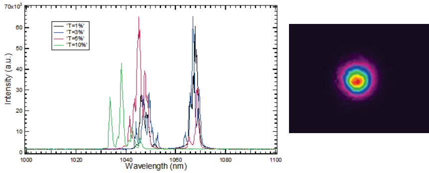
Figure 3.69 : Spectres d’émission du faisceau laser pour différents miroirs de sortie (gauche) et profil 2D du spot laser obtenu pour une transmission du miroir de sortie de 3%.
