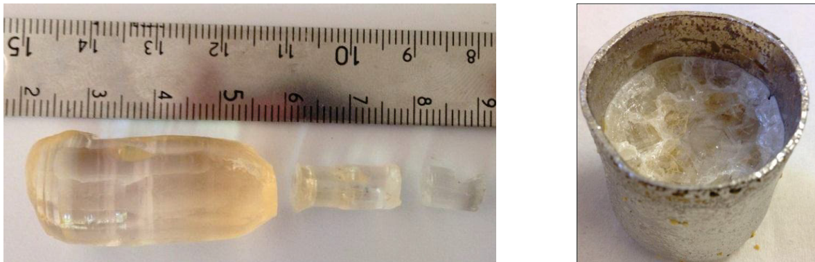
Figure 2.26 : Monocristal de composition souhaitée Ba_{0,9}Sr_{0,1}CaBO_3F (CZ04) obtenu par la méthode Czochralski (gauche) et creuset après croissance (droite).
