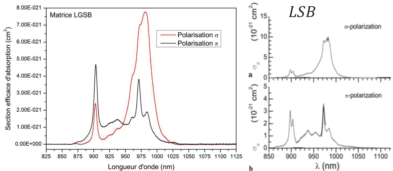
Figure 3.42 : Sections efficaces d'absorption pour les polarisations \sigma et \pi sur l'échantillon de LGSB:Yb (4,7%) CZ02 (gauche) et comparaison avec les données publiées pour un échantillon de LSB:Yb dans [30] (droite).
