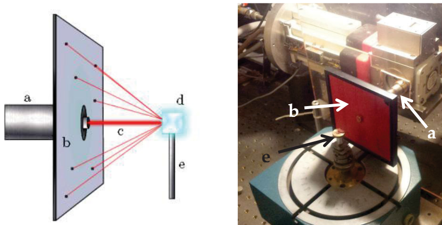
Figure 3.19 : Schéma (gauche) et photo (droite) du dispositif expérimental pour l'orientation des cristaux par la méthode de Laue [1].
