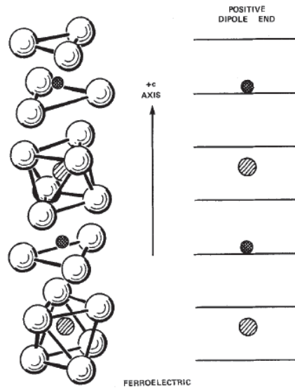
Figure 1.25 : Représentation structurale du LiNbO_3 pour une température inférieure à sa température de Curie. Les atomes de Li sont représentés en noirs, ceux de Nb sont hachurés et les lignes correspondent aux plans formés par les atomes blancs d'oxygène [68, 69].
