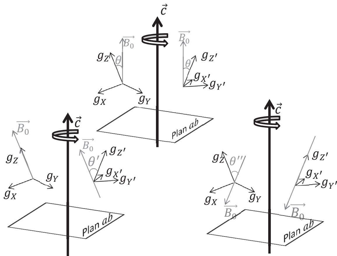
Figure 3.28 : Orientation relative des tenseurs \hat{g} pour deux ions Yb^{3+} obtenus par rotation autour du ternaire. Les schémas correspondent à différentes orientations du champ magnétique \vec{B}_0 pour une variation angulaire depuis l'axe \vec{c} vers le plan ab : \vec{B}_0 // \vec{c} (haut), \vec{B}_0 // \vec{g}_z (bas gauche) et \vec{B}_0 // \vec{g}_{z'} (bas droite).
