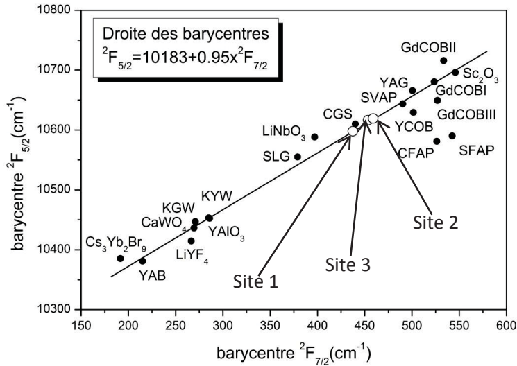
Figure 3.34 : Positionnement en énergie des barycentres des termes {}^2F_{7/2} et {}^2F_{5/2} de l'ion Yb^{3+} dans plusieurs matrices. Les cercles vides représentent les trois sites que nous avons identifiés pour la matrice de BCBF: Sr .
