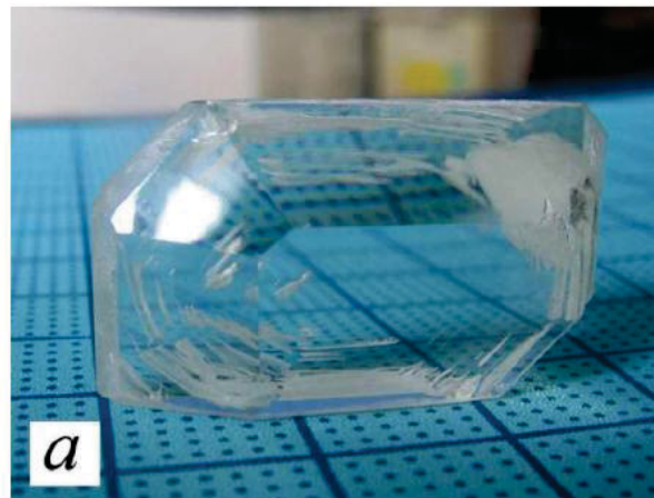
Figure 1.36 : Monocristal de Na_3La_9O_3(BO_3)_8 obtenu par croissance TSSG à partir d'un flux Na_2O - B_2O_3 - NaF avec un germe orienté [210]. D'après [106].
