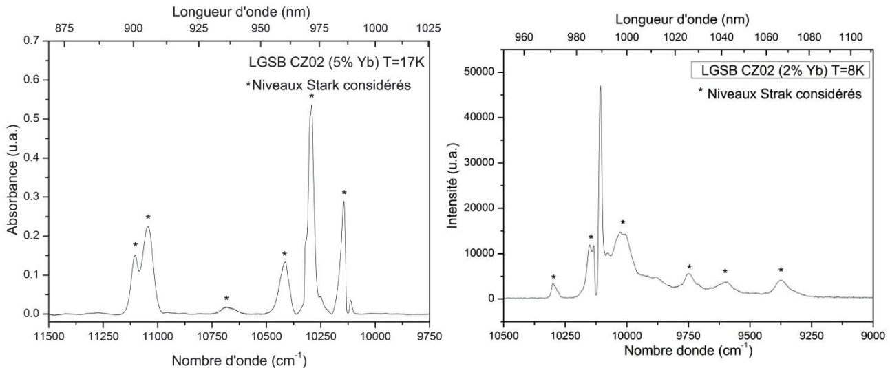
Figure 3.35 : Spectres d'absorption (gauche) et d'émission (droite) obtenus à basse température sur une tranche non orientée issue du cristal LGSB: Yb(5%at) CZ02 . Les abscisses sont indiquées par valeur d'énergie décroissante.
