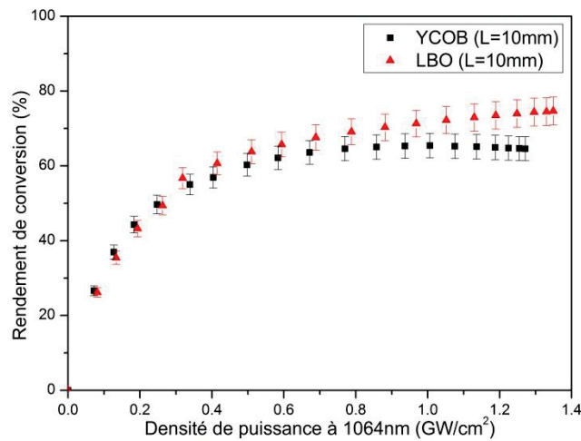
Figure 3.82 : Rendement de conversion pour la GSH de type I à 1064nm en fonction de la densité de puissance fondamentale à 1064nm dans des cristaux de YCOB et LBO de 10mm de long taillés pour l'accord de phase à 1064nm [47].
