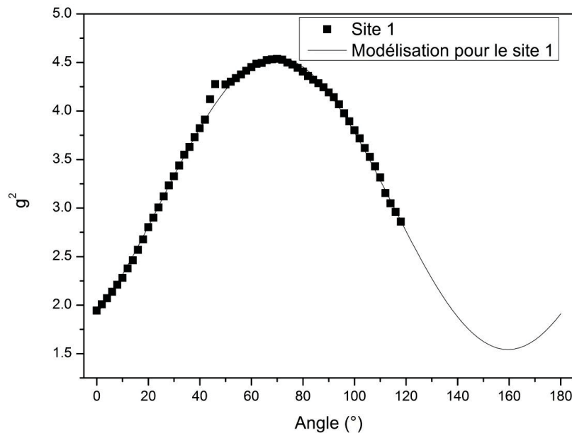
Figure 3.20 : Variation angulaire dans le plan ZX pour les ions Yb^{3+} dans le site principal (environnement 1, site cristallographique 2a).
