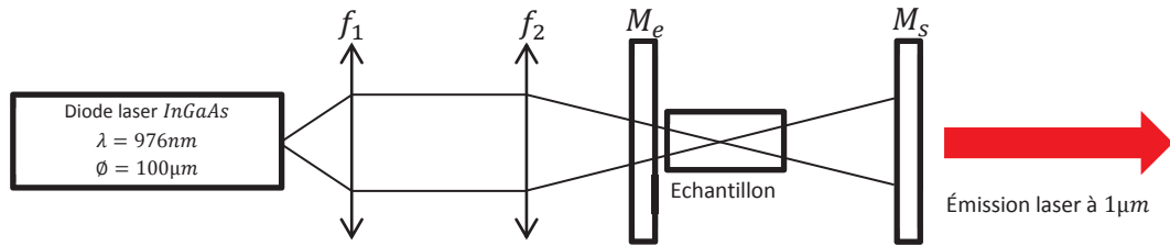
Figure 3.67 : Schéma expérimental du montage optique pour l'émission laser autour de 1\mu\text{m} dans la matrice de \text{LGSB:Yb}(13\%at) .
