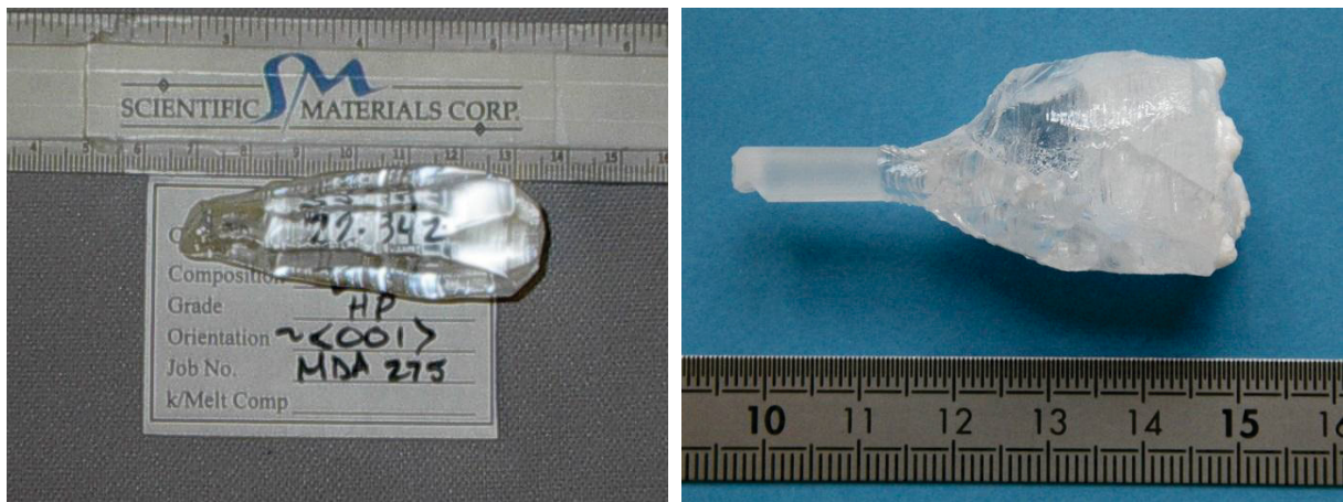
Figure 2.39 : Cristaux de composition (La_{0,625}Gd_{0,375})Sc_3(BO_3)_4 élaborés par la méthode Czochralski à partir d'un bain de composition (La_{0,625}Gd_{0,375})_{1,25}Sc_{2,75}(BO_3)_4 .
