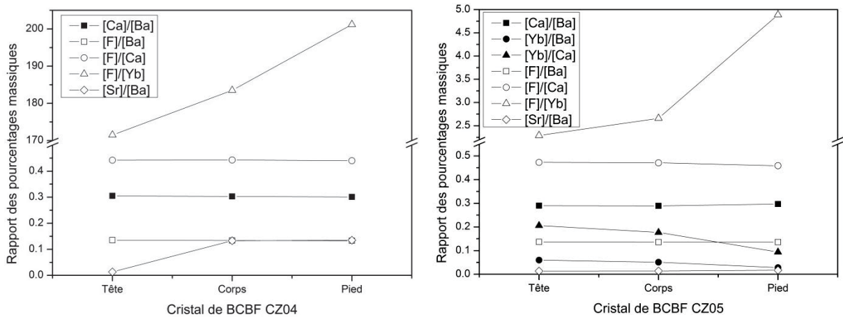
Figure 3.3 : Rapport de pourcentages massiques de différents cations et anions obtenus par ICP-AES pour différentes parties des cristaux de BCBF CZ04 et CZ05 .
