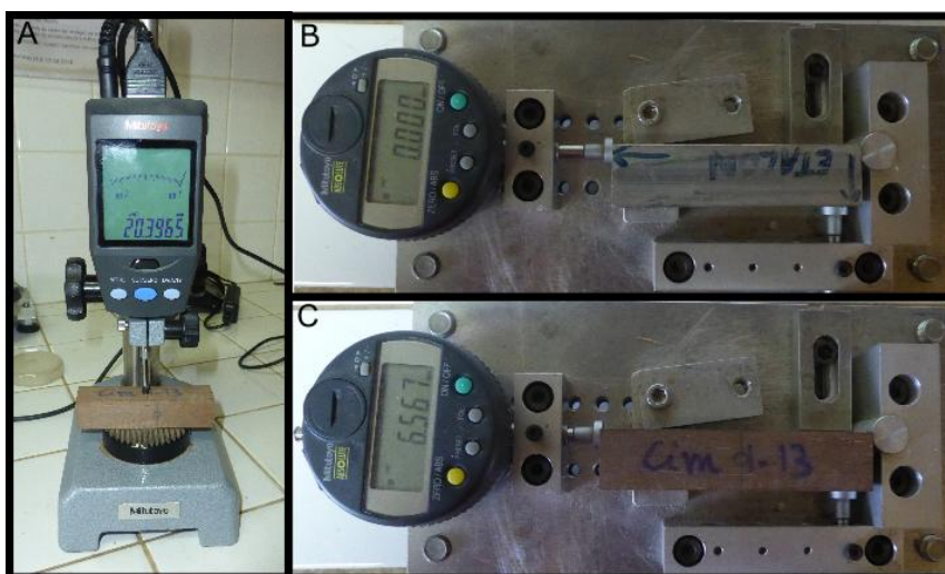
Figure 14 : Mesure des dimensions des éprouvettes de retrait.
