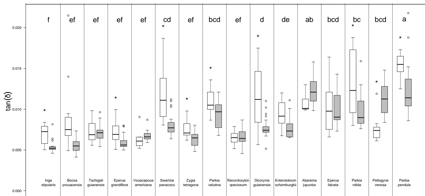
Variation interspécifique et intra-spécifique de l'amortissement ( \tan\delta ).
