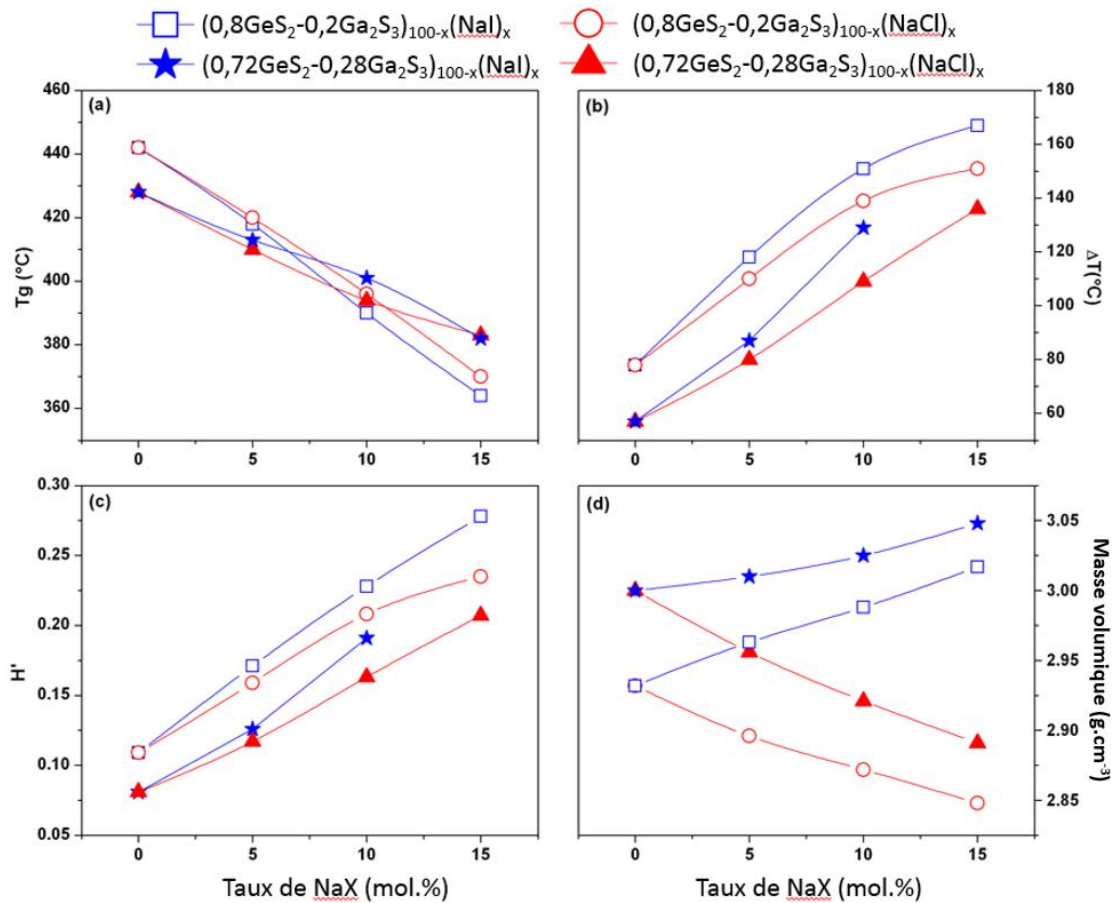
Figure 5.3 : Evolution des paramètres thermiques et de densité en fonction du taux x de NaX avec 0 \leq x \leq 15 et X = \text{Cl} ou \text{I} : (a) la transition vitreuse T_g , (b) la différence \Delta T entre T_g et T_x , (c) le critère de formation vitreuse H' et (d) la densité
