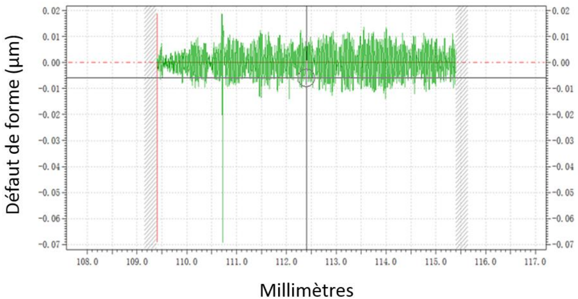
Figure 3.30: mesure de rugosité du verre 75\text{GeS}_2-15\text{Ga}_2\text{S}_3-10\text{CsCl}
