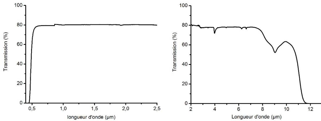
Figure 3.12 : Transmission du verre 75\text{GeS}_2-15\text{Ga}_2\text{S}_3-10\text{CsCl} (épaisseur : 4mm)
