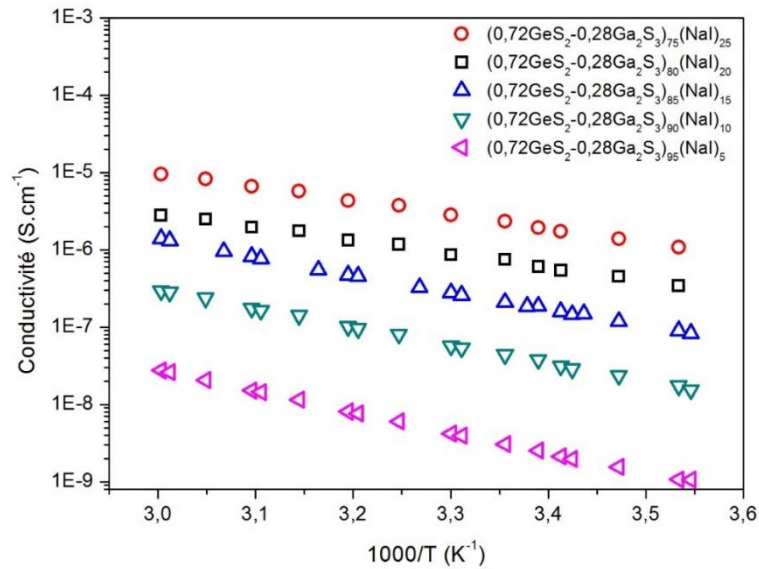
Figure 5.13 : Conductivité des verres de la série 1 correspondant à la ligne (0,72GeS_2-0,28Ga_2S_3)_{100-x}(NaI)_x avec 5 \leq x \leq 25
