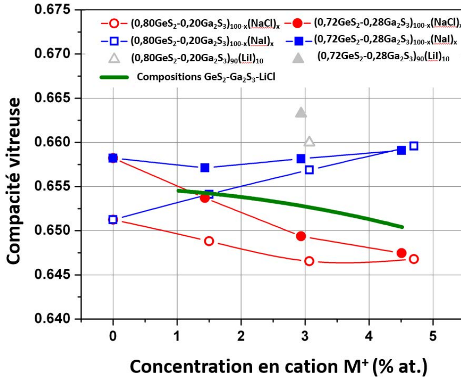
Figure 5.11 : Evolution de compacité vitreuse \rho en fonction de la concentration cationique M^+ des différents verres : (1) Pour (0,80\text{GeS}_2\text{-}0,20\text{Ga}_2\text{S}_3)_{100-x}(\text{MX})_x (symboles vides) avec \text{MX}=\text{NaCl} (rouge) ou \text{NaI} (bleu) ou \text{LiI} (gris clair). (2) (0,72\text{GeS}_2\text{-}0,28\text{Ga}_2\text{S}_3)_{90}(\text{MX})_{10} (symboles pleins) avec \text{MX}=\text{NaCl} (rouge) ou \text{NaI} (bleu) ou \text{LiI} (gris clair). De plus les compacités vitreuses de \text{LiCl-Ga}_2\text{S}_3\text{-GeS}_2 (ligne verte) sont montrées pour comparaison.
