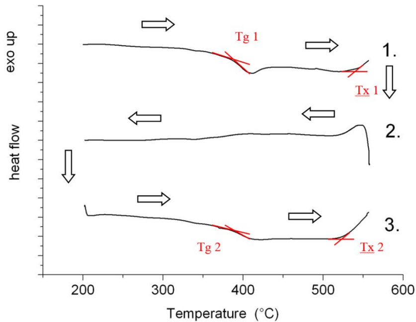
Figure 3.6 : Analyse par DSC du verre 65\text{GeS}_2-20\text{Ga}_2\text{S}_3-15\text{CsCl}
