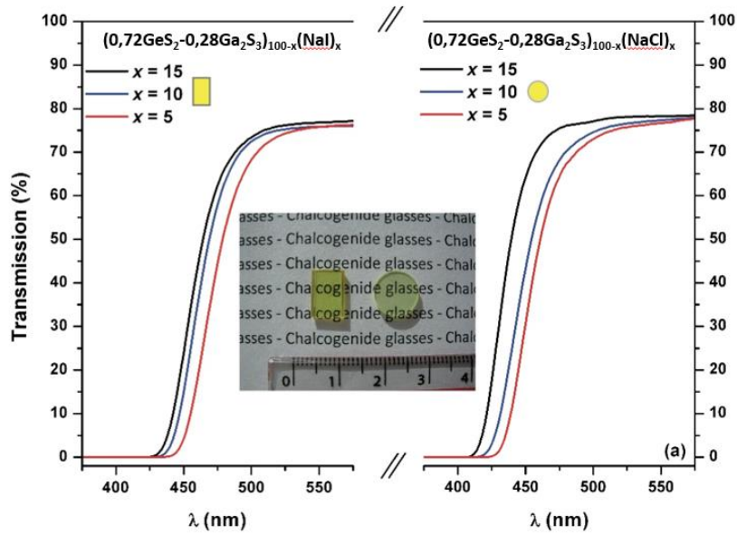
Figure 5.4 : Evolution de la transmission dans le domaine visible pour les verres de composition (0,72\text{GeS}_2\text{-}0,28\text{Ga}_2\text{S}_3)_{100-x}(\text{NaX})_x avec X = \text{Cl} ou \text{I} et 5 \leq x \leq 15 . La photographie des échantillons est présentée au milieu du graphique avec un parallélépipède et une pastille pour les compositions (0,72\text{GeS}_2\text{-}0,28\text{Ga}_2\text{S}_3)_{90}(\text{NaI})_{10} et (0,72\text{GeS}_2\text{-}0,28\text{Ga}_2\text{S}_3)_{90}(\text{NaCl})_{10} respectivement.
