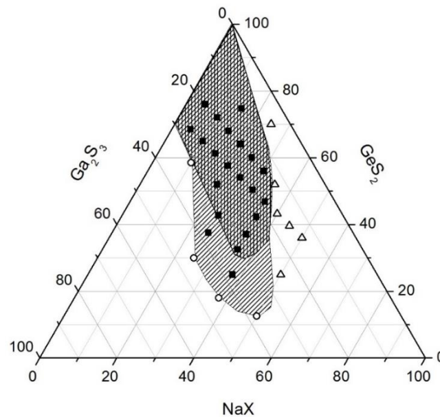
Figure 5.2 : Système vitreux GeS_2-Ga_2S_3-NaX avec X=Cl (rayures verticales) : domaine issu de travaux de Tver'Yanovich [23] et al. ou X = I (rayures horizontales) : point noir (échantillon vitreux), point vide (échantillon partiellement cristallisés) et triangle vide (échantillon totalement cristallisé)
