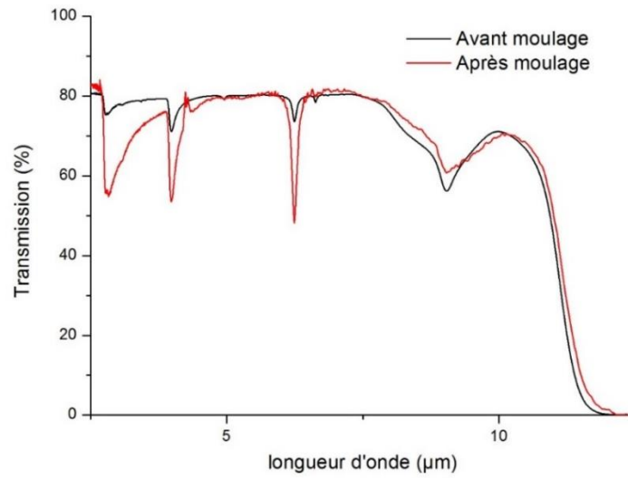
Figure 3.29: Transmission de 20\text{Ga}_2\text{S}_3-65\text{GeS}_2-15\text{CsCl} avant et après moulage
