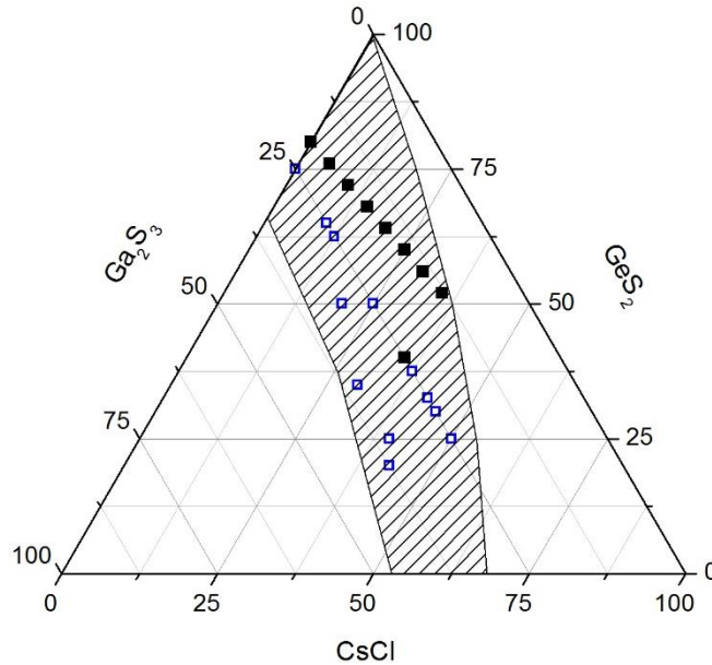
Figure 2.17 : Compositions étudiées dans le système GeS_2-Ga_2S_3-CsCl (carré plein : compositions synthétisées et carré vide : compositions issues de la littérature)
