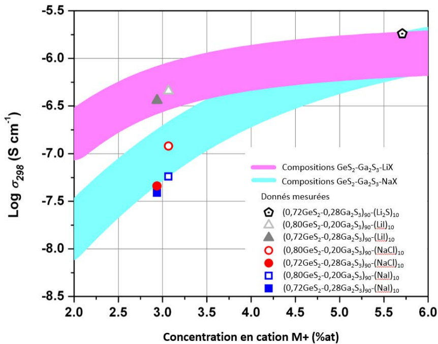
Figure 5.10 : Conductivités à température ambiante \sigma_{298} pour les différents verres : (1) (0,80GeS_2-0,20Ga_2S_3)_{90}(MX)_{10} (symboles vides) avec MX=NaI (bleu) ou NaCl (rouge) ou LiI (gris clair), (2) (0,72GeS_2-0,28Ga_2S_3)_{90}(MX)_{10} (symboles pleins) avec MX=NaI (bleu) ou NaCl (rouge) ou LiI (gris clair) et (3) (0,72GeS_2-0,28Ga_2S_3)_{90}(Li_2S)_{10} (symboles noirs). Les données reportées [23] correspondent aux conductivités moyennes à 298K pour les systèmes NaCl-Ga_2S_3-GeS_2 (ligne bleue) et LiCl-Ga_2S_3-GeS_2 (ligne violette).
