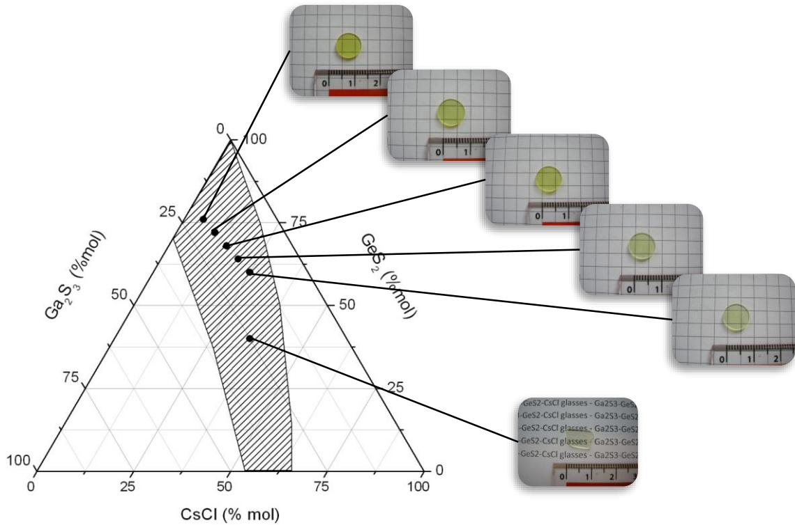
Figure 2.18: Système ternaire GeS_2 - Ga_2S_3 - CsCl
