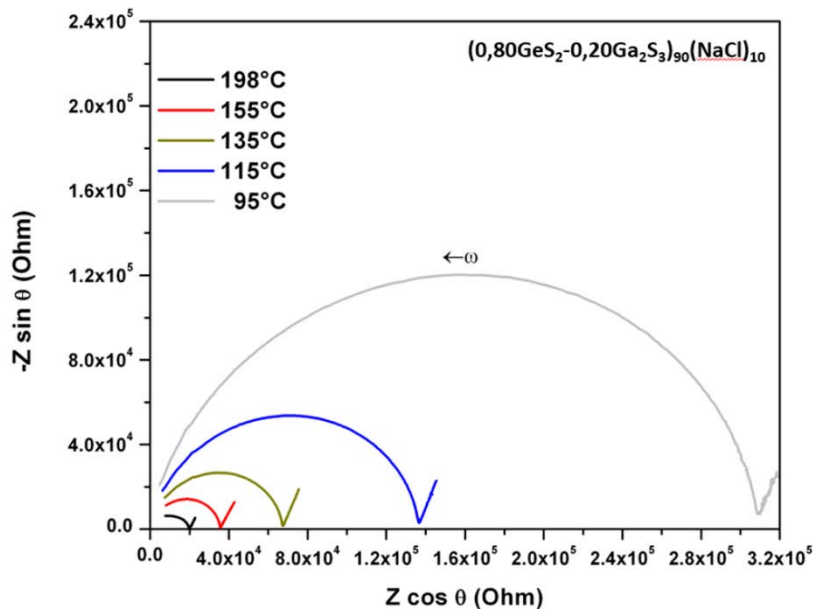
Figure 5.7 : Evolution des diagrammes de Nyquist pour la composition (0,80GeS_2-0,20Ga_2S_3)_{90}(NaCl)_{10} à différentes températures
