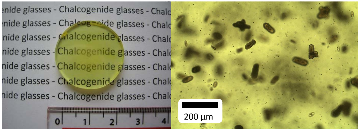
Figure 3.2 : Exemple de cristallisation à cœur pour la composition 63\text{GeS}_2-22\text{Ga}_2\text{S}_3-15\text{CsCl}
