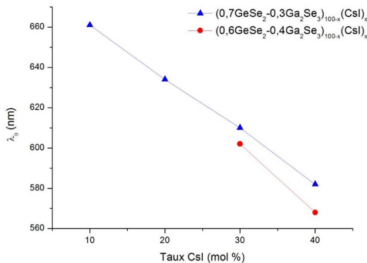
Figure 2.16 : Evolution de \lambda_0 en fonction du taux de CsI (les lignes ne représentent aucune données scientifiques)
