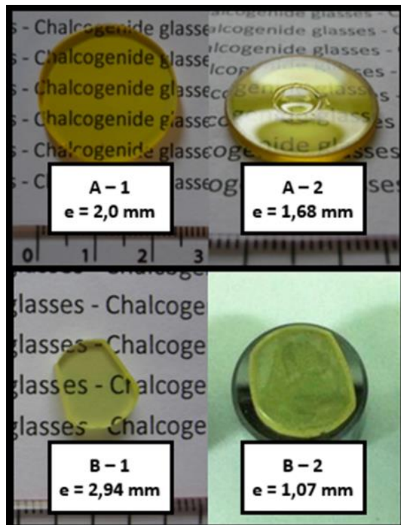
Figure 3.27 : Mise en forme de 75\text{GeS}_2-15\text{Ga}_2\text{S}_3-10\text{CsCl} (forme asphérique : A-1 et A-2) et 65\text{GeS}_2-20\text{Ga}_2\text{S}_3-15\text{CsCl} (forme plane : B-1 et B-2)
