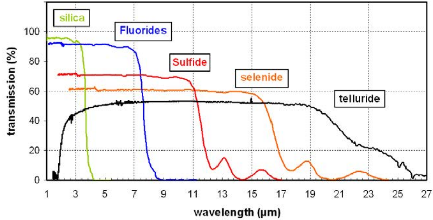
Figure 2.3 : Evolution de la coupure multi-phonon en fonction des familles de verres
