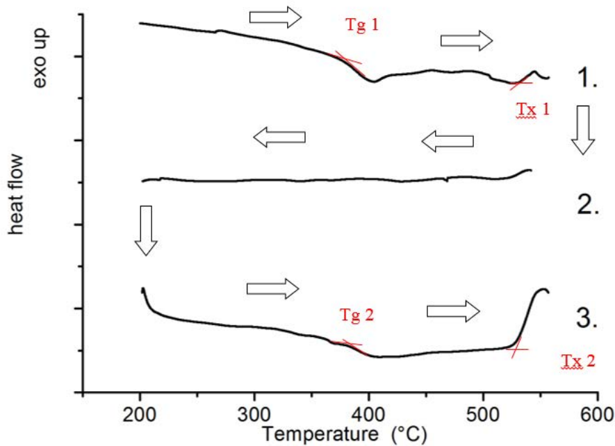
Figure 3.3 : Analyse par DSC du verre 75\text{GeS}_2-15\text{Ga}_2\text{S}_3-10\text{CsCl}
