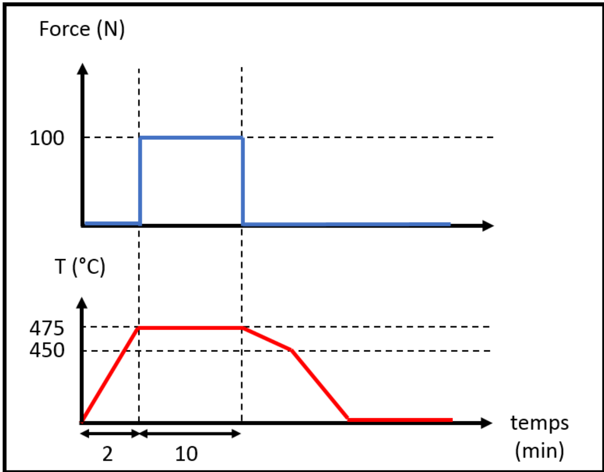
Figure 3.28 : Détails des forces et températures appliquées pour le moulage du verre 65\text{ GeS}_2-20\text{ Ga}_2\text{S}_3-15\text{ CsCl} pour une forme plane
