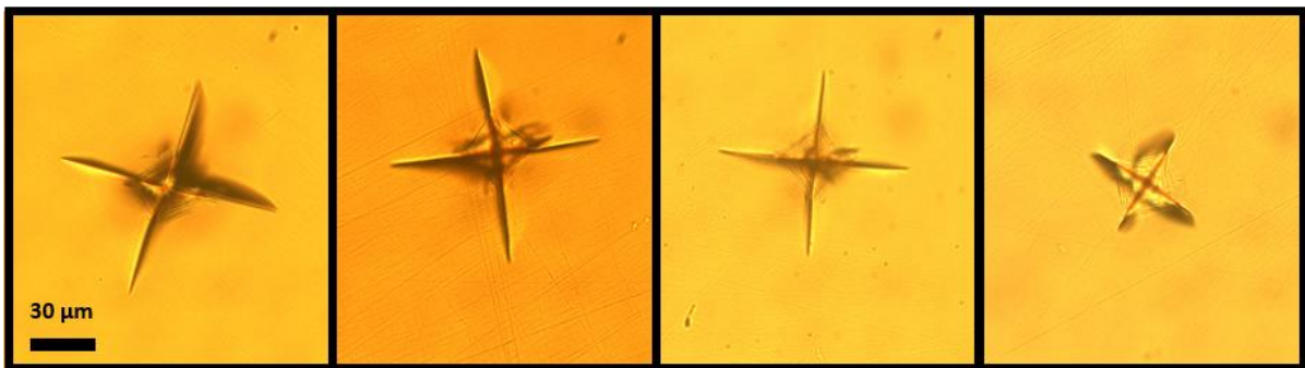
Figure 3.11 : Duretés Vickers des verres (compositions (0,8\text{GeS}_2-0,2\text{Ga}_2\text{S}_3)_{100-x}\text{CsCl}_x avec de gauche à droite x=0, 5, 10 et 15 )
