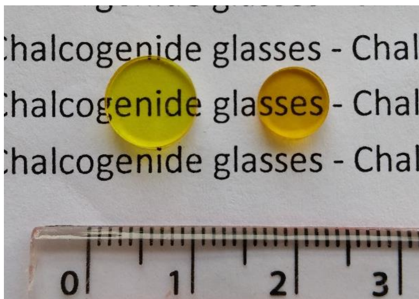
Figure 4.4 : Pastille de 75 GeS 2 - 15 Ga 2 S 3 - 10 CsCl (à gauche, de couleur jaune) et 75 GeS 2 - 15 In 2 S 3 - 10 CsCl (à droite de couleur orange)
