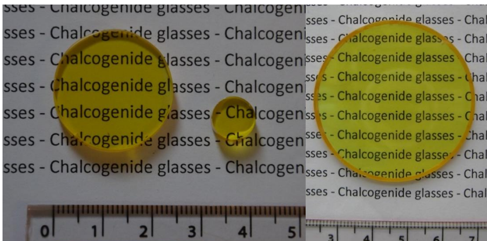
Figure 3.7 : Verres de compositions 75\text{GeS}_2-15\text{Ga}_2\text{S}_3-10\text{CsCl} (image de gauche en diamètres 10 et 25mm) et 65\text{GeS}_2-20\text{Ga}_2\text{S}_3-15\text{CsCl} (image de droite en diamètres 50mm)
