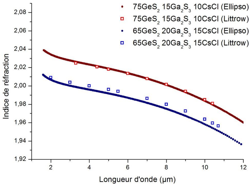
Figure 3.17 : Comparaison des mesures par ellipsométrie et Littrow
