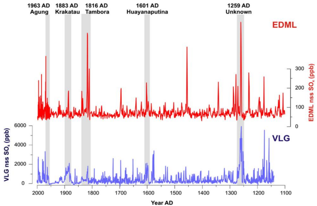
Figure 18. Enregistrements de SO 4 nss (non seasulphate) à EPICA Dronning Maud Land (EDML) et à Victoria Lower Glacier (VLG) pour les derniers 900 ans, indiquant les éruptions volcaniques sur cette période. Les aires en gris soulignent les éruptions volcaniques identifiées aux deux sites, EDML et VLG. D'après Bertler et al., 2011.
