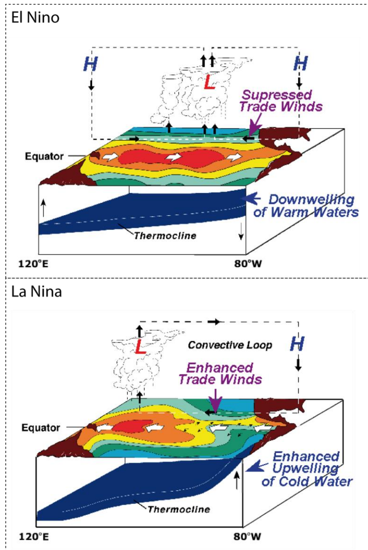
Figure 13. Vue schématique des conditions El Niño/La Niña dans le Pacifique, et des répercussions atmosphériques et océaniques dans la région du Pacifique ( http://fr.wikipedia.org/wiki/El_Niño ).
