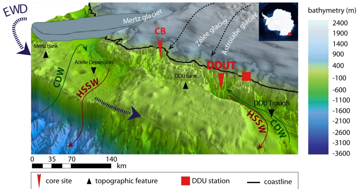
Figure 30. Vue topographique 3D de la TAGV, indiquant les structures topographiques remarquables (glaciers, hauts fonds etc.), les principales masses d'eau et les principaux courants océaniques (ex: East Wind Drift - EWD), ainsi que la localisation des sites de carottage. Données topographiques issues de Beaman et al. (2011).
