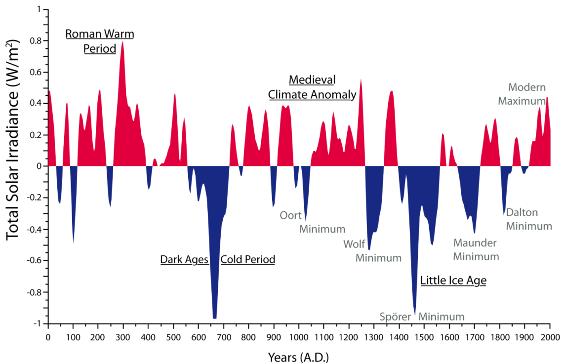
Figure 17. Variation de l'activité solaire reconstruite d'après les enregistrements de ^{10}\text{Be} mesurés dans la glace polaire (Steinhilber et al., 2009), indiquant les anomalies positive (aires rouges) et négatives (aires bleues), les pics reconnaissables (en gris) de l'activité solaire du dernier millénaire ainsi que les grandes phases climatiques connues de l'Hémisphère Nord (surlignées).
