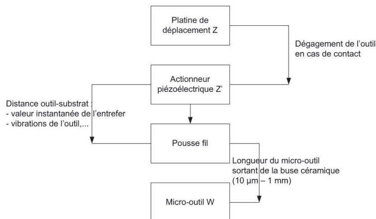
Figure 53 – Actionnement triple du micro-outil.
