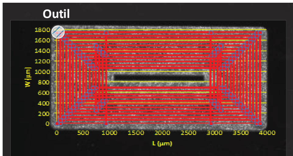
Figure 132 – Usinage d'un insert avec R=75\% : parcours d'outil d'une couche en rouge superposé au résultat d'usinage (photographie).
