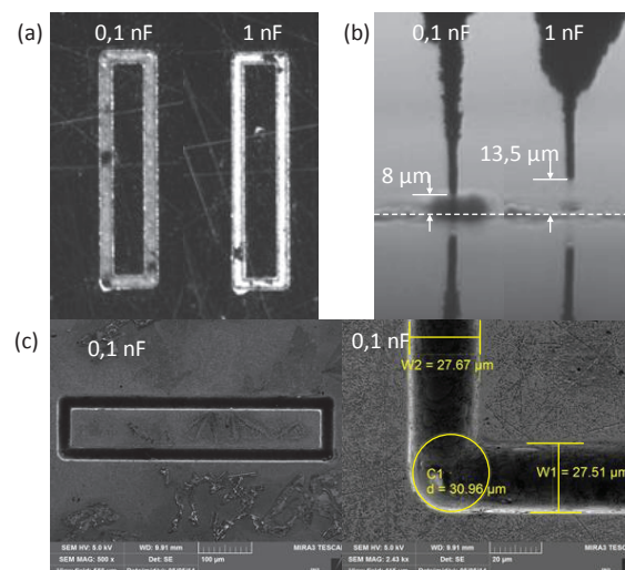
Figure 167 – (a) Images optiques des canaux usinés à H_C = 50 \mu\text{m} avec : (b) longueur d'usure du micro-outil ; (c) Images MEB du canal usiné avec C_C = 0,1 \text{ nF} .
