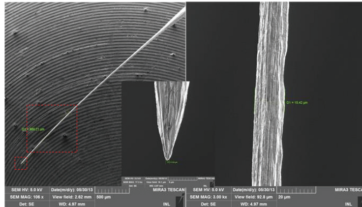
Figure 98 – Défaut de surface d'un micro-outil de 15 µm de diamètre vu au MEB.
