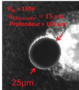
Figure 181 – Trous profonds. ( \Phi_{\text{Electrode}} = 5 \mu\text{m} sur la pointe)
