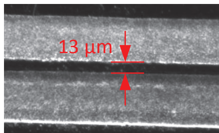
Figure 182 – Mur fin de 13 \mu\text{m} . ( \Phi_{\text{Electrode}} = 14 \mu\text{m} ; C = 22 \text{ nF} ; entrefer initial H = 10 \mu\text{m} ; enfoncement 10 \mu\text{m} )
