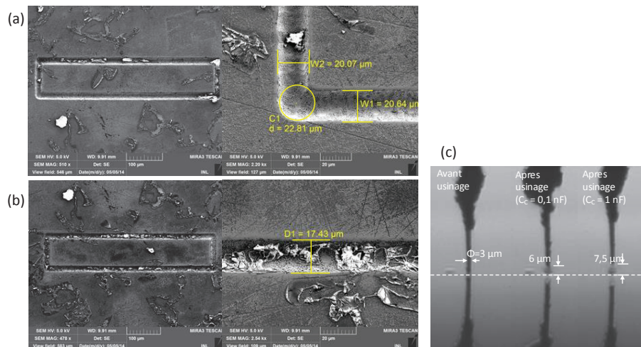
Figure 166 – Images des canaux usinés à H_C = 20 \mu\text{m} avec : (a) C_C = 0,1 \text{ nF} ; (b) C_C = 1 \text{ nF} ; (c) longueurs d'usure du micro-outil.
