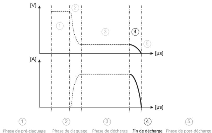
Figure 12 – Phase de fin de décharge d'après [27].
