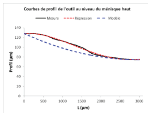
Figure 174 – Comparaison entre les profils décrits par la mesure au profilomètre laser, la courbe de régression et le modèle mathématique décrit par Lim et al. [180].
