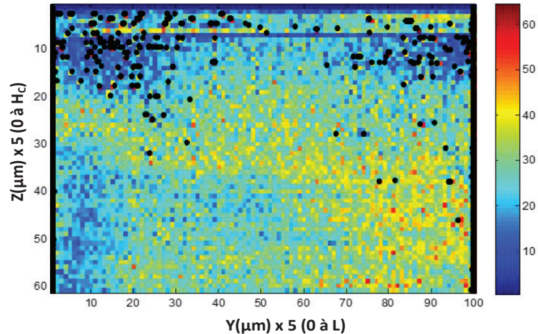
Figure 117 – Superposition de la cartographie des contacts et de la représentation en couleur des décharges ( H_c = 300 \mu\text{m} ). Echelle en X et Y : 5 \mu\text{m} / unité.
