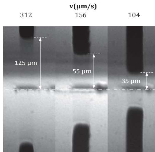
Figure 123 – Influence de la vitesse sur l'usure de l'outil.
