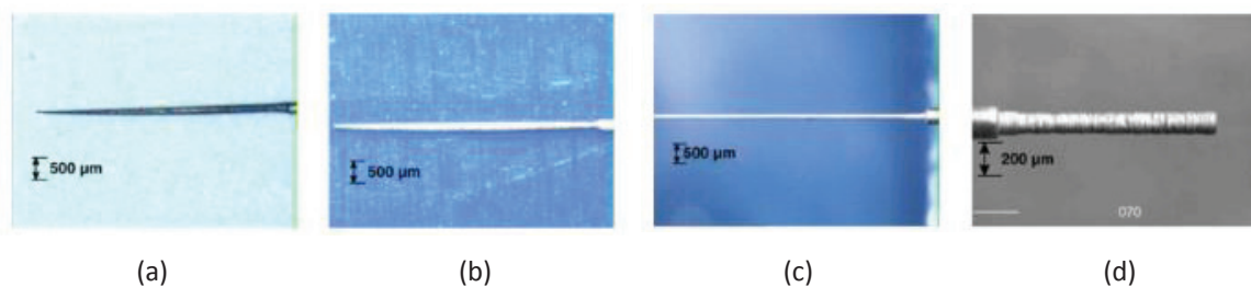
Figure 70 – Micro-outils obtenus par électroérosion par les méthodes suivantes: (a) et (b) bloc stationnaire; (c) disque en rotation ; (d) érosion à fil [141][142].
