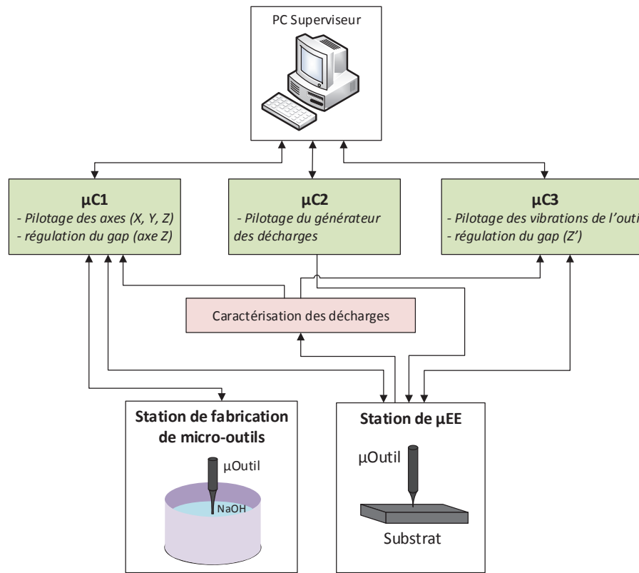
Figure 48 – Solution retenue pour la commande électronique de la machine de μEE de 2 ème génération.
