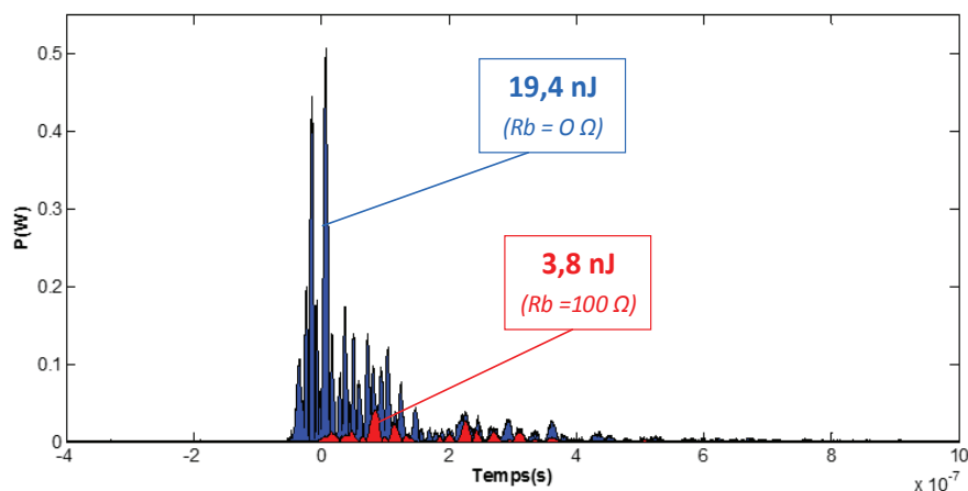
Figure 161 – Puissance véhiculée par les signaux de type B pour R_b 0 et 100 \Omega .
