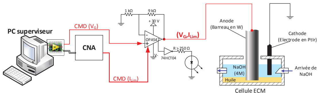
Figure 83 – Principe de la carte de génération des impulsions de gravure après modification.
