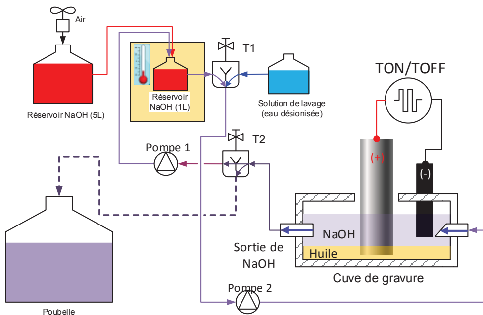
Figure 81 – Cellule de gravure électrochimique avec le dispositif fluidique permettant de renouveler la solution d'électrolyte.
