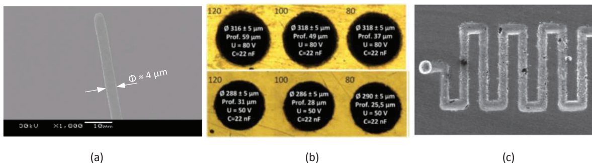
Figure 46 – Essais réalisés avec la machine de 1 ère génération d'après [13]. (a) Micro-outil en tungstène ( \phi = 4 \mu\text{m} ; F_r = 20 ). (b) Série de trous usinés dans l'acier inoxydable. (c) Canal microfluidique ( W = 40 \mu\text{m} ; H = 15 \mu\text{m} ).
