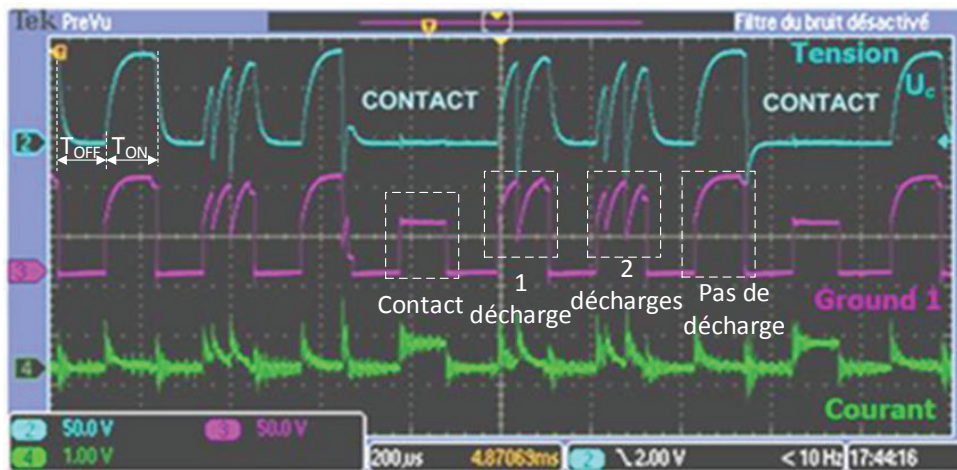
Figure 45 – Capture d'écran par oscilloscope des décharges en cours d'usinage. En bleu : d.d.p. aux bornes de C_C . Violet : d.d.p. entre le point POL et le point de référence GND2. Vert : courant qui traverse l'outil ( 1V=1A ). R_b = 0 \Omega
