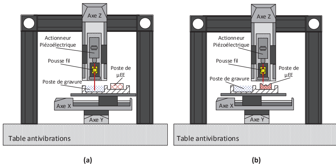
Figure 50 – Principales fonctions de la machine de \mu EE: (a) Fabrication de micro-outils par gravure électrochimique; (b) Fraisage sur substrat en acier inoxydable par \mu EE.
