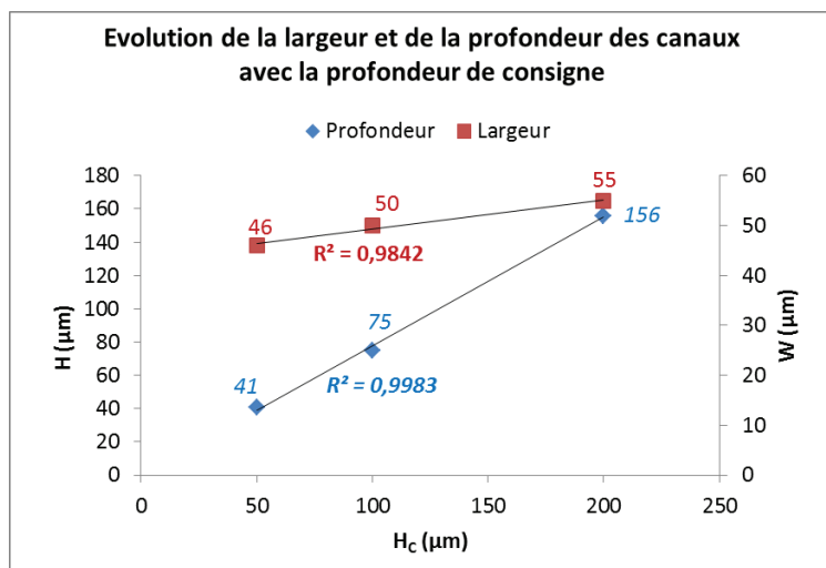
Figure 141 – Evolution de la largeur et de la profondeur des canaux usinés en fonction de la profondeur de consigne H_c (usinage avec régulation de l'entrefer).
