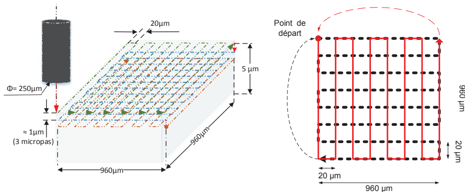
Figure 155 – Illustration du parcours d'outil pour l'usinage de la cavité carrée.
