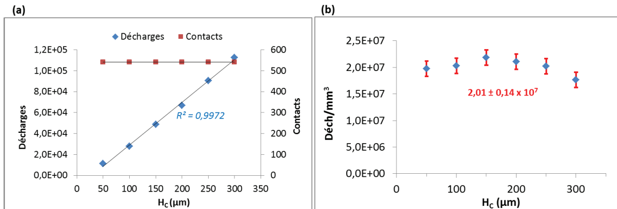
Figure 113 – Influence de la profondeur de consigne sur : (a) le nombre total de décharges électriques et de contacts mécaniques détectés ; (b) le nombre de décharges par \text{mm}^3 de matière usinée.
