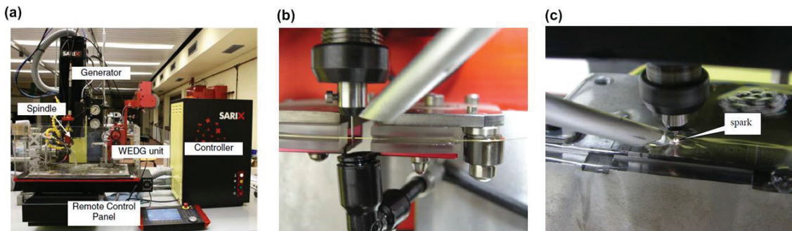
Figure 29 – Machine de fraisage par \mu\text{EE} SX-100. (a) Vue d'ensemble d'après [101]. (b) Poste de fabrication des outils par WEDG d'après [100]. (c) Poste de fraisage par \mu\text{EE} d'après [100].
