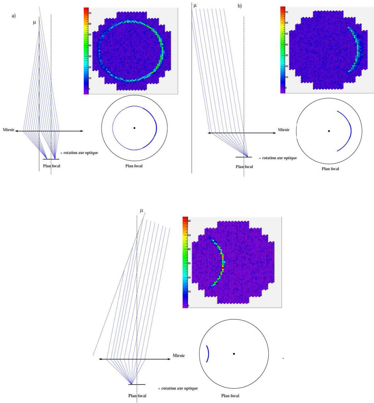
FIGURE 6.1 – Comportement d'un anneau de muon en fonction du paramètre d'impact et de l'inclinaison du muon avec l'axe optique. En haut à gauche, muon tombant dans le miroir. En haut à droite, muon tombant à l'extérieur du miroir. En bas, muon tombant à l'extérieur avec un angle non nul par rapport à l'axe optique.
