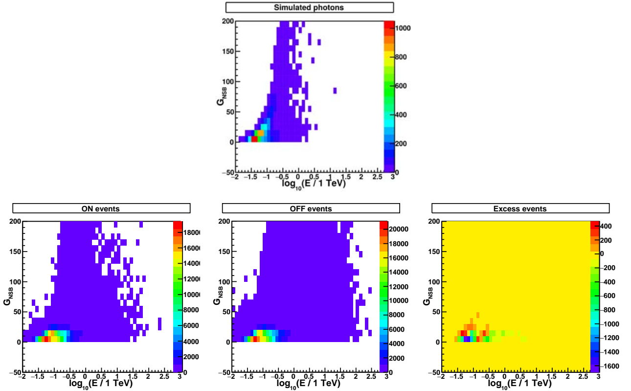
FIGURE 8.11 – Distribution du NSB Goodness en intensité G_{NSB} en fonction de l'énergie reconstruite pour les événements issus de l'analyse de photons simulés (en haut) et de PKS 2155-304 (en bas). Parmi ces derniers, les événements des régions ON sont représentés à gauche, ceux des régions OFF au centre et l'excès à droite.
