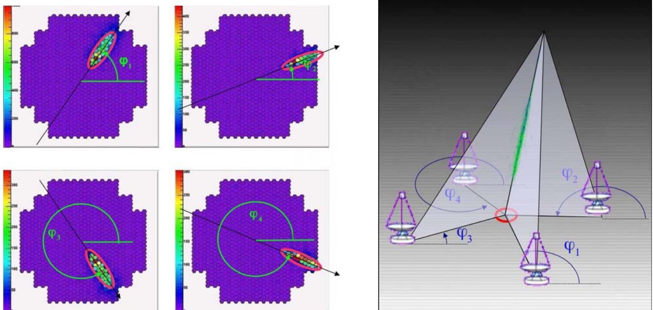
FIGURE 7.3 – Reconstruction géométrique du paramètre d'impact de la gerbe en mode stéréoscopique. L'angle \varphi_i entre le grand axe de l'ellipse et l'axe x de la caméra correspond à la direction du plan qui contient le télescope et la trajectoire de la gerbe. L'intersection de ces plans donne directement le paramètre d'impact sur le sol. Figure issue de [De Naurois, 2012]
