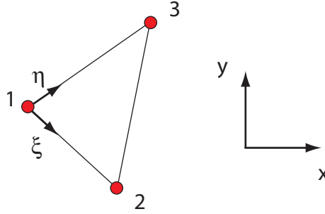
Figure 5.3: Triangular MINI element
