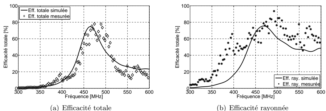
FIGURE 4.36 – Efficacité de l'antenne à 466 MHz avec petit plan de masse.
