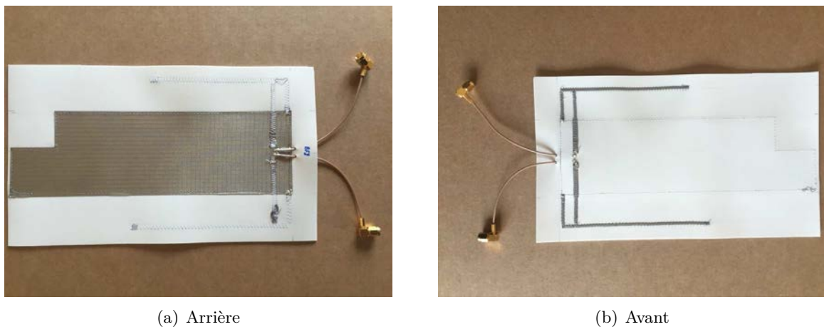
FIGURE 4.51 – Antenne bi-fréquence avec plan de masse unique réalisée.
