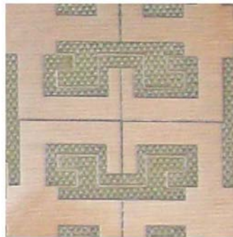
(a) Cellule du CMA
