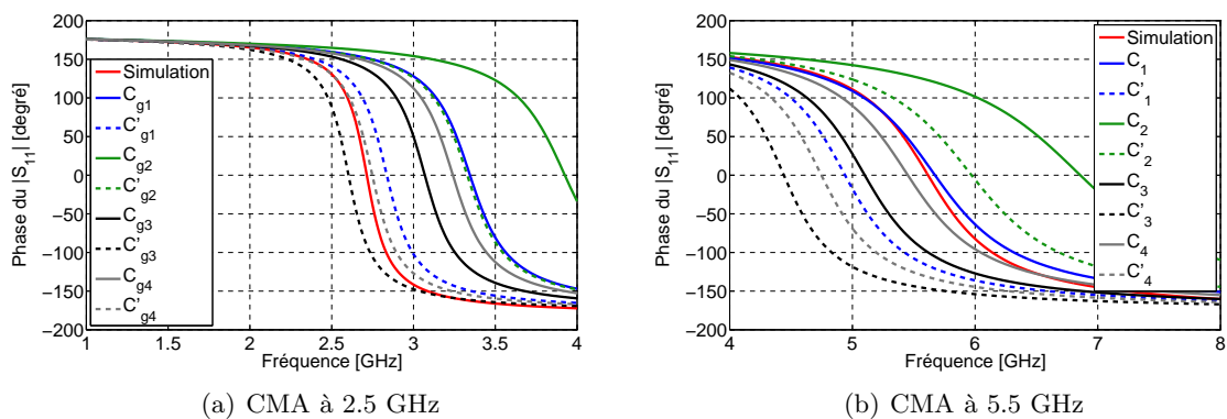
FIGURE 5.20 – Phase du coefficient de réflexion simulé comparée à quatre modèles.
