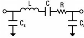
FIGURE 5.24 – Schéma équivalent d'une capacité interdigitée [143].
