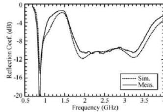
(b) Coefficients de réflexions simulé et mesuré
