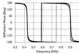
(b) Simulation de la phase réfléchie, trait pointillé : P = 10mm
