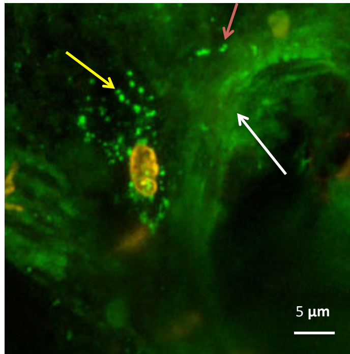
Figure 20. Visualisation du biofilm sur Dacron® traité par daptomycine – rifampicine Visualisation pour double marquage Syto9® (cellules vivantes en vert) et Iodure de Propidium (cellules mortes en rouge). La flèche blanche désigne les structures extracellulaires du biofilm. La flèche rouge signale un corps bactérien vivant (vert) enchâssé dans cette structure et la flèche jaune des bactéries en position intracellulaire (cellule en voie de mort cellulaire car noyau marqué à l'IP)
