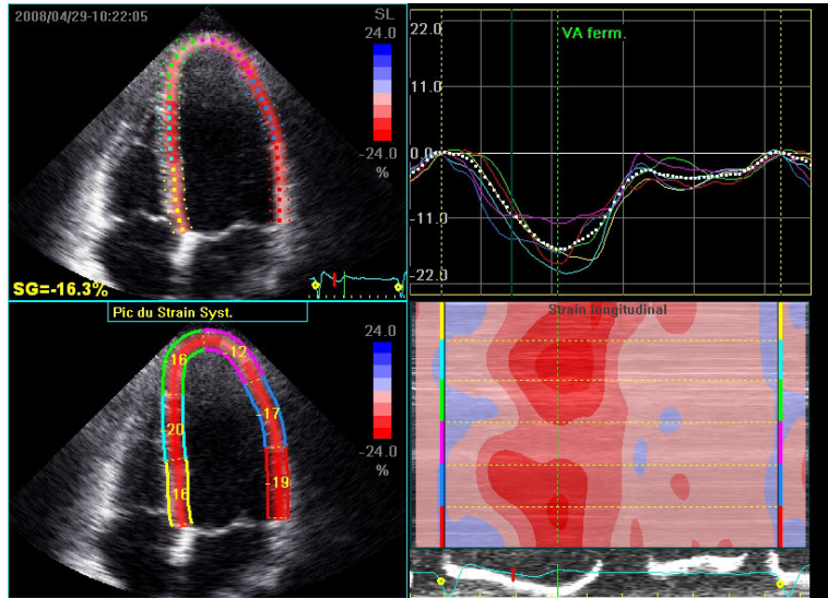
Figure 6 : Exemple de courbe de strain longitudinal, déterminé à partir d'une coupe apicale 4 cavités (données personnelles)
