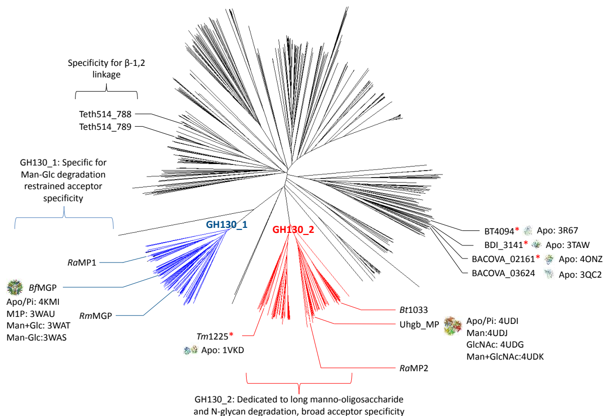
Figure 22: Représentation radiale de l'arbre phylogénétique de la famille GH130, en Janvier 2015.
