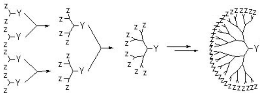
Figure 28 - Schématisation du principe de synthèse convergente de dendrimère, des dendrons vers le coeur (Y= point focal et Z= surface du dendrimère).
