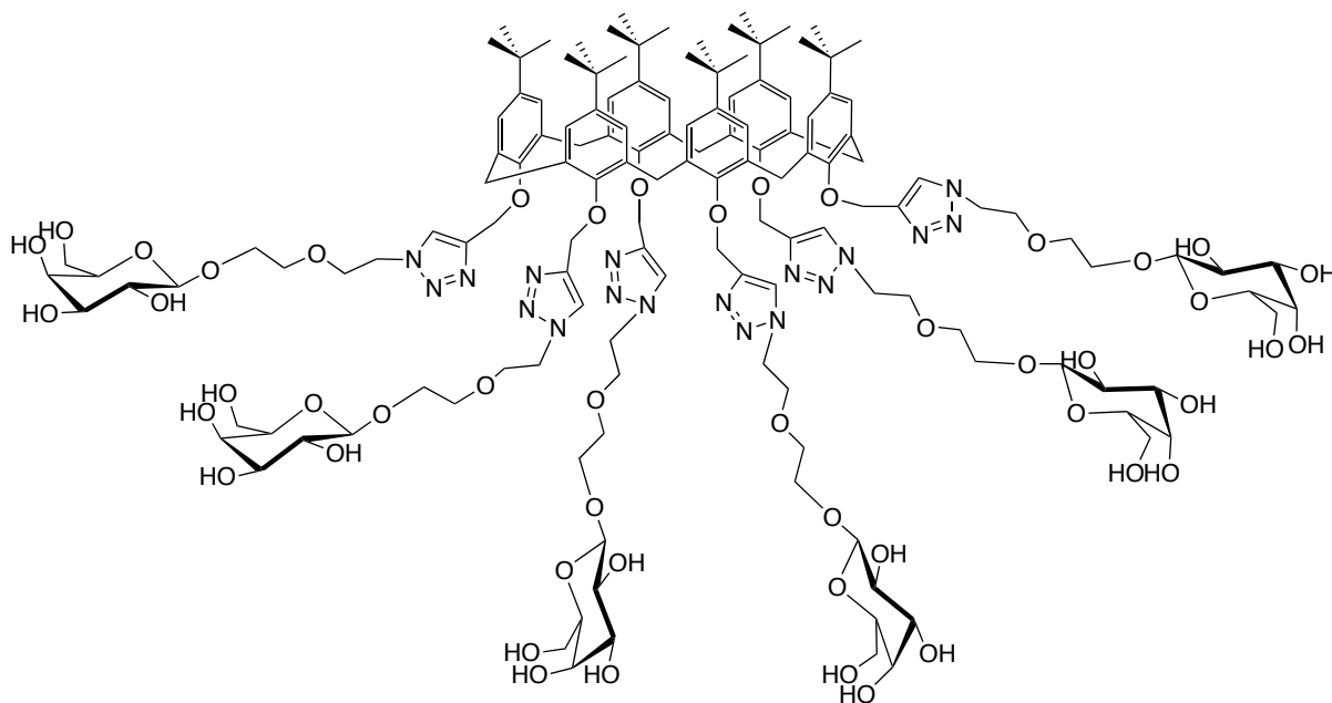
Figure 19 - Glycocluster développé par Vidal et al..
