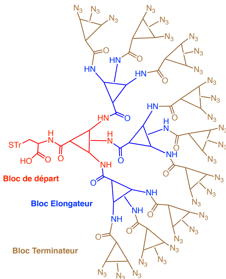
Figure 44 - Modèle de dendrimère synthétisé avec 3 parties : le bloc de départ en rouge, le bloc Elongateur en bleu et le bloc Termineur en marron.
