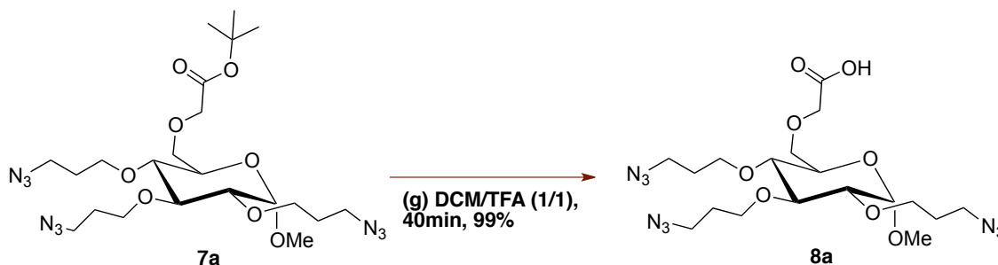
Figure 59 - Déprotection de l'acide carboxylique de 7a pour l'obtention du bloc Terminateur issu de l' \alpha -D-glucopyranoside de méthyle.
