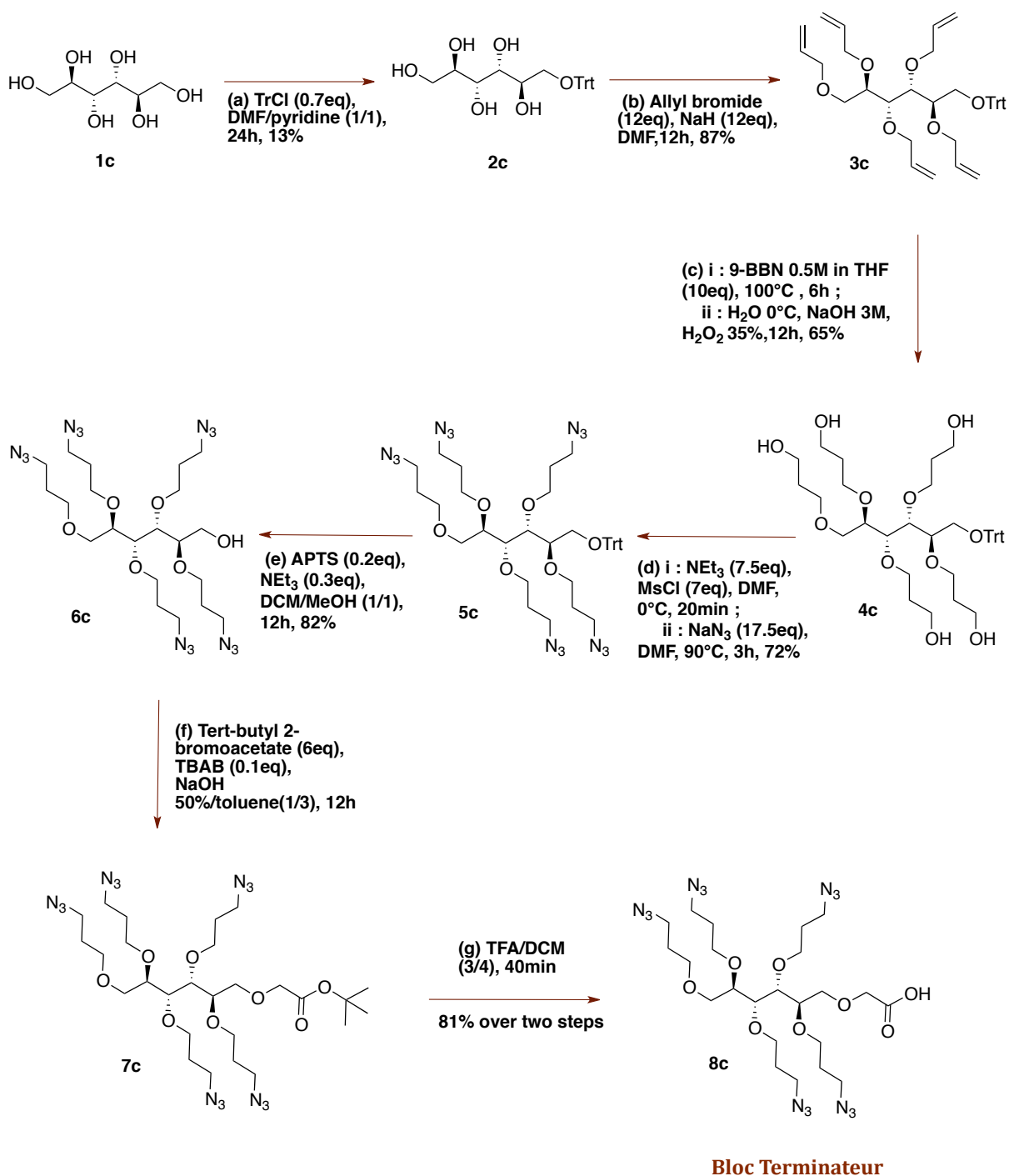
Figure 68 - Schéma de synthèse de 8c , du bloc Terminateur issu du D-mannitol.
