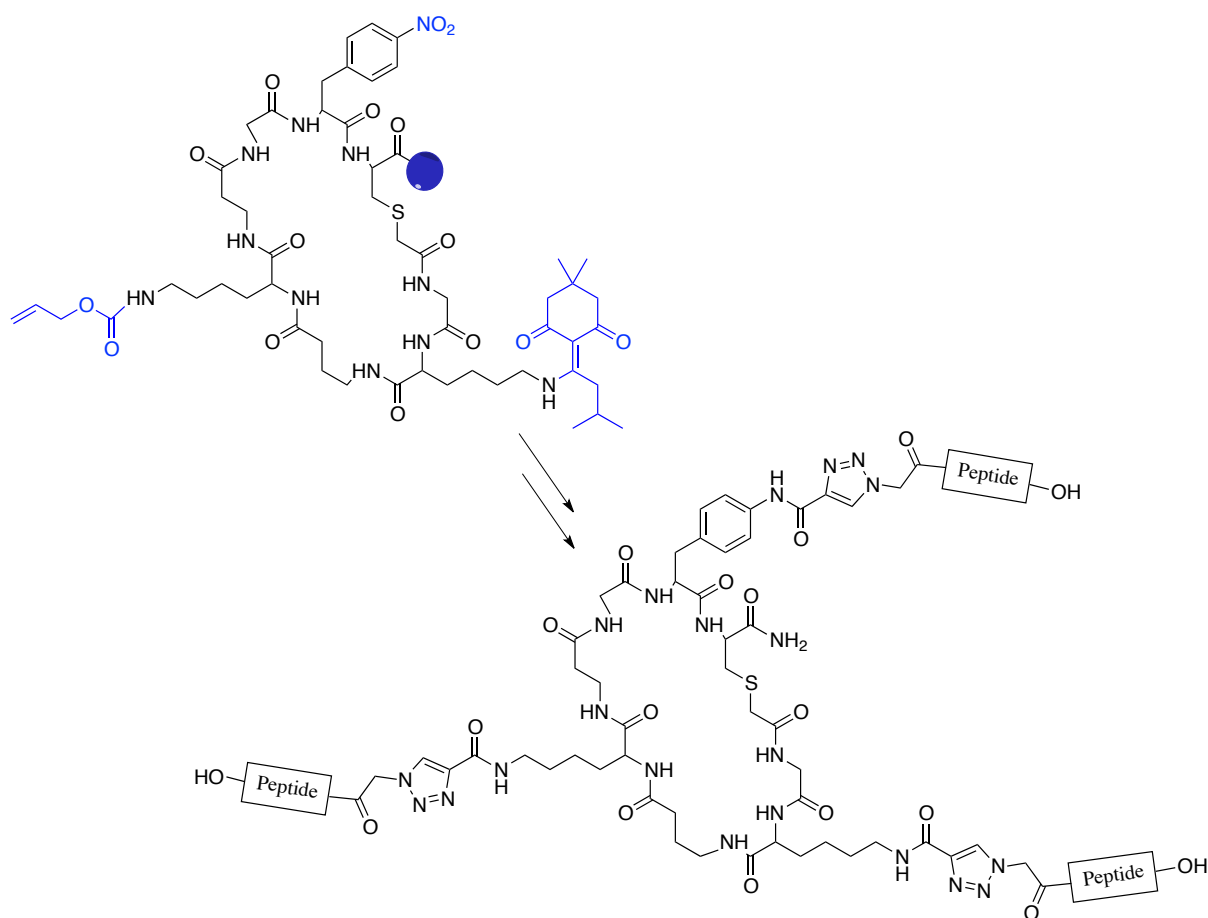
Figure 99 - Triple CuAAC sur une résine de type Tentagel S Ram de Franke et al..
