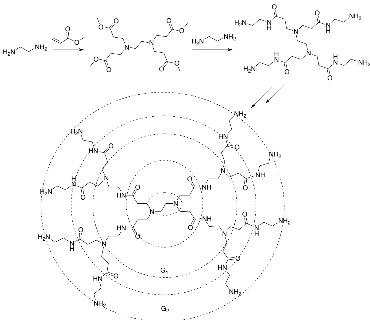
Figure 35 - Synthèse d'un dendrimère PAMAM de génération G_2 .
