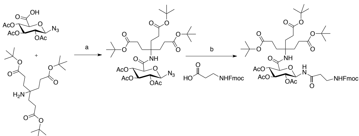
Figure 33 - Synthèse d'un monomère de glycopeptidodendrion - a : DIC, HOBT, DCM, 12h, 53% ; b : DIC, HOBT, PMe 3 , THF, 0°C-rt, 12h, 68%.
