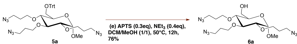
Figure 56 - Détritylation de l'alcool primaire de 5a .
