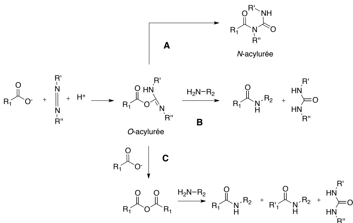
Figure 82 - Différentes réactions de couplage peptidique activées par du DCC - voie A : réarrangement en N-acylurée ; voie B : formation du peptide voulu ; voie C : formation de l'anhydride sachant que R_1' est l'épimère de R_1 .
