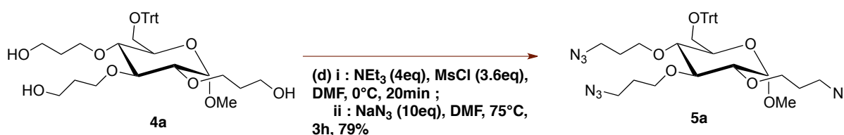
Figure 55 - Per-métylation et per-azidation de 4a.
