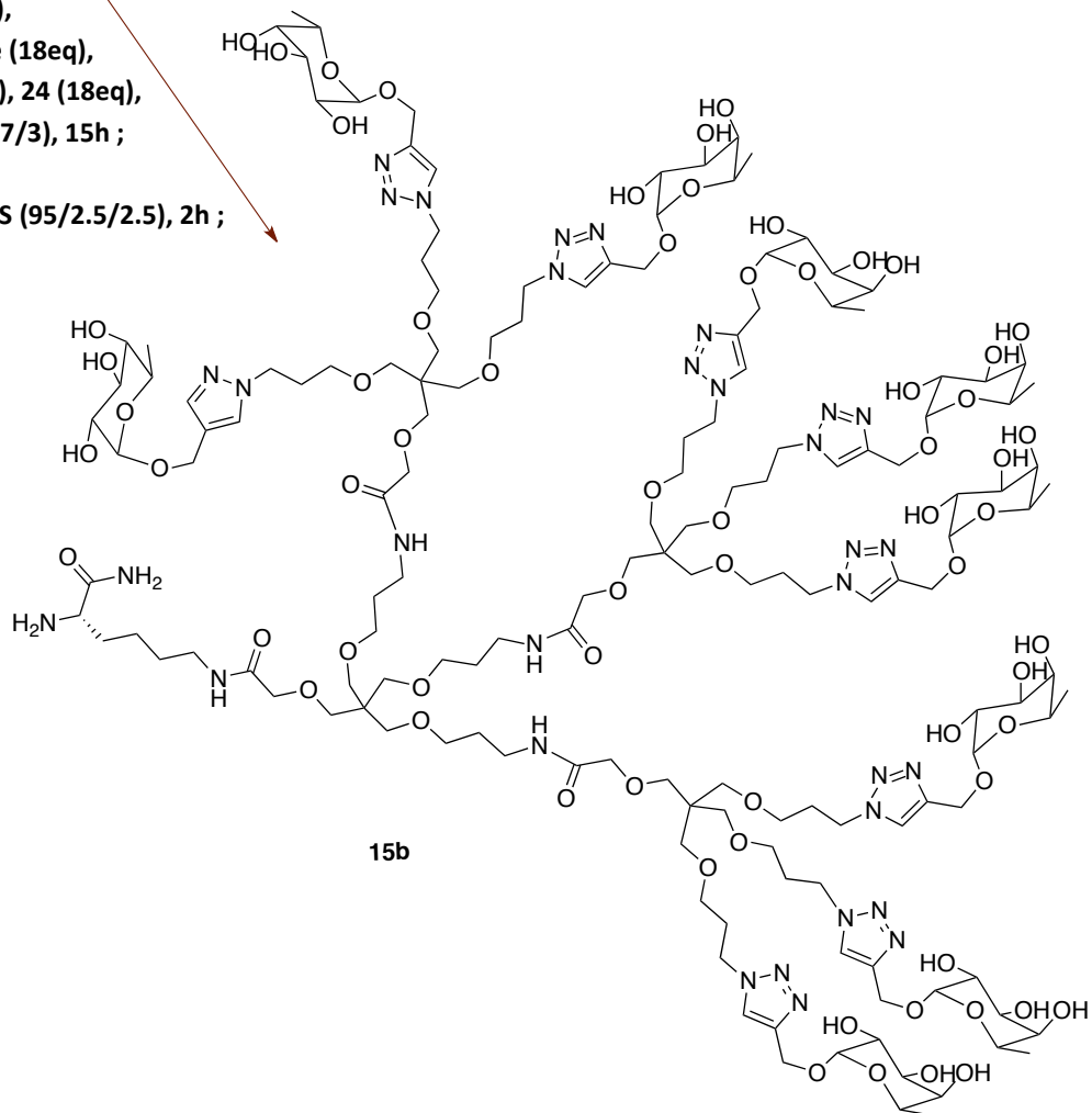
Figure 126 - Réaction de CuAAC et Clivage de 12b.
