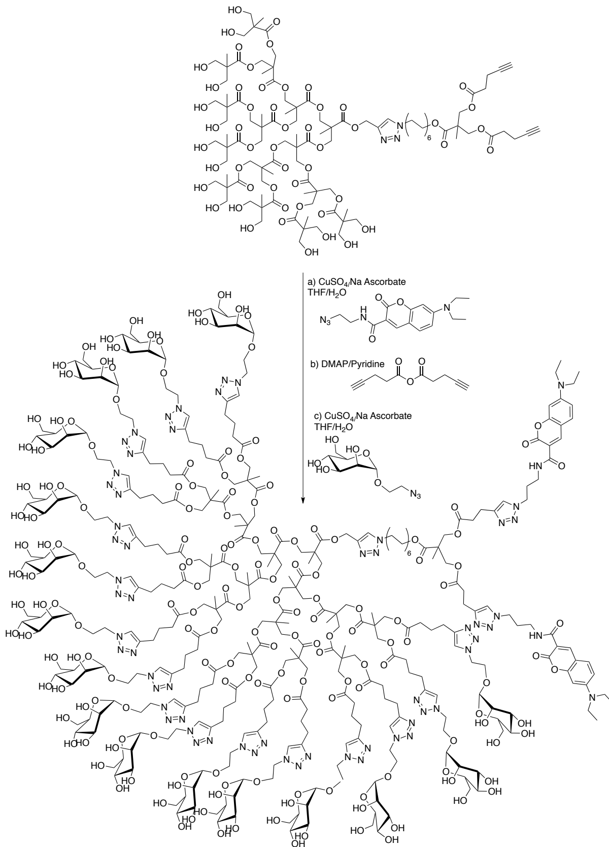
Figure 41 - Exemple d'un glycodendrimer issu du bis-MPA synthésé par Hawker et al..
