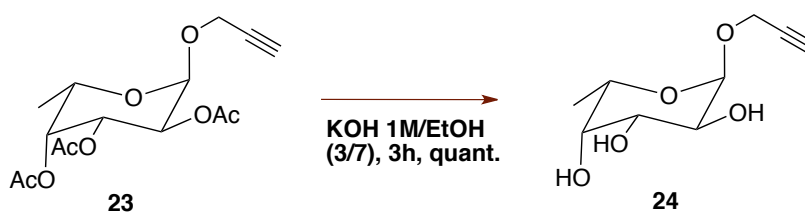
Figure 72 - Désacétylation de 23 .
