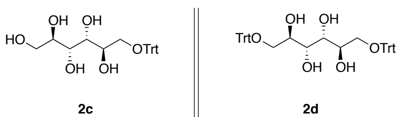
Figure 67 - D-mannitol monotritylé à gauche, et D-mannitol ditritylé à droite.
