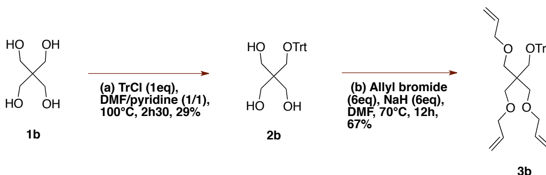
Figure 63 - Tritylation et per-allylation du pentaérythritol.
