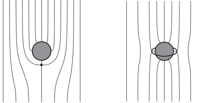
FIGURE 1.3 – Configurations dipolaire et quadrupolaire [131].
