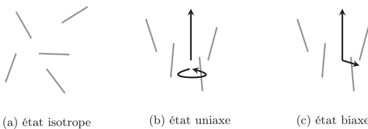
FIGURE 1.2 – Les différents degrés de symétrie dans \mathcal{S}_0 .
