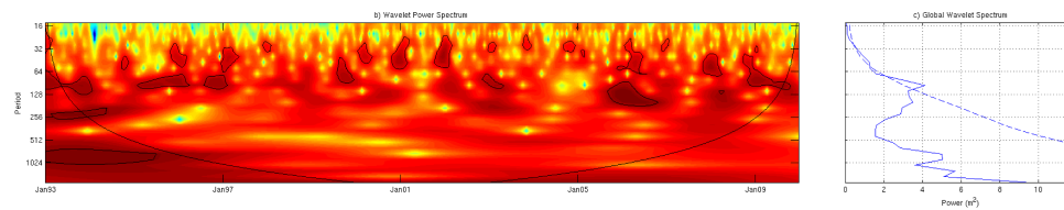
Fig. V.9 Analyse en ondelette (bas) et spectre d'énergie (droite, la ligne pointillée représente la significativité 99%) de la PC-2.
