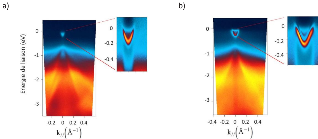
Figure IV-41 : 4 MC de Bi recuites et déposées sur InAs(111) : a) face A ; b) face B.
