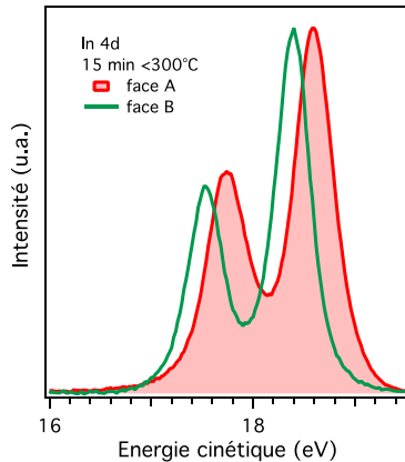
Figure IV-24 : Recuit à T < 300^{\circ}\text{C} : comparaison entre la face A (en rouge) et la face B (en vert) de a) In 4d et b) Bi 5d 5/2 .
