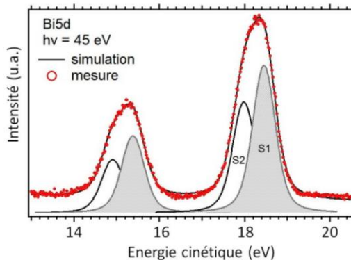
Figure IV-25 : Niveau de cœur Bi 5d, de la surface 4 MC Bi/InAs(111) B (2x2), a) mesuré à température ambiante sans recuit b) à température ambiante après recuit.
