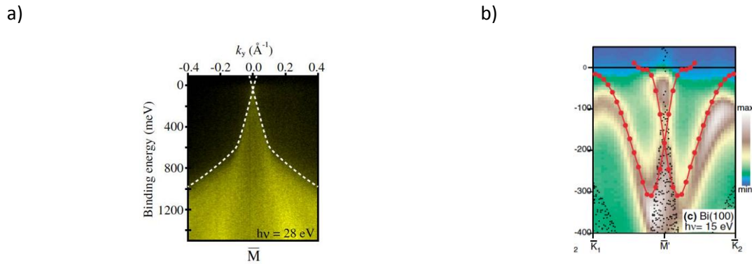
Figure IV-37 : a) Image ARPES dans la direction MK [Ohtsubo13] ; b) Structure électronique au point M. Les points noirs représentent la projection de la structure électronique de volume. Les points et lignes en rouge montrent les états de surface [Koroteev04].
