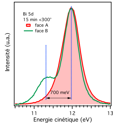
Figure IV-24 : Recuit à T < 300^{\circ}\text{C} : comparaison entre la face A (en rouge) et la face B (en vert) de a) In 4d et b) Bi 5d 5/2 .
