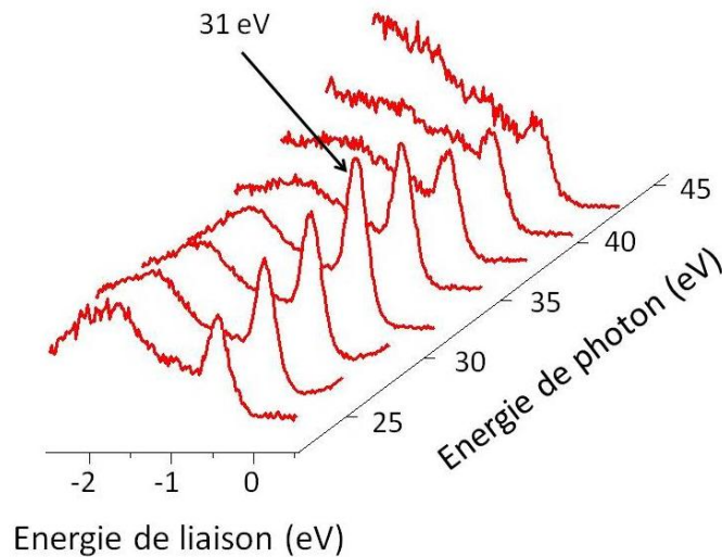
Figure III-25 : Pic de résonance observé à 31 eV
