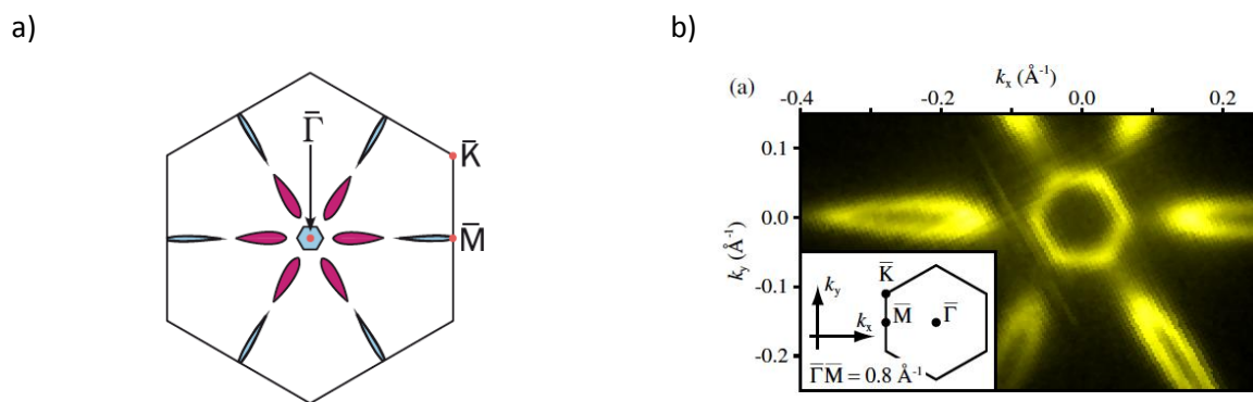
Figure IV-38 : a) Représentation schématique de la surface Fermi de Bi(111) dans la zone de Brillouin de surface [Hirahara06] ; b) Surface de Fermi déterminée par ARPES [Ohtsubo13].
