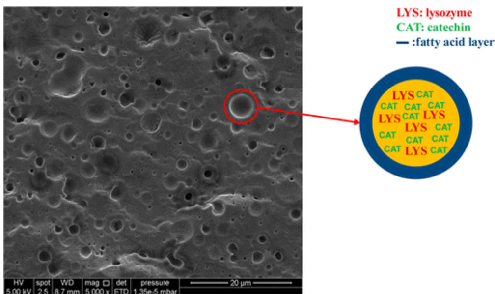
Figure 12 : Cliché de films composites à base de zéine, d'acides gras et de lécithine, incorporés avec du lysozyme et de la catéchine en tant qu'agents actifs : Présentation schématique de microsphères formées dans la matrice protéique[96].
