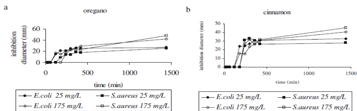
Figure 19 : Diamètres d'inhibition obtenus en milieu de culture gélosé ensemencé par des bactéries E.coli ou S.aureus en fonction du temps d'exposition aux huiles essentielles d'origan (a) et de cannelle (b) en phase vapeur[163]
