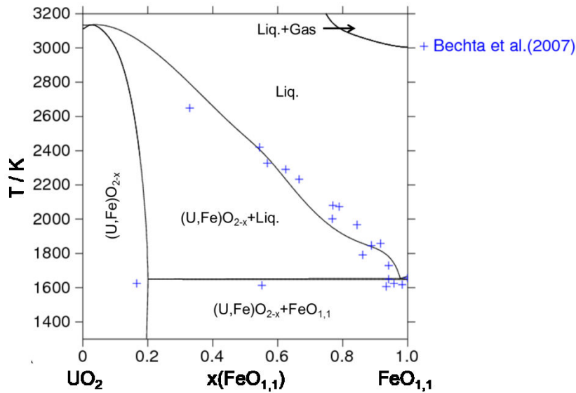
Figure 12 : Section UO_2 - FeO_{1,1} calculée avec le modèle développé pendant la thèse. Comparaison avec les points expérimentaux de Bechta et al. [20]
