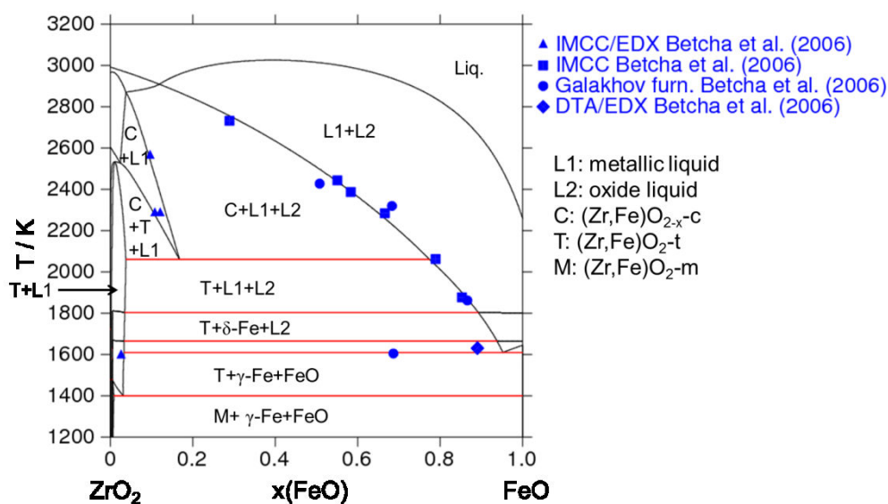
Figure 11 : Section ZrO_2 -FeO calculée avec notre modèle. Comparaison avec les points expérimentaux de Bechta et al [17]
