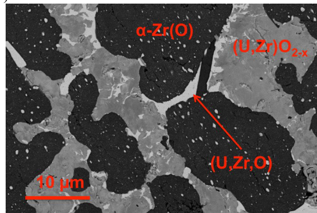
Figure 5 : (a) Image MEB en électrons rétrodiffusés (BSD) de l'échantillon OUZr_1 ; (b) Agrandissement de la microstructure dendritique ; (c) les trois phases identifiées : (U,Zr)O_{2-x} , \alpha -(Zr,U)(O) et une phase métallique enrichie en U
