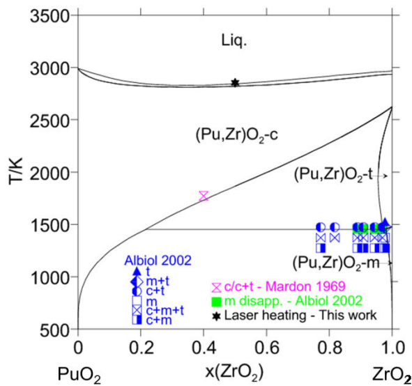
Figure 13 : Section PuO_2 - ZrO_2 , où les points expérimentaux de Mardon et al. [12] et Albiol et al. [21] ont été reportés
