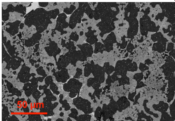
Figure 5 : (a) Image MEB en électrons rétrodiffusés (BSD) de l'échantillon OUZr_1 ; (b) Agrandissement de la microstructure dendritique ; (c) les trois phases identifiées : (U,Zr)O_{2-x} , \alpha -(Zr,U)(O) et une phase métallique enrichie en U
