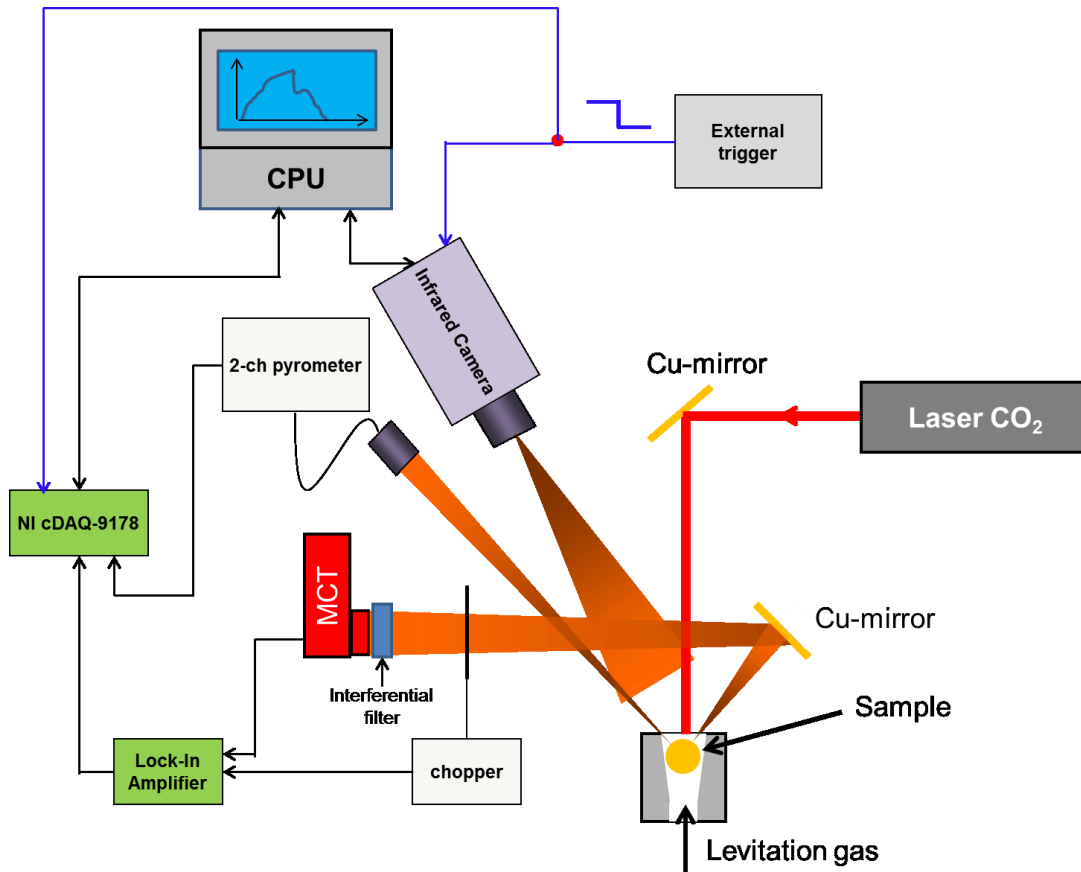
Figure 16 : Schéma du dispositif expérimental ATILHA
