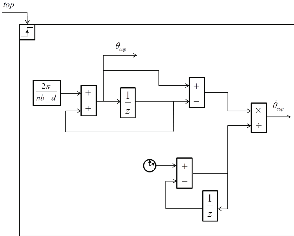
Figure 31 : Modèle de capteur incrémental seconde partie
