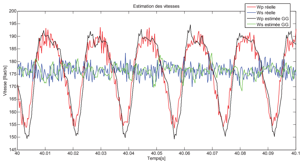
Figure 76 : Estimation de la vitesse primaire et de la vitesse secondaire par l'observateur à grand gain continu-discret sur les données réelles.
