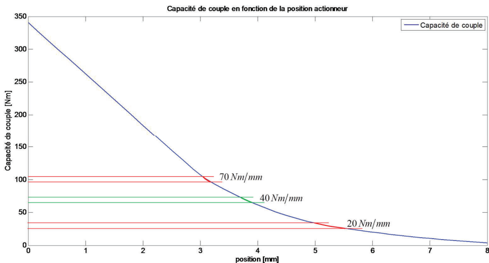
Figure 96 : Résolution en couple de l’actionneur d’embrayage
