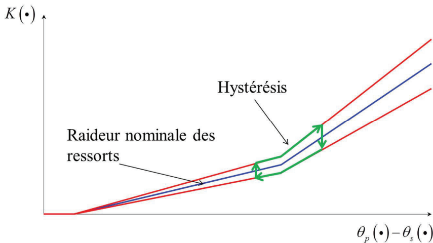
Figure 56 : Caractéristique de la raideur des ressorts du double volant amortisseur
