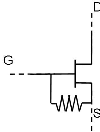
FIGURE 3.11: Schéma d'une contre-réaction entre la grille et la source à travers une résistance
