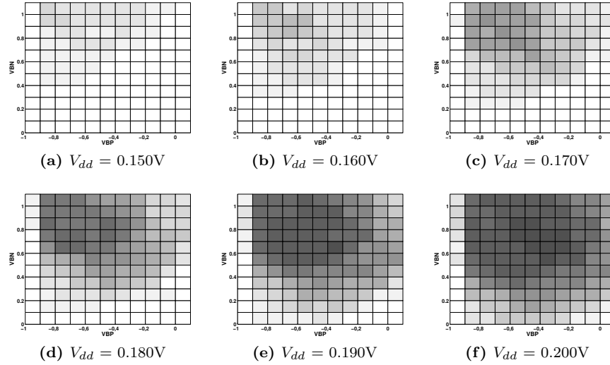
Figure D.23: Rendement mesuré de l'architecture TGPL-Data dans l'espace ( V_{dd} , G_{nds} ) à 25°C. Plus le carré est sombre, plus le rendement est élevé.
