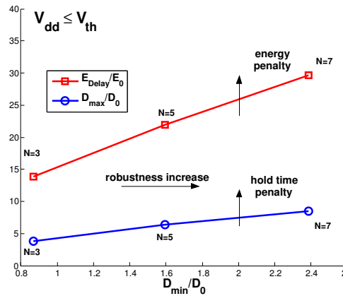
(b) La dissipation énergétique et le délais maximum ( \mu + 3\sigma ) en fonction du délais minimum ( \mu - 3\sigma ) d'une chaîne d'inverseurs ( N = 3, 5 and 7 )
