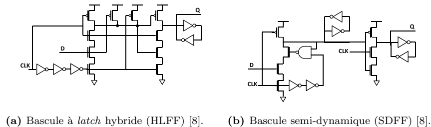
Figure D.4: Bascule semi-dynamiques à impulsion implicite.
