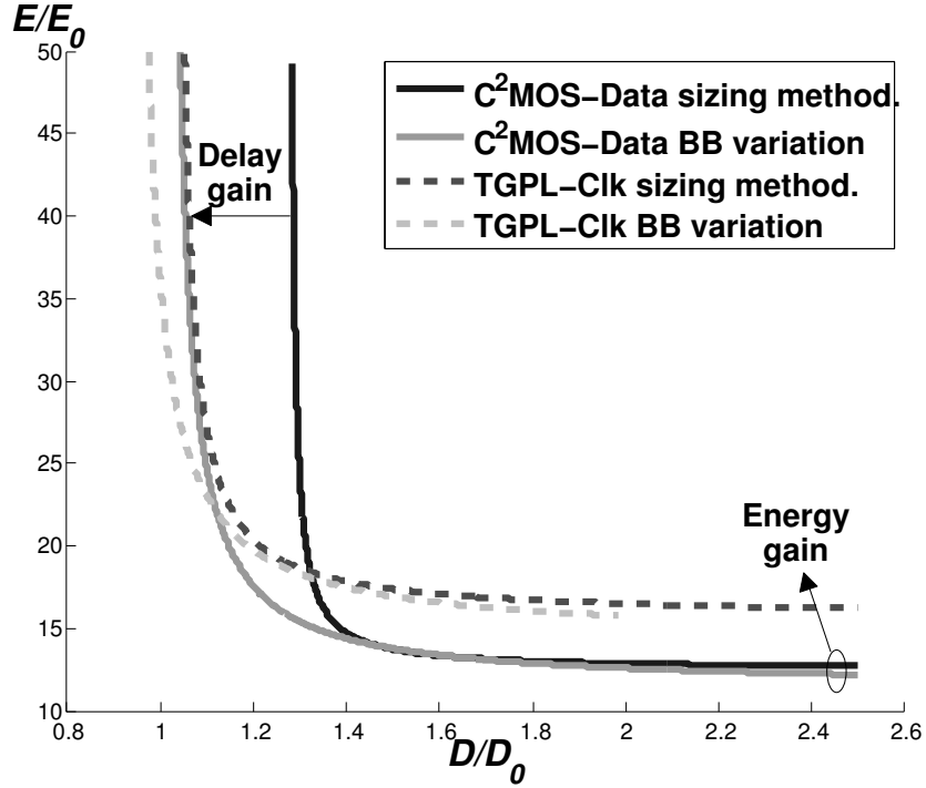
Figure D.13: CEEs des architectures C 2 MOS-Data et TGPL-Clk extraites partir de l'algorithme de dimensionnement et partir d'une polarisation face arrière ( V_{dd} = 1V , V_{dds}/Gnds range = \pm 1V , \alpha_{sw} = 0.15 , T_{clk} = 40FO4 , température 70^\circ C ). La technique de polarisation face arrière applique sur une large gamme fournie de meilleures performances en dlais et nergie que la mthodologie de dimensionnement.
