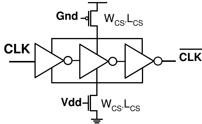
Figure D.19: Architecture du générateur de délais (GD) proposé [70].
