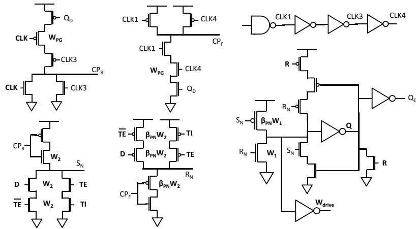
Figure D.10: CP 3 L-Data, version avec scan et reset de l'architecture CP 3 L de la figure 1.21.
