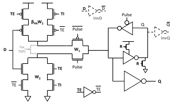
(b) Le latch C 2 MOS-Xor avec des inverseurs pour les signaux \bar{D} et \bar{Q}_d .
