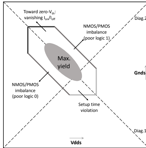
Figure D.24: Comportement schématique du rendement dans l'espace V_{dd} - G_{nds} .
