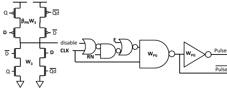
(a) Le générateur d'impulsion conditionnelle.
