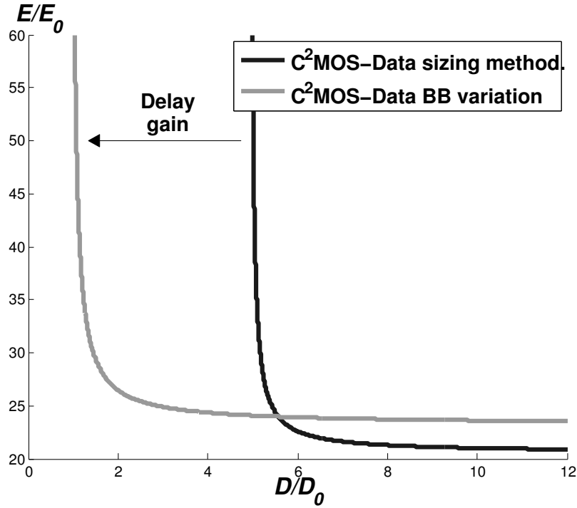
Figure D.14: CEEs de l'architecture C^2MOS-Data extraites partir de l'algorithme de dimensionnement et partir d'une polarisation face arrière ( V_{dd} = 0.35V , \alpha_{sw} = 0.15 , T_{clk} = 40FO4 , température 25^\circ C ).
