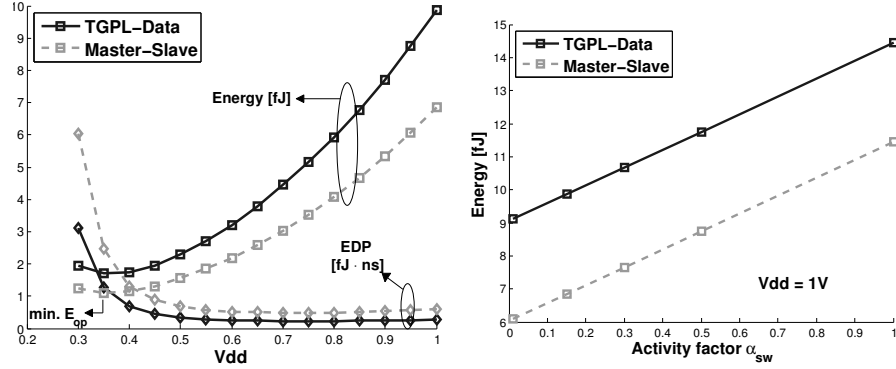
(a) Évolution de l'énergie moyenne par cycle ( \alpha_{sw} = 15\% ) et du produit énergie-délais avec le facteur d'activité. (PED) avec la tension d'alimentation.
