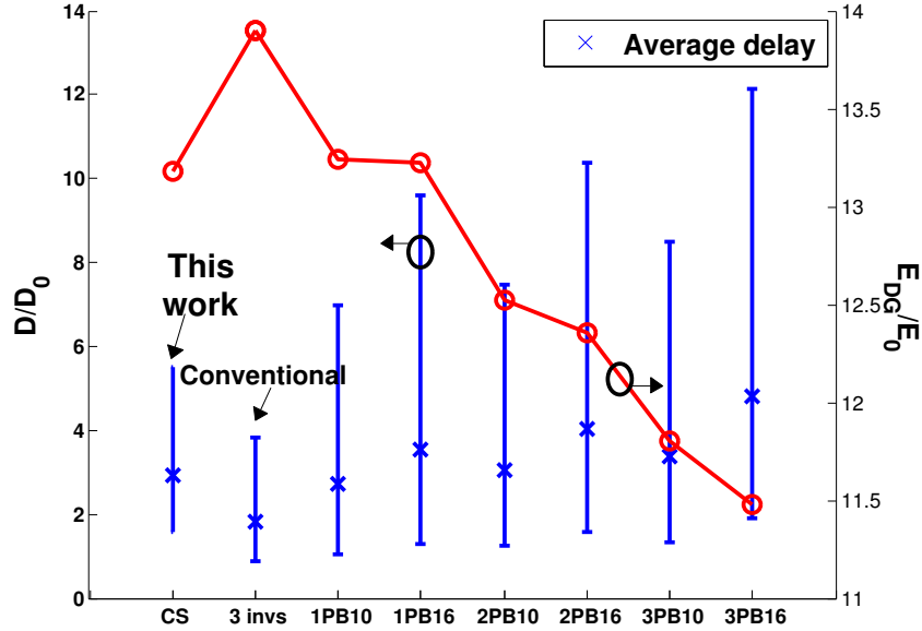
Figure D.21: Comparaison des performances énergétiques et en délais dans le régime sous-seuil ( V_{dd} = 0.3V ). Le nom indique l'augmentation de la longueur de polysilicium et le nombre d'étages présentant celle-ci.
