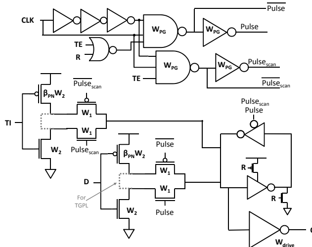
Figure D.8: Les bascules TGPL-Clk and C 2 MOS-Clk (respectivement avec et sans les pointillés), deux variantes de l'architecture TGPL de la figure D.5.
