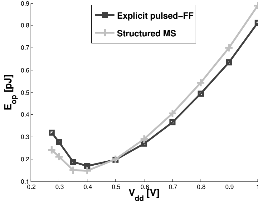
Figure D.30: Energie par opération sur une large gamme de tension ( G_{nds} = V_{dds} et \alpha_{rate} = 15\% ). Le banc de registres composé de bascules à impulsion explicite présente une plus faible consommation énergétique pour des V_{dd} au-dessus du seuil, et une optimale à 0.35V.
