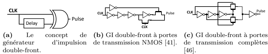
Figure D.6: Générateurs d'impulsion (GIs) double-front.
