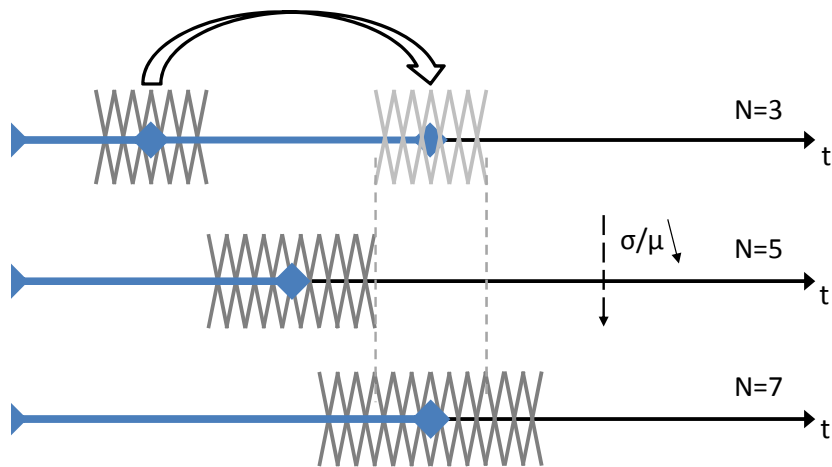
Figure D.20: L'architecture de GD dite current-starved effectue une translation sans expansion de la fenêtre de délais sur la ligne du temps. En d'autres mots, elle augmente le délais moyen sans augmentation notable de la dispersion.
