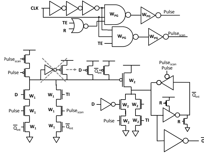
Figure D.9: La version avec scan et reset de l'architecture CDFD de la figure 1.17d
