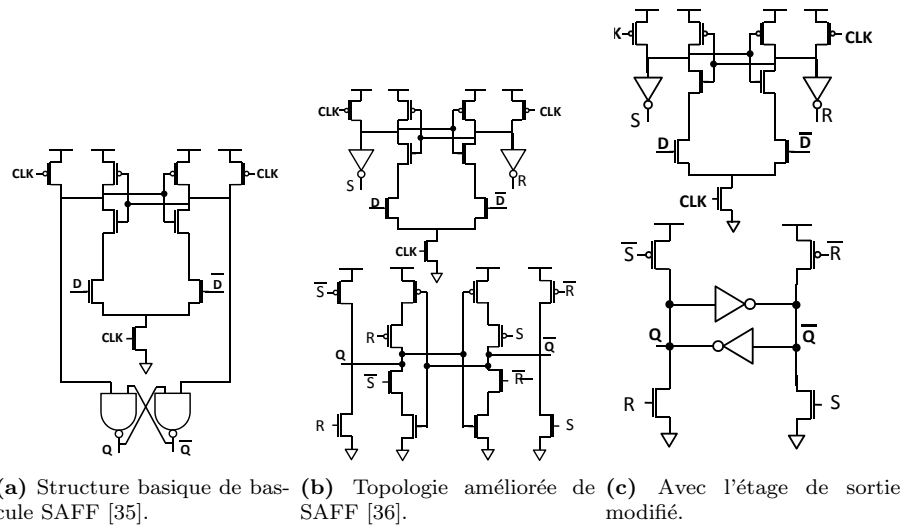
Figure D.3: Bascules différentielles basées sur le sense-amplifier .
