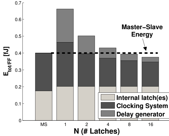
Figure D.27: L'énergie par bascule fonction du nombre de latches partageant un GI. Les barres représentent les proportions de l'énergie consommée dans le générateur de délais, la partie "horlogée" (les signaux CLK et Pulse ) et le latch pris isolément. V_{dd}=1V , T_{clk} = 40FO4 , \alpha_{sw} = 15\% .
