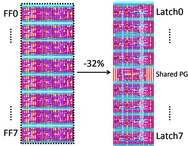
Figure D.28: Le bloc de 8 bascules à impulsion (droite) a 32% de surface en moins que les 8 bascules maître-esclave.
