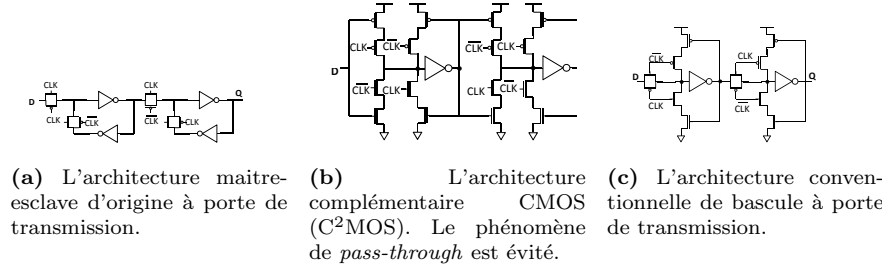
Figure D.2: Architectures maître-esclave conventionnelles. TGFF donne un meilleur compromis entre la vitesse et le phénomène pass-through .
