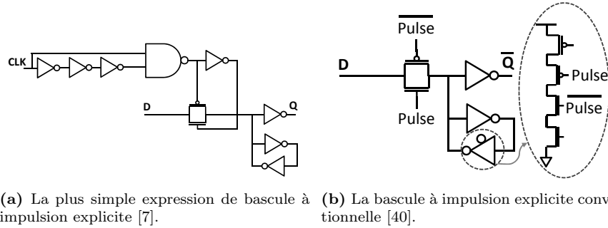
Figure D.5: Les structures basiques de bascules à impulsion explicite.
