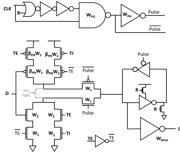
Figure D.7: Les bascules TGPL-Data and C 2 MOS-Data (respectivement avec et sans les pointillés), deux variantes de l'architecture TGPL de la figure D.5.
