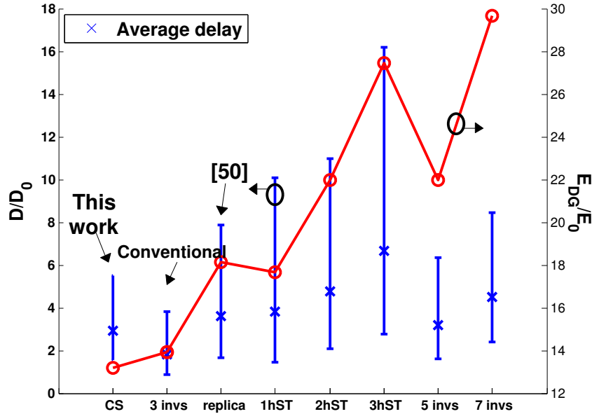
Figure D.22: Comparaison des performances énergétiques et en délais dans le régime sous-seuil ( V_{dd} = 0.3V ), pour différentes architectures de GD.
