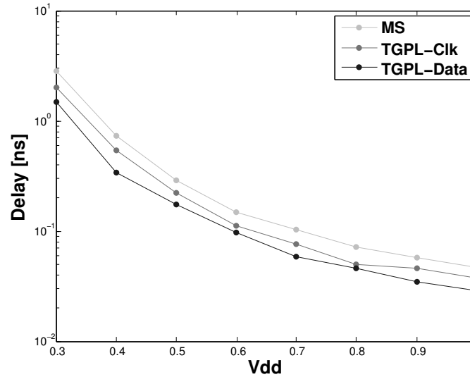
Figure D.15: Délais mesurés de 0.3V à 1V dans le cas nominal ( V_{dds}=G_{nds}=0V ). Le délai Clk-Q est plus faible pour la TGPL-Data que pour la TGPL-Clk, contrairement au délai entrée-sortie ( T^{\circ}=80^{\circ}C ).
