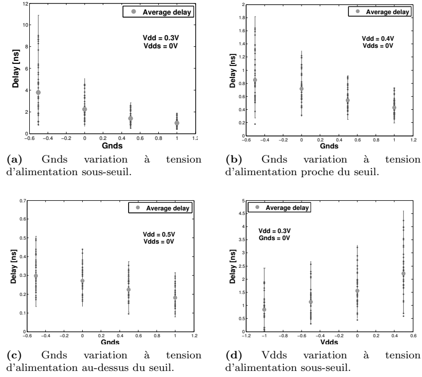
Figure D.16: Évolution du délais mesuré avec Vdds et Gnds.
