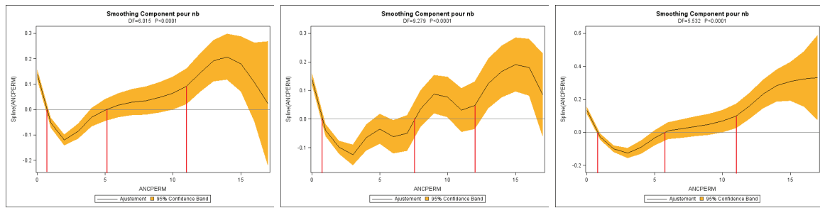
FIGURE 3.7 – Influence non linéaire de l’ancienneté du permis sur la sinistralité totale entre 2008 et 2010
