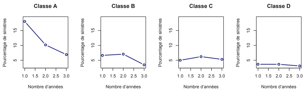
FIGURE 3.13 – Évolution du nombre moyen de sinistres responsables annuel entre 2008 et 2010
