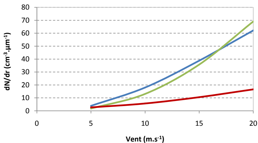
Figure 4-9 : Concentration en fonction de la vitesse du vent pour des particules de 1 \mu\text{m}
