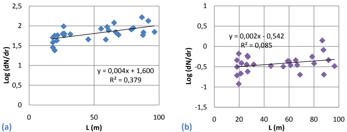
Figure 5-27 : Concentration en particules de 0.5 µm (a) et 5 µm (b) en fonction de la longueur d'onde des vagues, vent SO
