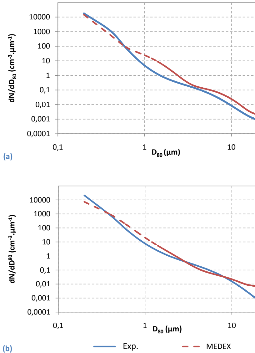
Figure 2-6 : Concentrations calculées par MEDEX (pointillé rouge) et mesurées (trait plein bleu) sur l'Atalante (MIRAMER 2008) en fonction du diamètre des particules : (a) X=7 km et U=5 m.s -1 et (b) X=250 km et U=10 m.s -1
