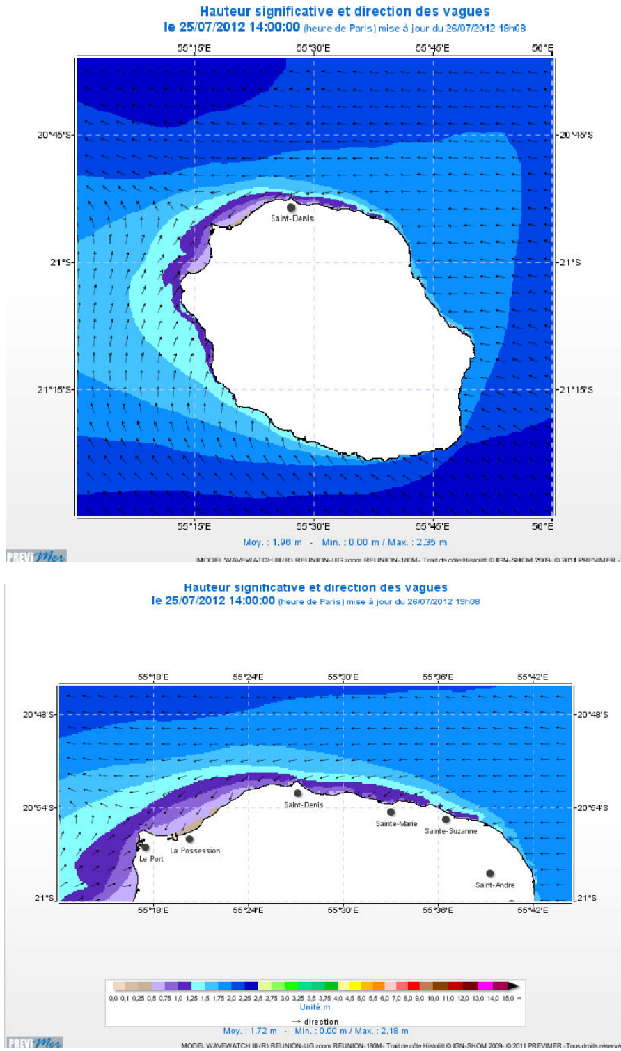
Figure 8-6 : Hauteur significative et direction des vagues issue du modèle wawewatch III à la Réunion le 25/07/2012 à 14h (PREVMER)
