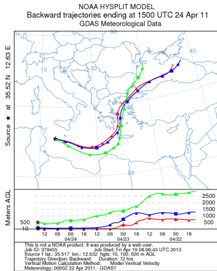
Figure 6-8 : Retro-trajectoire à Lampedusa le 24/04/2011 à 15h (Hysplit)
