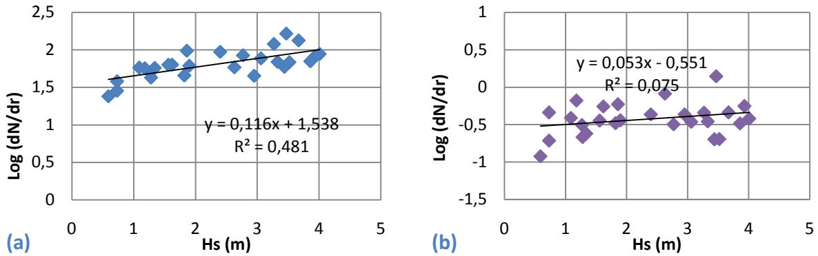
Figure 5-26 : Concentration en particules de 0.5 µm (a) et 5 µm (b) en fonction de la hauteur significative des vagues (vent SO)
