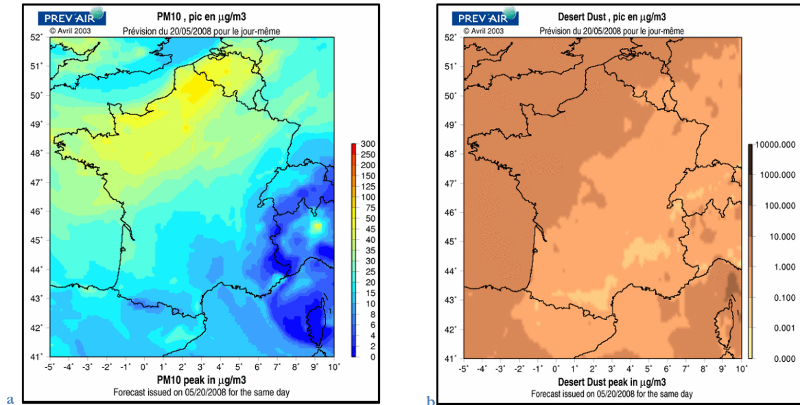
Figure 9-2 : Pic de PM 10 (a) et de poussières désertiques (b) le 20 mai 2008 (PREV'AIR)
