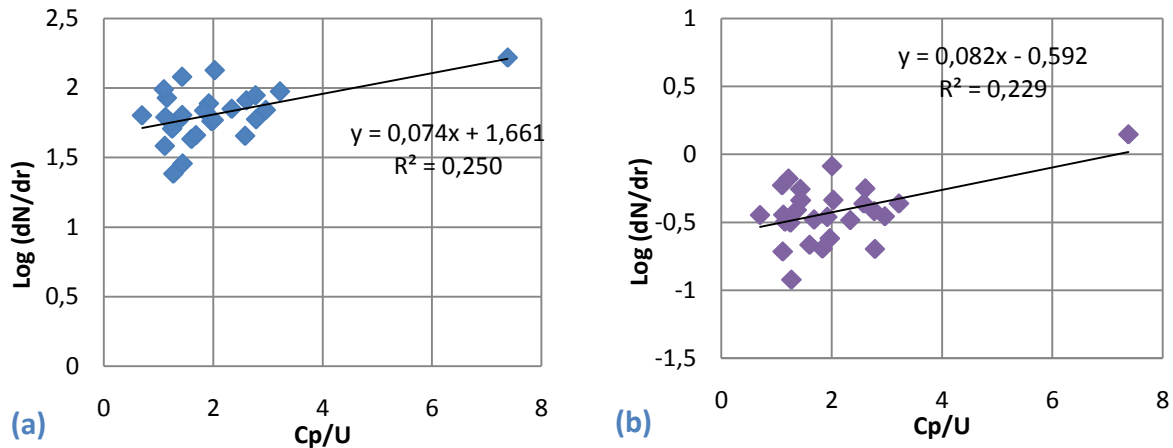
Figure 5-32 : Concentration en particules de 0.5 µm (a) et 5µm (b) en fonction de l'âge des vagues, vent SO
