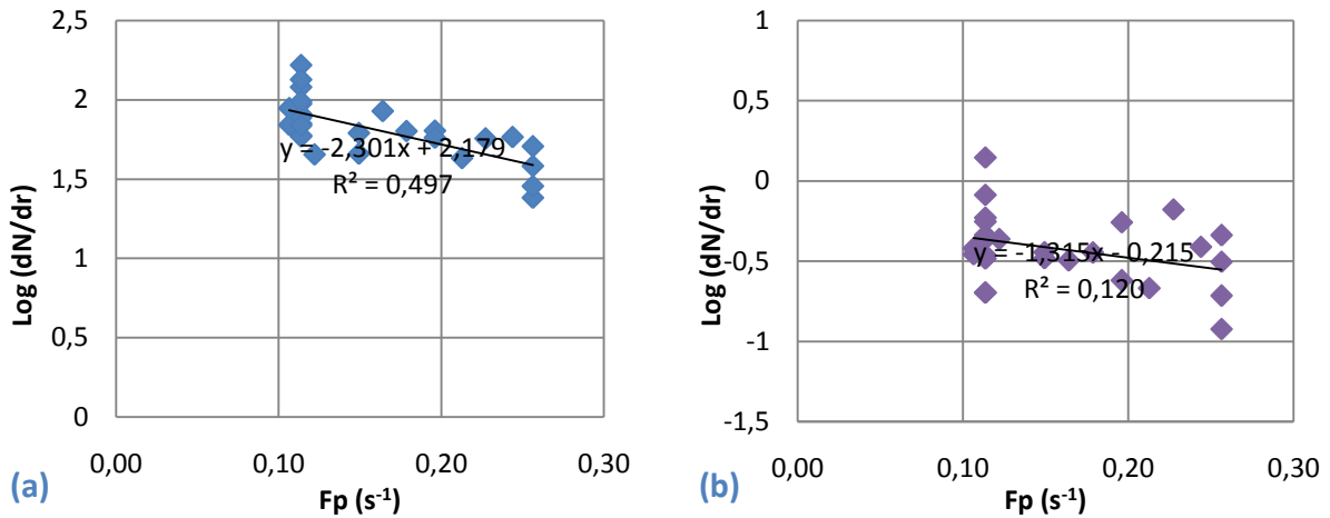
Figure 5-30 : Concentration en particules de 0.5 µm (a) et 5µm (b) en fonction de la fréquence pic des vagues, vent SO
