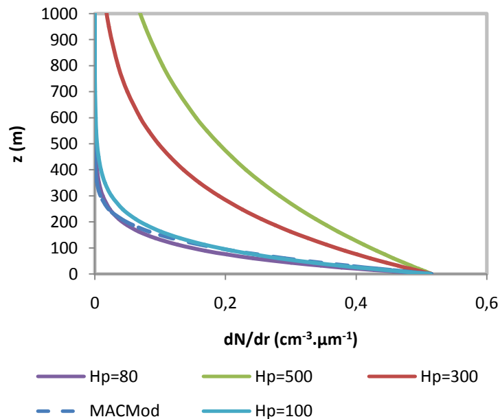
Figure 4-13 : Comparaison profil vertical modélisé par MACMod et théorique pour différentes valeurs du paramètre d'échelle et des particules de 1 µm.
