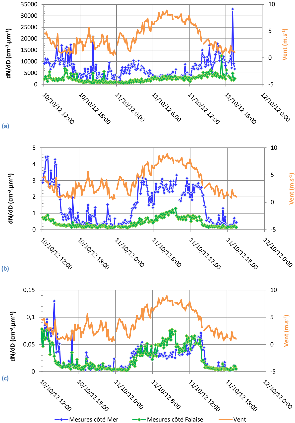
Figure 8-14 : Concentration mesurée « côté mer » et « côté falaise » de la route et vitesse du vent pour des particules de diamètre égal à 0.21 µm (a), 1.5 µm (b) et 8 µm (c) (Heure UTC).
