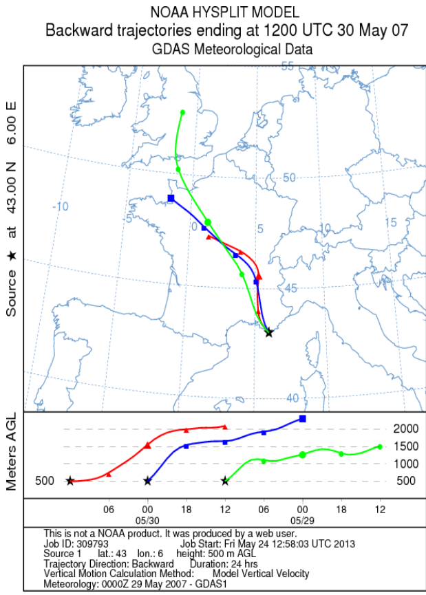
Figure 7-4 : Rétrotrajectoire durant un épisode de Mistral à Porquerolles (HYSPLIT)
