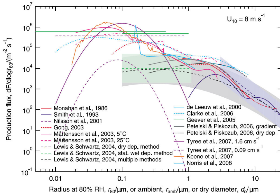
Figure 2-5 : Flux de production des aérosols marins en fonction de la taille des particules calculés à partir de diverses fonctions sources, pour un vent de 8 \text{ m.s}^{-1} (De Leeuw et al. 2011)
