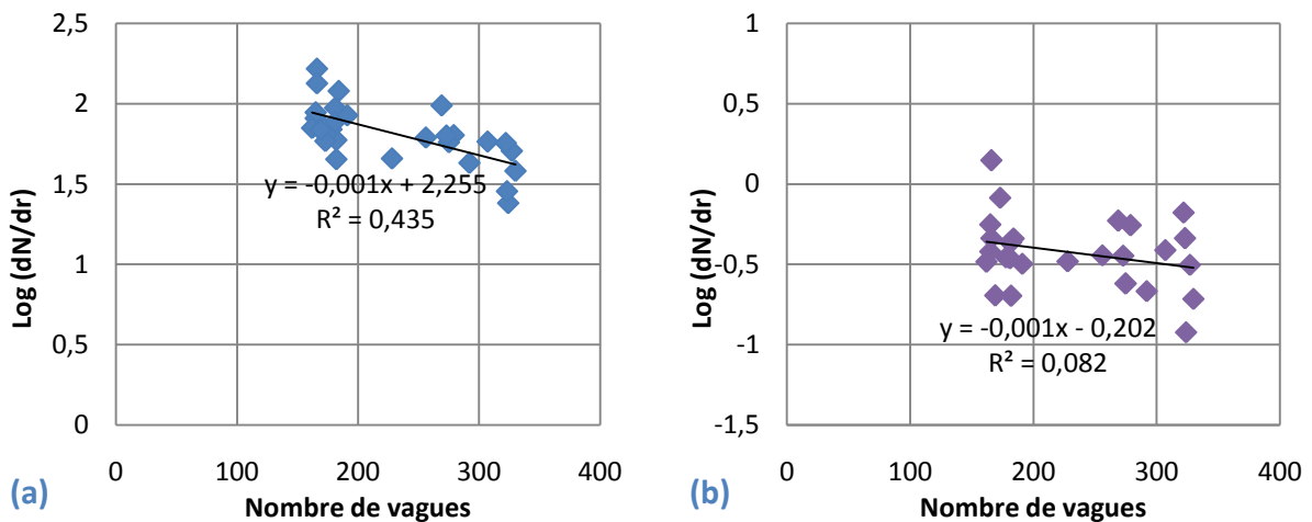
Figure 5-31 : Concentration en particules de 0.5 µm (a) et 5µm (b) en fonction du nombre de vagues, vent SO
