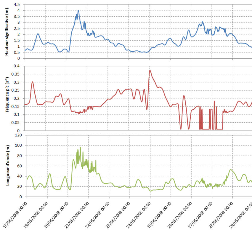
Figure 5-11 : Hauteur significative (trait plein bleu), fréquence pic (trait plein rouge) et longueur d'onde (trait plein vert) des vagues, houlographe PREVIMER
