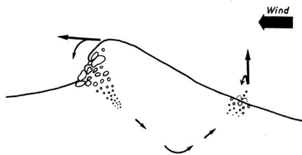
Figure 2-3 : Le déferlement à l'origine de la couverture moutonneuse (Resch 1982)
