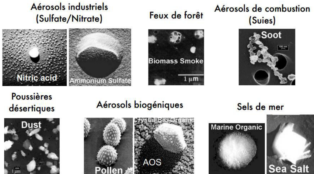
Figure 1-2 : Forme des aérosols atmosphériques
