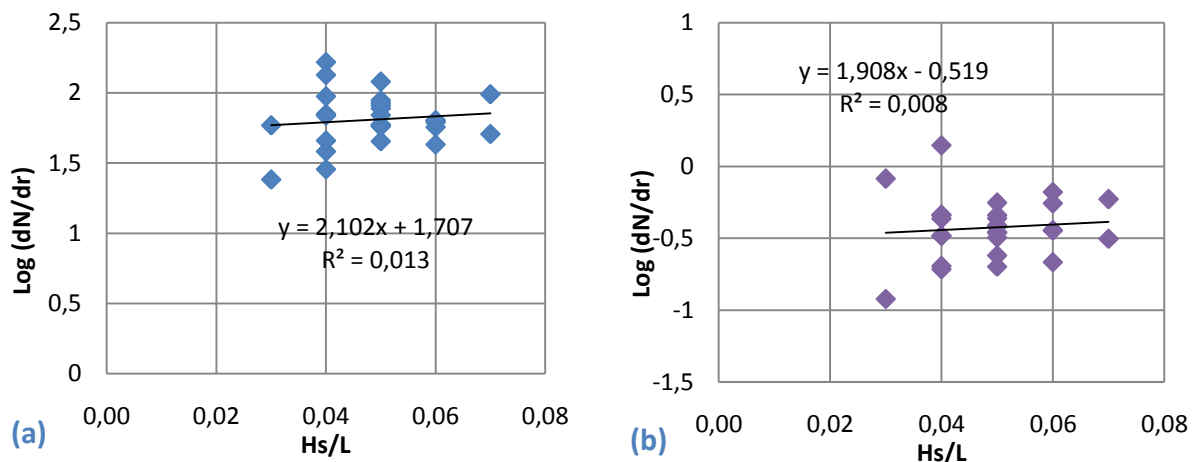
Figure 5-29 : Concentration en particules de 0.5 µm (a) et 5µm (b) en fonction de la cambrure significative des vagues, vent SO
