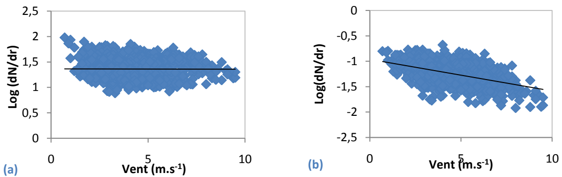
Figure 8-8 : Relation entre le logarithme de la concentration et la vitesse du vent à St Denis pour des particules de 0.5 µm (a) et 5 µm (b)
