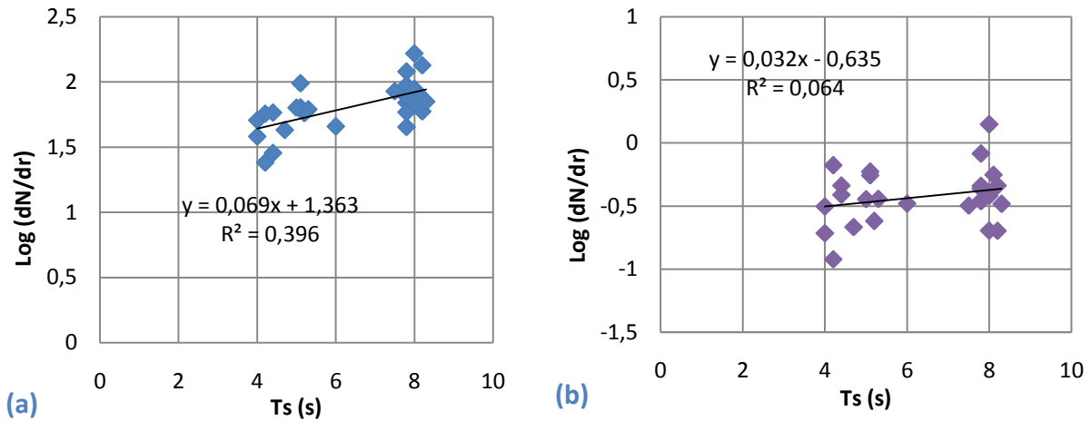
Figure 5-28 : Concentration en particules de 0.5 µm (a) et 5µm (b) en fonction de la période significative des vagues, vent SO
