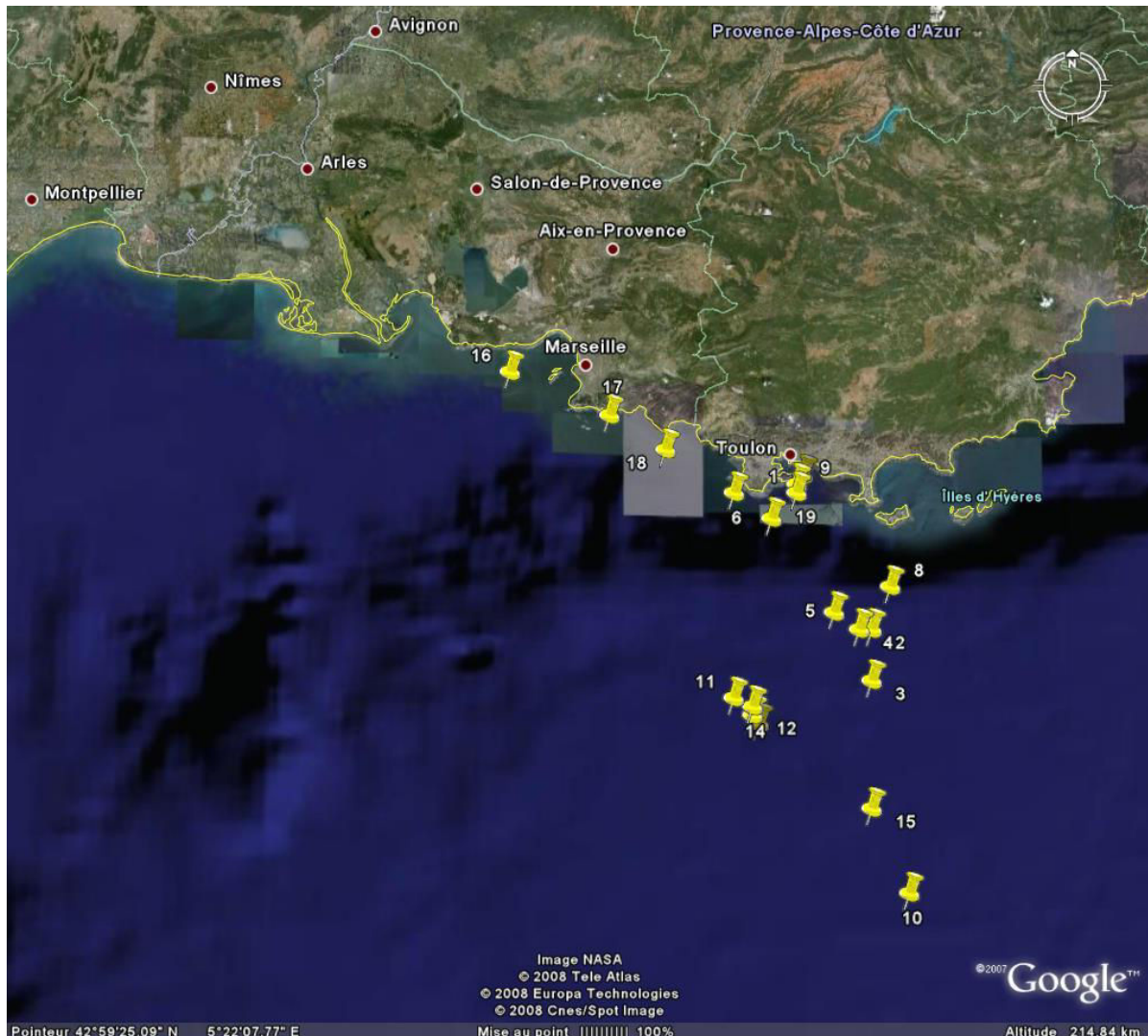
Figure 3-6 : Stations de mesures de l'Atalante durant la campagne MIRAMER 2008 (carte Google Earth)
