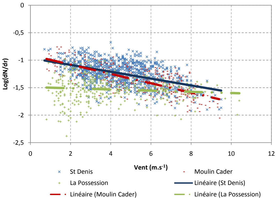
Figure 8-9 : Relation entre le logarithme de la concentration et la vitesse du vent à St Denis, Moulin Cader et La Possession pour des particules de 5 µm
