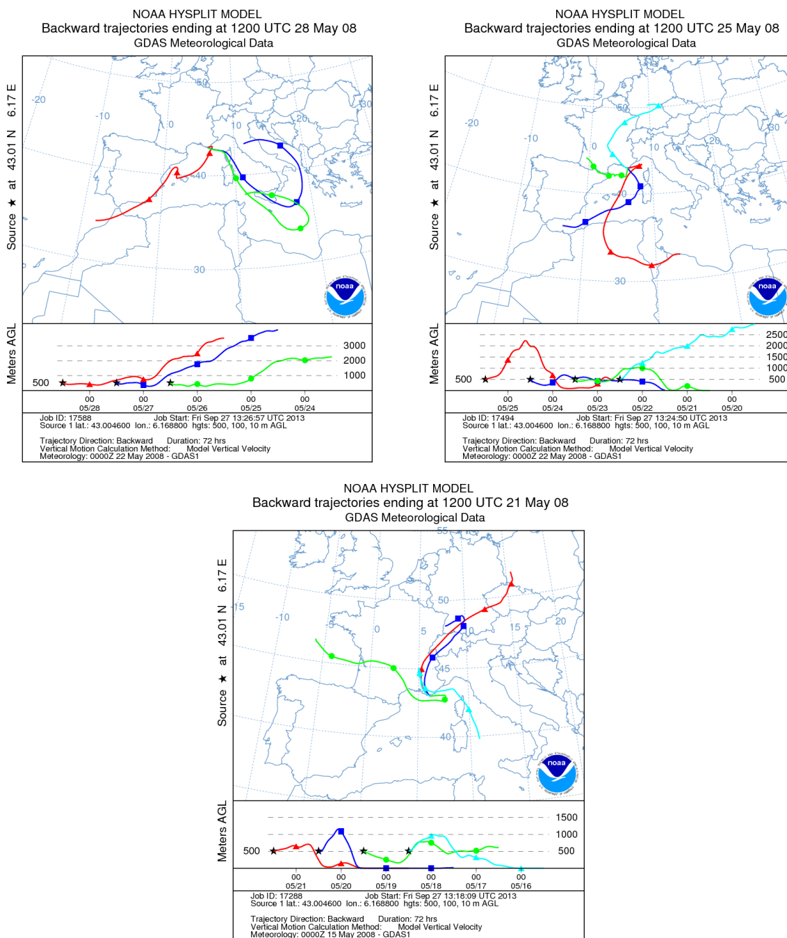
Figure 5-7 : Rétrotrajectoires des masses d'air du 18 au 28 mai 2008 dans la baie de Toulon Hyères (HYSPLIT)
