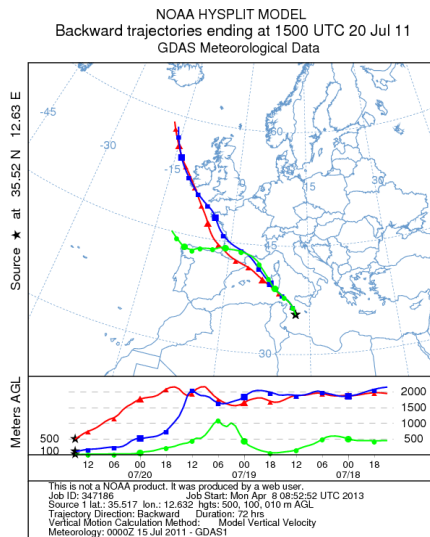
Figure 6-10 : Retro-trajectoire à Lampedusa le 20/07/2011 à 15h (Hysplit)
