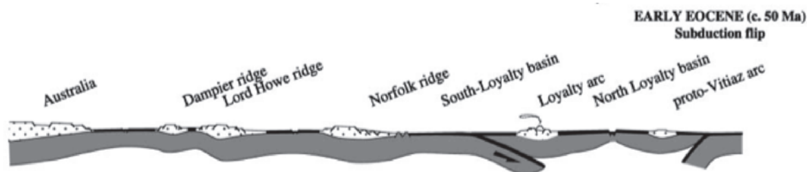
Figure I.4 Reconstitution géodynamique de la zone sud-ouest Pacifique à l'Éocène inférieur illustrant la phase de convergence qui mènera à l'obduction de la Nappe des Péridotites sur la ride de Norfolk à l'Éocène supérieur. D'après Cluzel et al. (2001).
