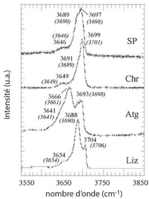
Figure II.1.7. Spectres Raman de référence pour les quatre variétés de serpentines (Lemaire, 2000). Les nombres en italiques sont montrés en guise de comparaison et sont issus de l'étude d'Auzende et al (2004). L'échelle des ordonnées est en unités arbitraires (u.a.). Liz : lizardite ; Atg : antigorite ; Chr : chrysotile ; SP : serpentine polygonale. Extrait de Ulrich (2010).
