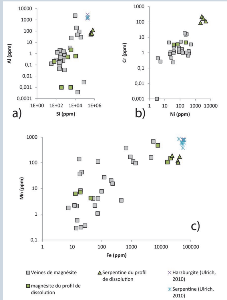
Figure 1 a,b,c) Diagrammes Al=f(Si), Cr=f(Ni) et Mn=f(Fe) où sont représentées les compositions élémentaires des veines de magnésite, des magnésites et des serpentines du profil de dissolution analysées dans cette étude ainsi que les compositions élémentaires d'échantillons de harzburgite et de serpentine provenant du massif de Koniambo analysées par Ulrich (2010).
