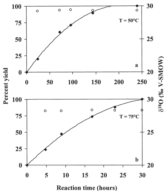
Figure III.3.3 Relation entre le taux d'avancement de la réaction entre acide phosphorique et magnésite (losange noir) et valeur du \delta^{18}\text{O} (cercle) à a) 50^\circ\text{C} et b) 75^\circ\text{C} en fonction du temps de réaction.
