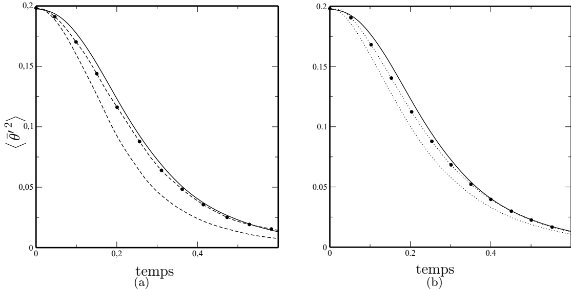
FIGURE 4.4 – Evolution de la variance statistique du scalaire résolu \langle \bar{\theta}^2 \rangle des SGE à \bar{\Delta} = 8\Delta . (a) : CM (-----) et EO-CM ( \bullet \bullet ). (b) : DEDM (.....) et EO-DEDM ( \bullet \bullet ). Le trait fort représente l'évolution de la variance de la SND filtrée.
