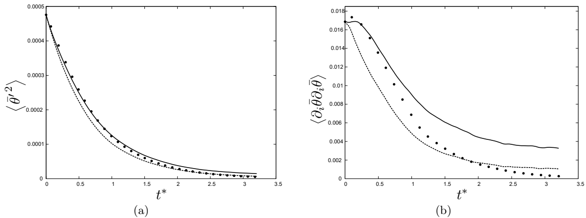
FIGURE 5.9 – Evolution de la variance (a) et de l’entropie (b) de scalaire résolu pour les modèles ACWM (—), DEDM (-----) et de la SND filtrée ( \bullet \bullet ) ( Re_\lambda = 90 , N_\theta = 64^3 ).
