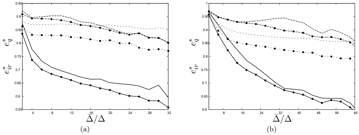
FIGURE 3.4 – Evolution des erreurs quadratiques des modèles GM (- - -), DSM (- - - -), DRGM (—) et de leurs erreurs irréductibles ( \bullet \cdot ) pour les bases de données Re_\lambda = 160 , Sc = 0.7 (a) et Re_\lambda = 90 , Sc = 16 (b)
