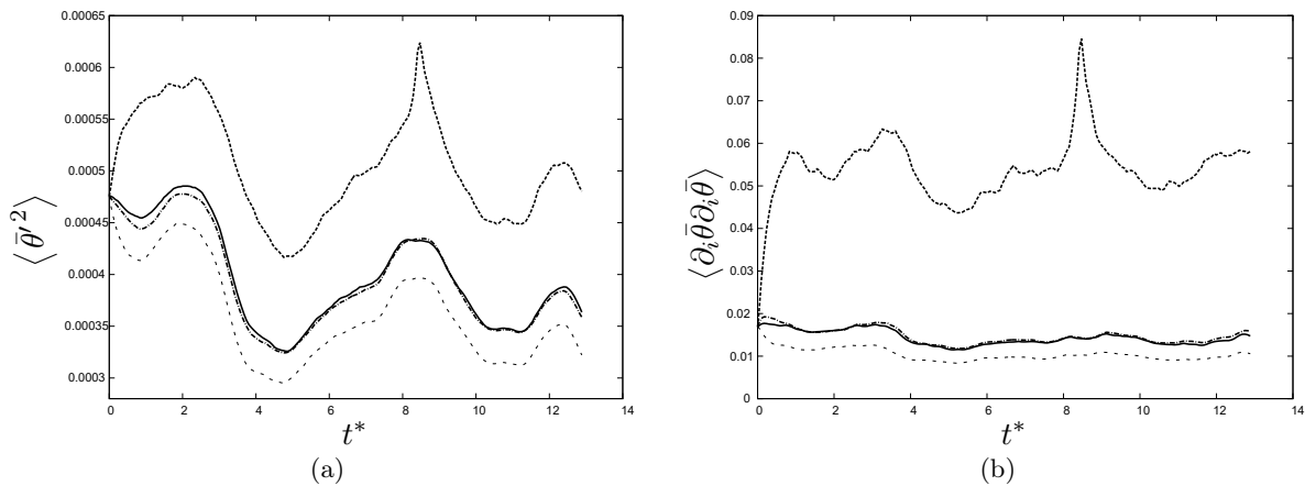
FIGURE 4.12 – Evolution de la variance du scalaire résolu (a) et évolution de l'ensrophie du scalaire (b), pour les SGE réalisées avec les modèles DEDM (- - -), DNTDM (- · - · -) et ANNM (· · · · ·) et pour la SND filtrée (—).
