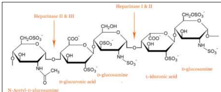
Figure 39 : Différentes spécificités de reconnaissance et de clivage au niveau des HS par les héparinases I, II et III de P.heparinus .
