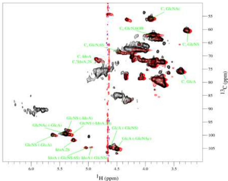
Figure 104 : Spectres RMN ^{13}\text{C} -HSQC d'HS cellulaires purifiés de cellules Caco-2 non-différenciées (noir) et différenciées (rouge). Les échantillons sont analysés à 37°C pendant 15h dans un spectromètre 600MHz (spectre rouge) ou 700MHz (spectre noir).
