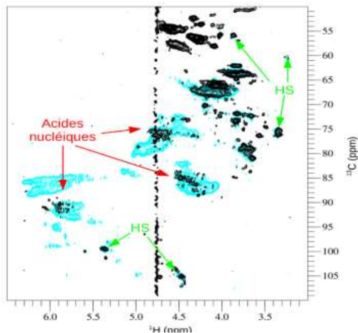
Figure 81 : Analyse par RMN de l'extrait d'HS de cellules HeLa marquées avant (spectre cyan) et après (spectre noir) digestion à la DNase I. Les spectres 13 C-HSQC sont partiellement attribués pour les HS (flèches vertes) et pour les acides nucléiques (flèches rouges).
