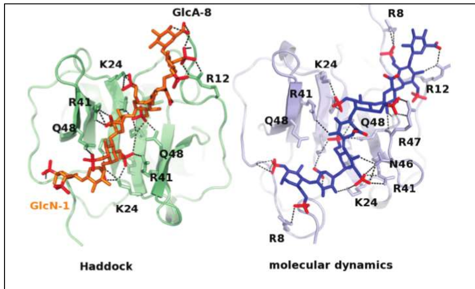
Figure 64 : Comparaison entre deux structures d'interaction CXCL12-dp8 d'héparosan modifié GlcNS,6S obtenue par la méthode d' amarrage moléculaire HADDOCK (gauche) et par dynamique moléculaire (droite). D'après (Laguri et al. 2011).
