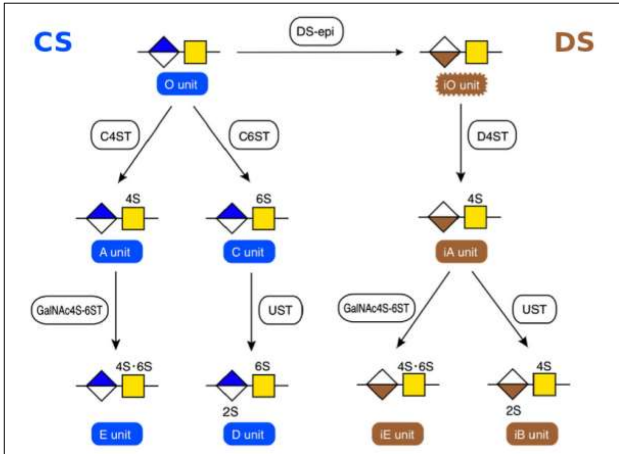
Figure 26 : Diagramme schématisé des voies de modification biosynthétiques des chaînes de CD/DS. D'après (Mikami & Kitagawa 2013).
