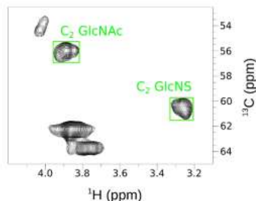
Figure 92 : Spectre RMN ^{13}\text{C} -HSQC des déplacements chimiques \text{H}_2 - \text{C}_2 des glucosamines d'HS. Les encadrés verts représentent les bornes utilisées pour l'intégration des pics. L'échantillon est analysé à 37°C pendant 16h dans un spectromètre 600MHz équipé d'une cryosonde.
