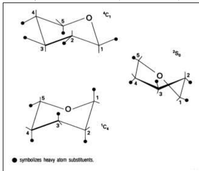
Figure 61 : Trois conformations principales de basse énergie de l' \alpha -L-iduopyranose retrouvé en solution. D'après (Mulloy et al. 1993).
