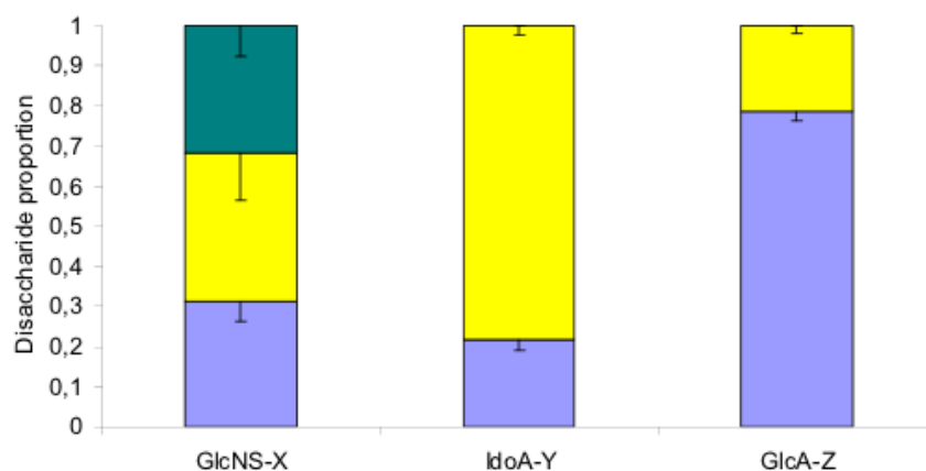
Figure 97 : Caractéristiques des unités disaccharidiques des HS de cellules HeLa. Proportion des disaccharides des HS de cellules HeLa dans lesquels une GlcNS±6S est associée à X = GlcA (bleu), IdoA (jaune) ou IdoA,2S (vert) ; un IdoA est associé à Y = GlcNS (bleu) ou GlcNS,6S (jaune) ; un GlcA est lié à Z = GlcNAc (bleu) ou GlcNS (jaune).
