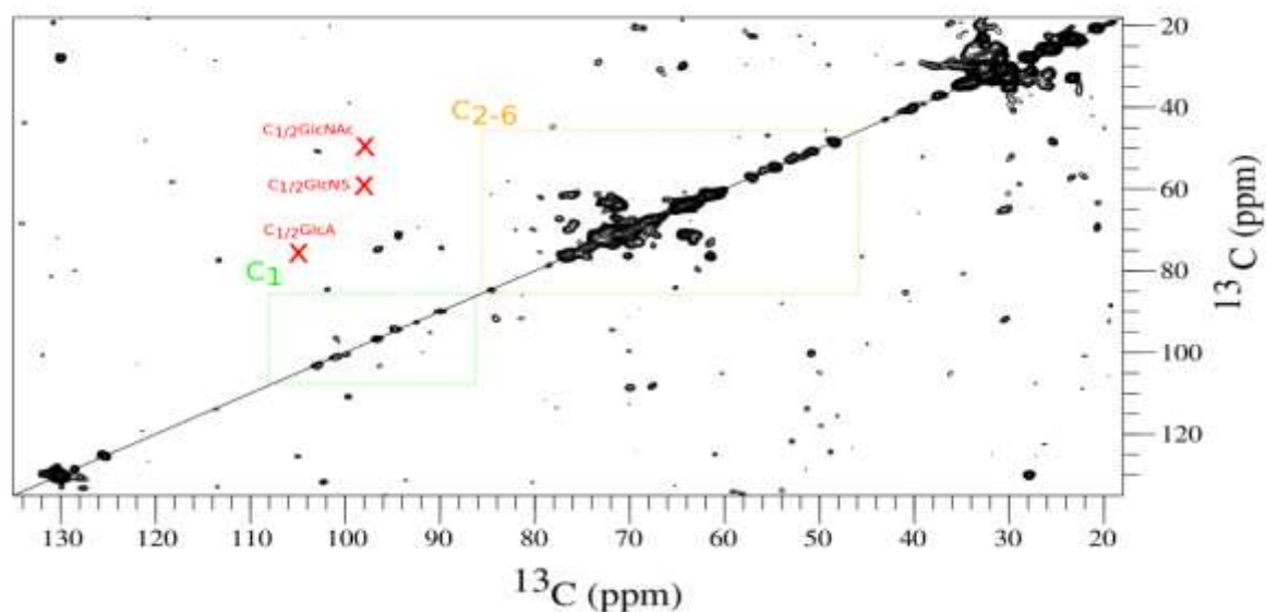
Figure 109 : Expérience par ssNMR de corrélation ^{13}\text{C} - ^{13}\text{C} après excitation directe du ^{13}\text{C} et en utilisant le couplage scalaire lors du transfert ^{13}\text{C} - ^{13}\text{C} . Ce spectre a été enregistré sur cellules entières HeLa à 4°C, avec un temps expérimental de 15h et à une vitesse de rotation à l'angle magique de 3,4 kHz. L'encadré vert correspond aux corrélations attendues pour les carbones anomériques et l'encadré orange aux autres corrélations attendues pour les GAG. Les corrélations \text{C}_1 - \text{C}_2 attendues pour les GlcNAc, GlcNS et GlcA sont indiquées par une croix rouge.
