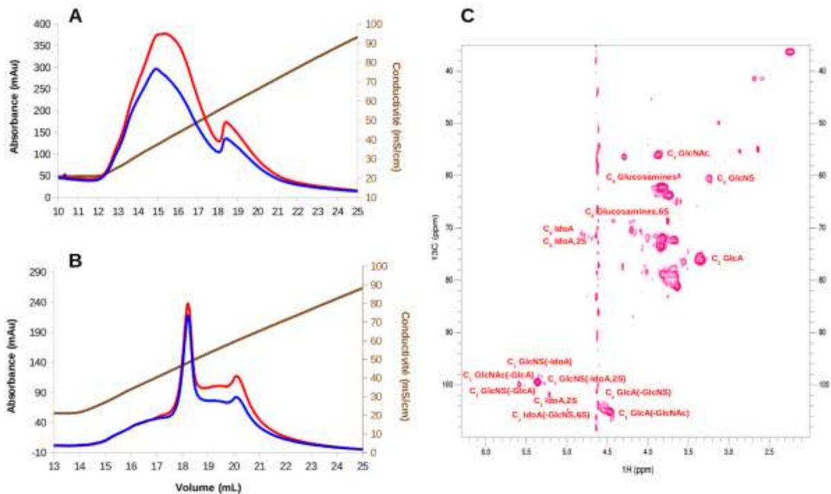
Annexe 3 : Purification et analyse RMN d'un échantillon-type d'HS issu de MEF ndst-1 -/- . Les extraits d'HS de MEF KO sont purifiés par chromatographies successives après digestion à la trypsine (A) et à la DNase I (B). Toutes les fractions d'éluion absorbant à 260nm (rouge) et 280nm (bleu) sont gardées pour analyse par RMN. Les spectres sont enregistrés sur un spectromètre 600MHz à 37°C pendant 16h et attribués d'après Guerrini et al 2005 (C)
