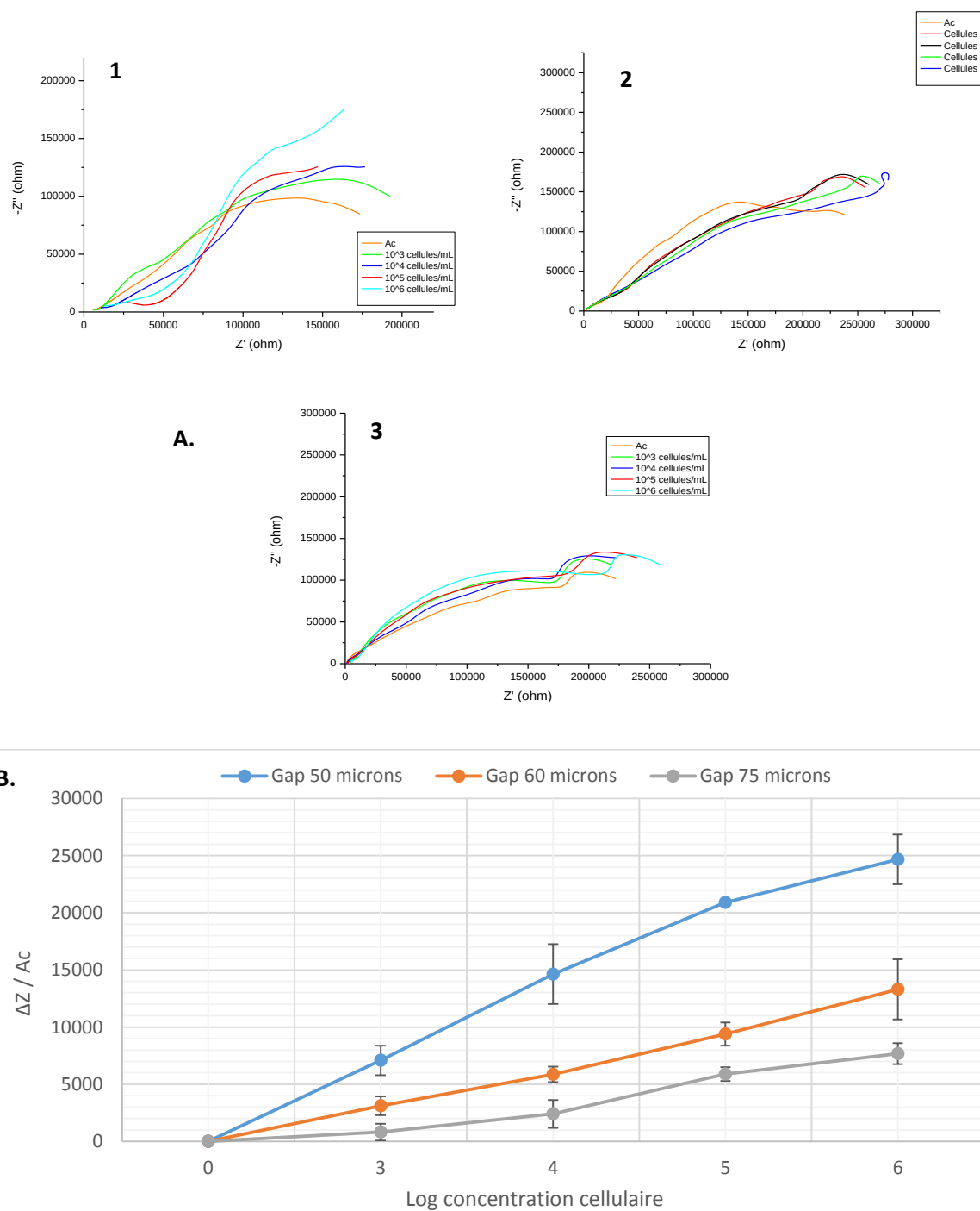
Figure III-25 : A- Exemples de diagrammes de Nyquist obtenus en mode faradique après incubation en présence de suspensions cellulaires dans une gamme de 10^3 à 10^6 cellules/mL pour des électrodes interdigitées ayant différentes valeurs de gap 1) 50 \mu\text{m} 2) 60 \mu\text{m} et 3) 75 \mu\text{m} , B- Variation correspondante du module d'impédance mesuré à 100Hz en fonction du logarithme de la concentration cellulaire
