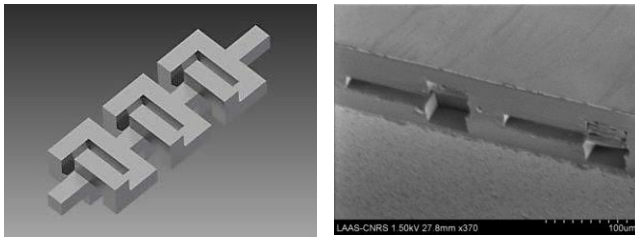
Figure A2- 4 : Schéma d'un micromélangeur et image MEB en coupe
