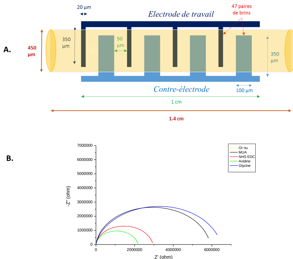
Figure IV-5 : A- Structure et dimensions de la microélectrode interdigitée et de la canalisation microfluidique, B- Exemple de diagramme de Nyquist de fonctionnalisation fluide de microélectrodes d'or interdigitées sur wafer verre
