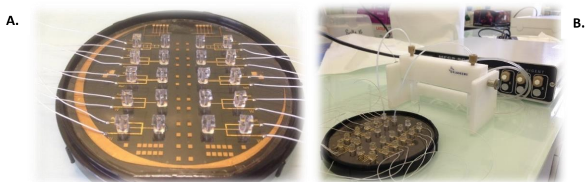
Figure III-18 : A- Wafer verre avec canalisations microfluidiques, plots PDMS et connectiques extérieurs, B- Exploitation du wafer par le FLUIGENT®
