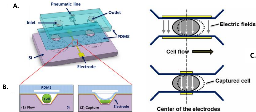
Figure I-13 : Schéma du dispositif, A-Composition des trois couches, B- vue en coupe du canal microfluidique, capable de piéger une cellule unique, C- Champs électriques
