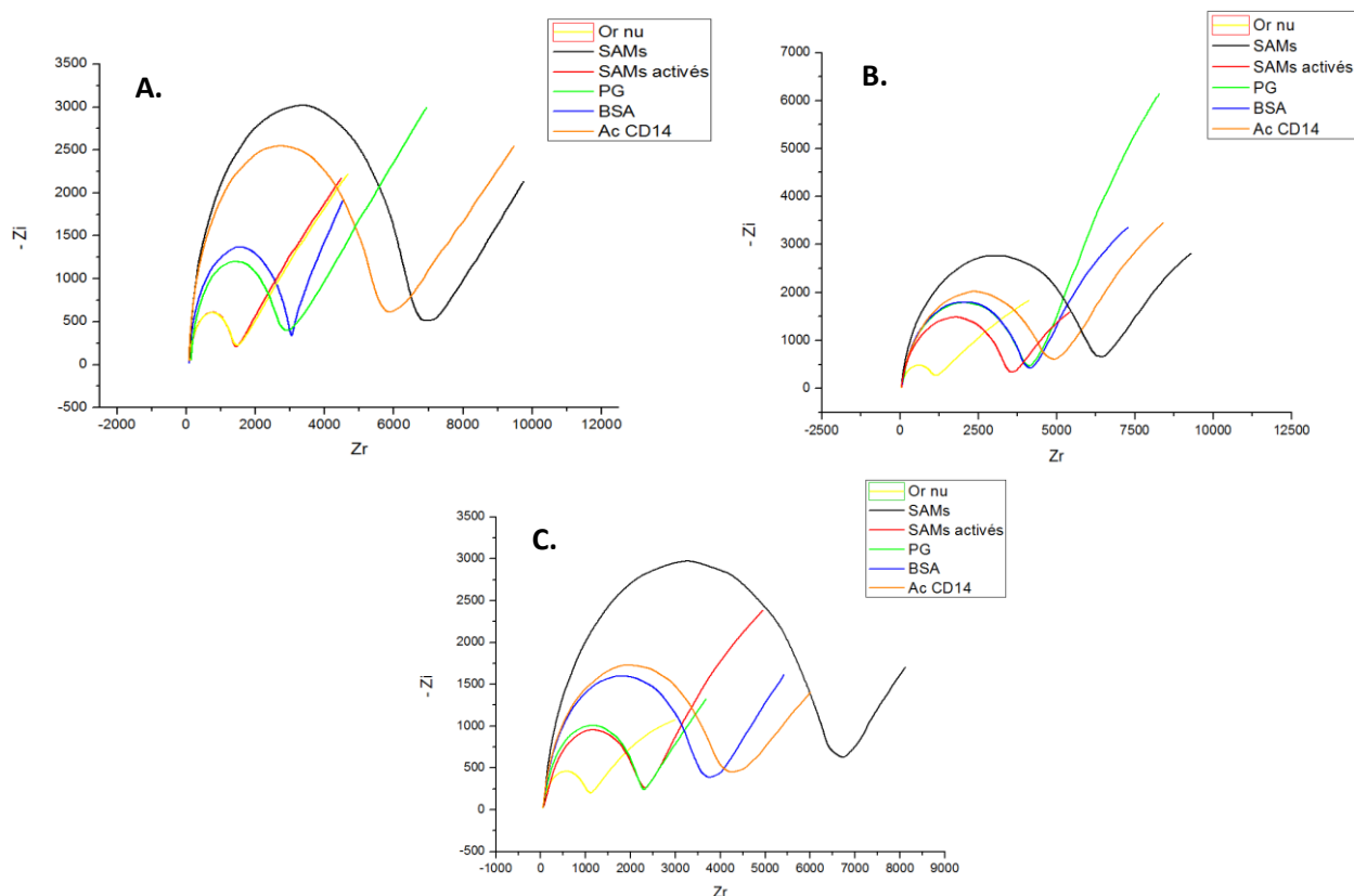
Figure III-12 : Exemples de diagrammes de Nyquist obtenus en mode faradique ( \text{Fe(CN)}_6^{3-/4-} 5mM) après chaque étape de fonctionnalisation sur microélectrodes d'or en mode statique, A-Simples, B-Multiples, C-Interdigitées
