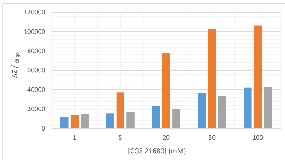
Figure IV-18 : Variation du module d'impédance à 100 Hz pour des électrodes fonctionnalisées par c-di-AMP après passage de 10^5 CHO-A2a/mL ayant été préalablement incubée en fluide en présence de différentes concentrations en CGS 21680: 1, 5, 20, 50 et 100 mM
