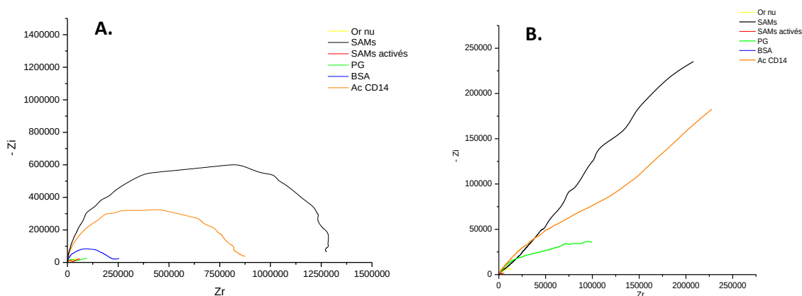
Figure III-7 : Exemples de diagrammes de Nyquist obtenus après fonctionnalisation de microélectrodes, A-multiples et B-interdigitées
