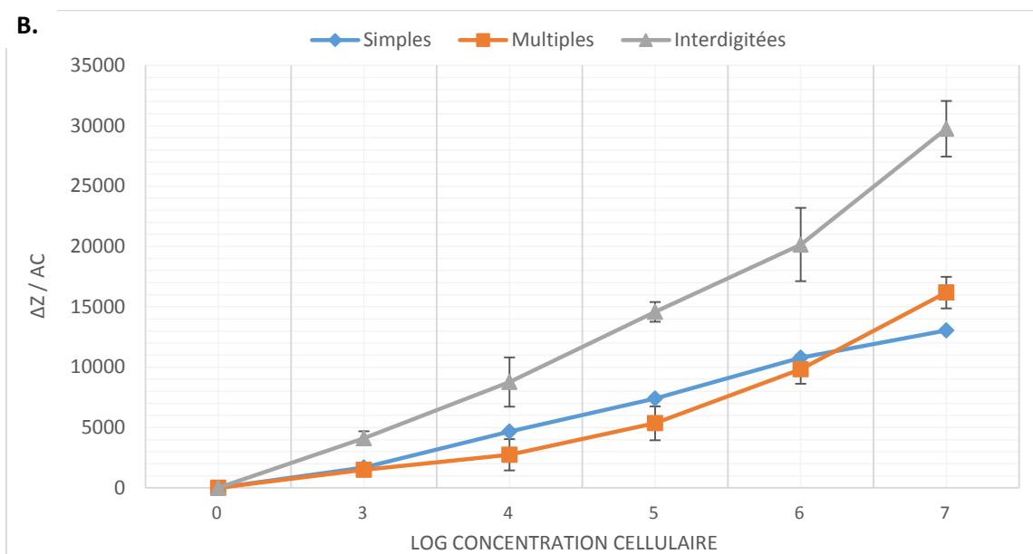
Figure III-22 : A-Exemples de diagrammes de Nyquist (1-Simples 2-Multiples 3-Interdigitées) obtenus en mode faradique après incubation en fluide en présence de suspensions cellulaires dans une gamme de 10^3 à 10^7 cellules/mL, B- Variation correspondante du module d'impédance mesuré à 100Hz en fonction du logarithme de la concentration cellulaire
