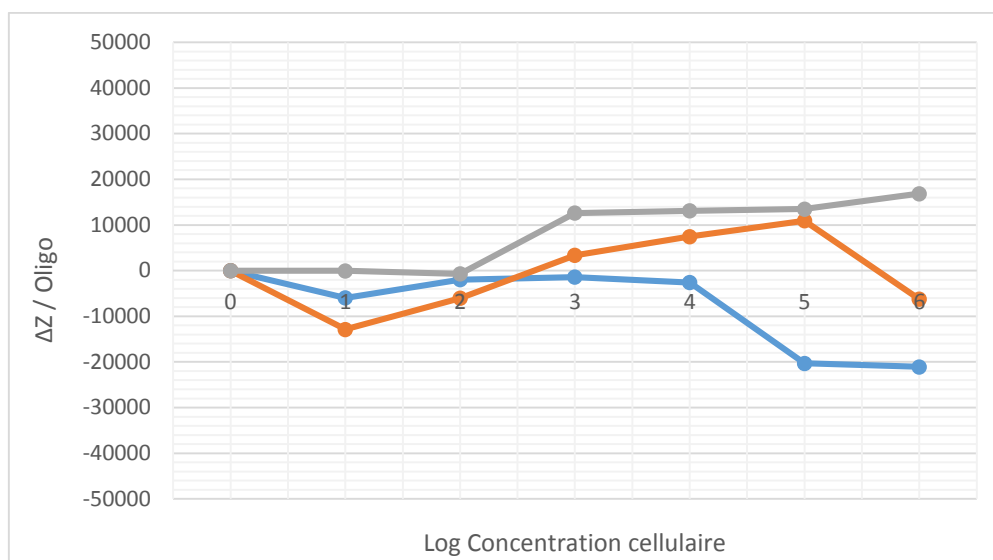
Figure IV-11 : Variation du module de l'impédance mesurée à 100 Hz par rapport à la couche d'oligomères pour 3 puces fonctionnalisées c-di-AMP après incubation en présence de suspensions de différentes concentrations en CHO ne surexprimant pas A2a
