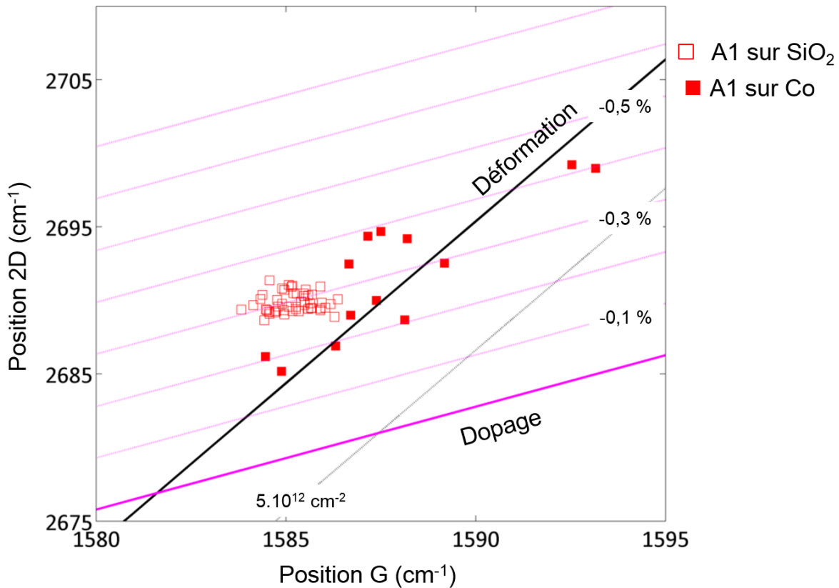
Figure 57 : Effet de la contrainte et du dopage sur le graphène après synthèse sur film mince de Co puis après son transfert sur \text{SiO}_2(285 \text{ nm})/\text{Si} .
