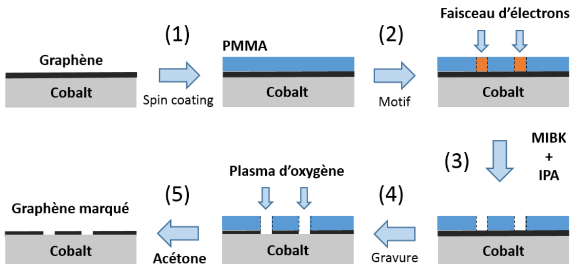
Figure 13 : Schéma des étapes du procédé de marquage des échantillons par lithographie électronique.
