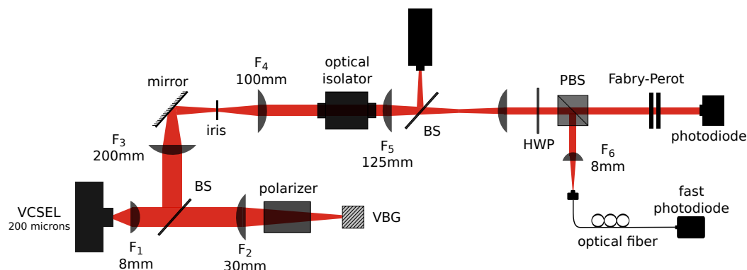
FIGURE 2.2 – Schéma expérimental complet détaillant le système de détection. F_3 , F_4 , F_5 , F_6 et F_7 : lentilles de focales f_3 = 200 mm, f_4 = 100 mm, f_5 = 125 mm, f_6 = 50 mm et f_7 = 8 mm. Optical isolator : isolateur optique comprenant un rotateur de Faraday et deux polariseurs. BS : lame séparatrice de faisceaux, réflectivité R = 10\% . HWP : lame demi-onde. PBS : cube séparateur de faisceaux polarisant.
