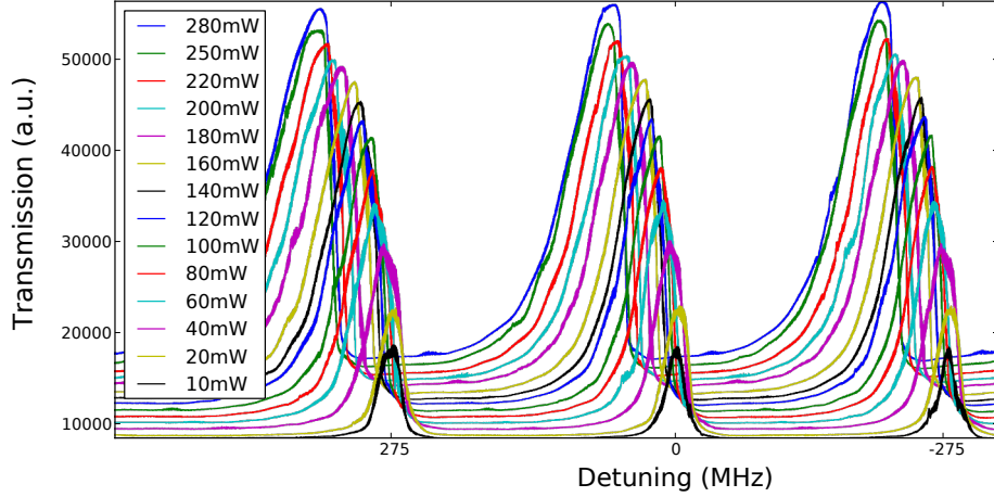
FIGURE 3.8 – Courbes de transmission de la cavité en anneau en modifiant le désaccord en fréquence lorsqu’il est opéré sous le seuil ( I = 1600 mA). Du bas vers le haut la puissance d’injection augmente exhibant ainsi l’évolution des résonances en fonction de ce paramètre.
