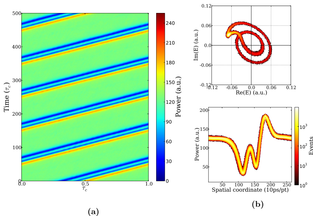
FIGURE 4.4 – Présentation des caractéristiques d’un soliton de phase de charge +2. a) Diagramme spatio-temporel indiquant une propagation rectiligne sur 500 \times \tau_c . b) histogramme des trajectoires de la phase parcourues durant 1000 \times \tau_c (haut) et histogramme réalisé en superposant la forme du soliton sur 20\,000 \times \tau_c (bas).
