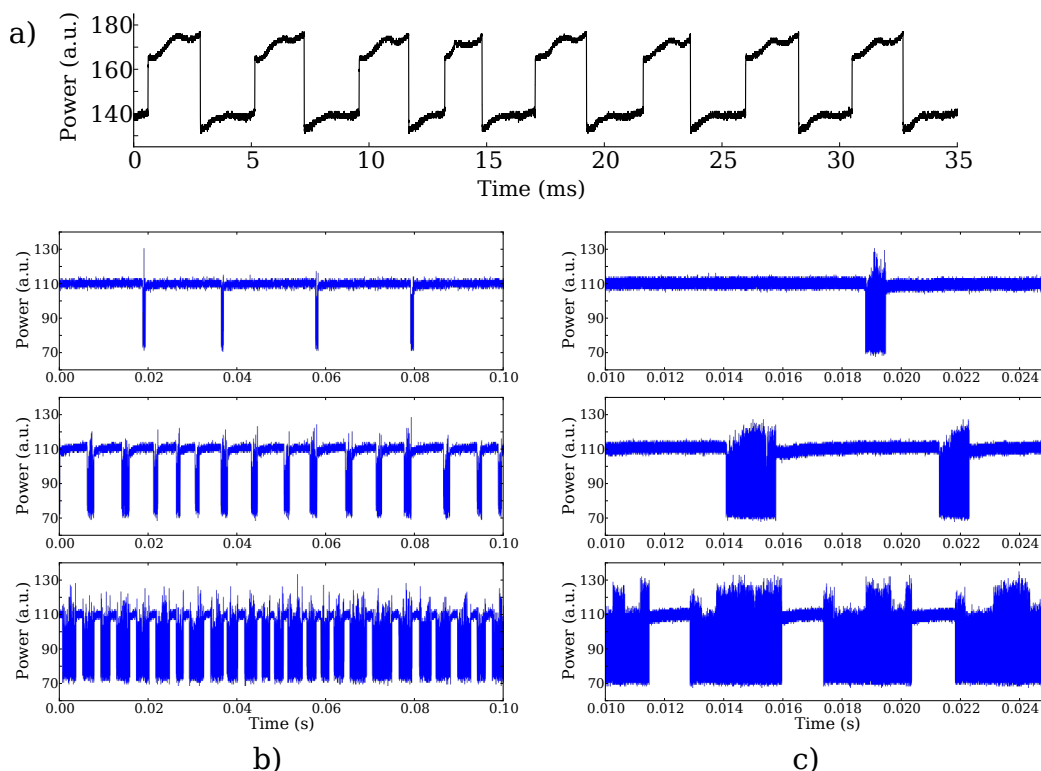
FIGURE 3.19 – Traces temporelles correspondant à la dynamique de van der Pol–Fitzhugh–Nagumo. a) Evolution de l’intensité durant 35 ms détectée grâce à la photodiode lente. b) traces temporelles longues de 100 ms, acquises avec la détection rapide pour \Delta croissant (du côté négatif) en descendant. c) Zoom de 10 à 25 ms sur les traces montrées en dans b) . L’échantillonnage de la détection rapide est choisi à 25 MHz pour permettre d’observer les temps longs tout en montrant la présence de la dynamique rapide. Les données en a) sont obtenues pour les mêmes paramètres que b) et c) en bas.
