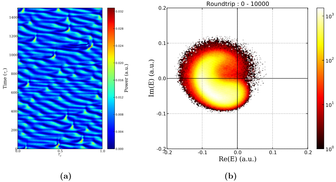
FIGURE 3.26 – a) Diagramme spatio-temporel présentant les évènements extrêmes qui se forment sur l'état faiblement modulé, tracé sur 1500 \times \tau_c . b) Histogramme effectué sur les valeurs de la phase durant 10\,000 \times \tau_c indiquant un temps d'occupation important dans une petite zone du plan complexe (en blanc et jaune).
