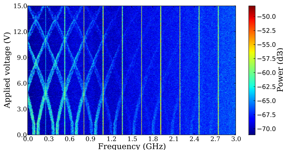
FIGURE 3.10 – Evolution du spectre de puissance en fonction du désaccord en fréquence lorsque le laser placé au dessus de seuil ( I = 2000 mA) bat avec le faisceau d’injection (système non forcé). L’axe vertical correspond à la tension appliquée au piezo-électrique impliquant une variation du \Delta . Les lignes verticales correspondent au battement entre les modes de la cavité, alors que les courbes intermédiaires proviennent du battement de ces modes avec le faisceau d’injection. L’échelle de couleur code pour la puissance en échelle logarithmique.
