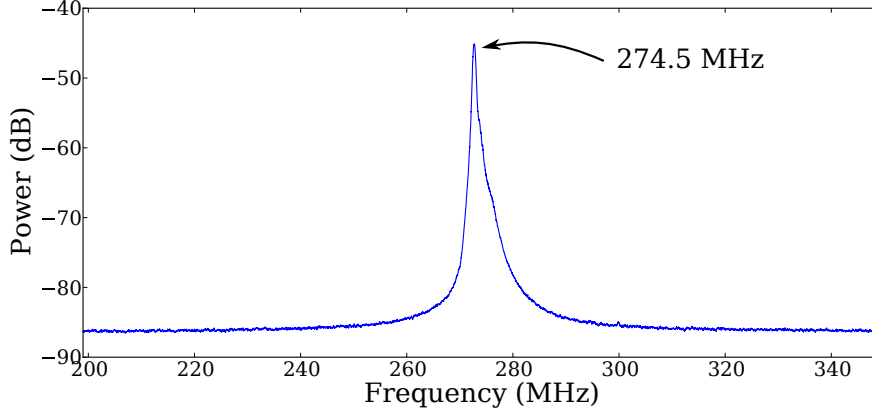
FIGURE 3.5 – Spectre de puissance mesuré autour du premier pic donnant une valeur de l’espacement entre modes à 274.5 MHz.
