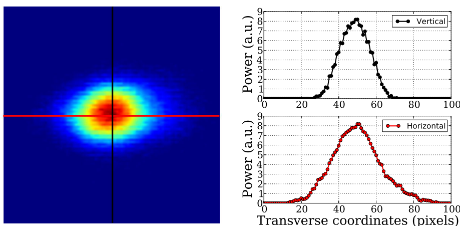
FIGURE 2.5 – A gauche : zoom sur le champ proche du soliton sur une grille de 100 \times 100 pixels. L'échelle de couleur va du bleu au rouge, i.e. des faibles au fortes intensités. A droite : coupes verticales et horizontales du soliton. Les lignes verticale (noire) et horizontale (rouge) sur le champ proche indiquent la position de ces coupes.
