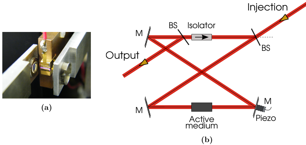
FIGURE 3.1 – Gauche : photo de l'amplificateur optique dans sa monture, entouré des deux collimateurs. Droite : Représentation schématique du laser en anneau montrant la géométrie du laser anneau. M : miroir, BS : lame séparatrice de faisceau, Piezo : matériau piezo-électrique sur lequel est fixé un des miroirs, Isolator : isolateur optique constitué d'un rotateur de faraday entre deux cubes polariseurs.
