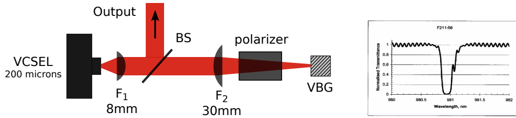
FIGURE 2.1 – Gauche : schéma expérimental du laser à solitons de cavité. VCSEL : laser à cavité verticale émettant par la surface (@975 nm). F1 : lentille asphérique de courte focale f_1 = 8 mm et distance de travail WD_1 = 5.92 mm. F2 : lentille de focale f_2 = 30 mm. Polarizer : polariseur linéaire Glen Thomson orienté verticalement, indice de réfraction 1.66, longueur 25mm. VBG : réseau de diffraction de Bragg en volume. Droite : courbe de transmission du VBG en fonction de la longueur d’onde.
