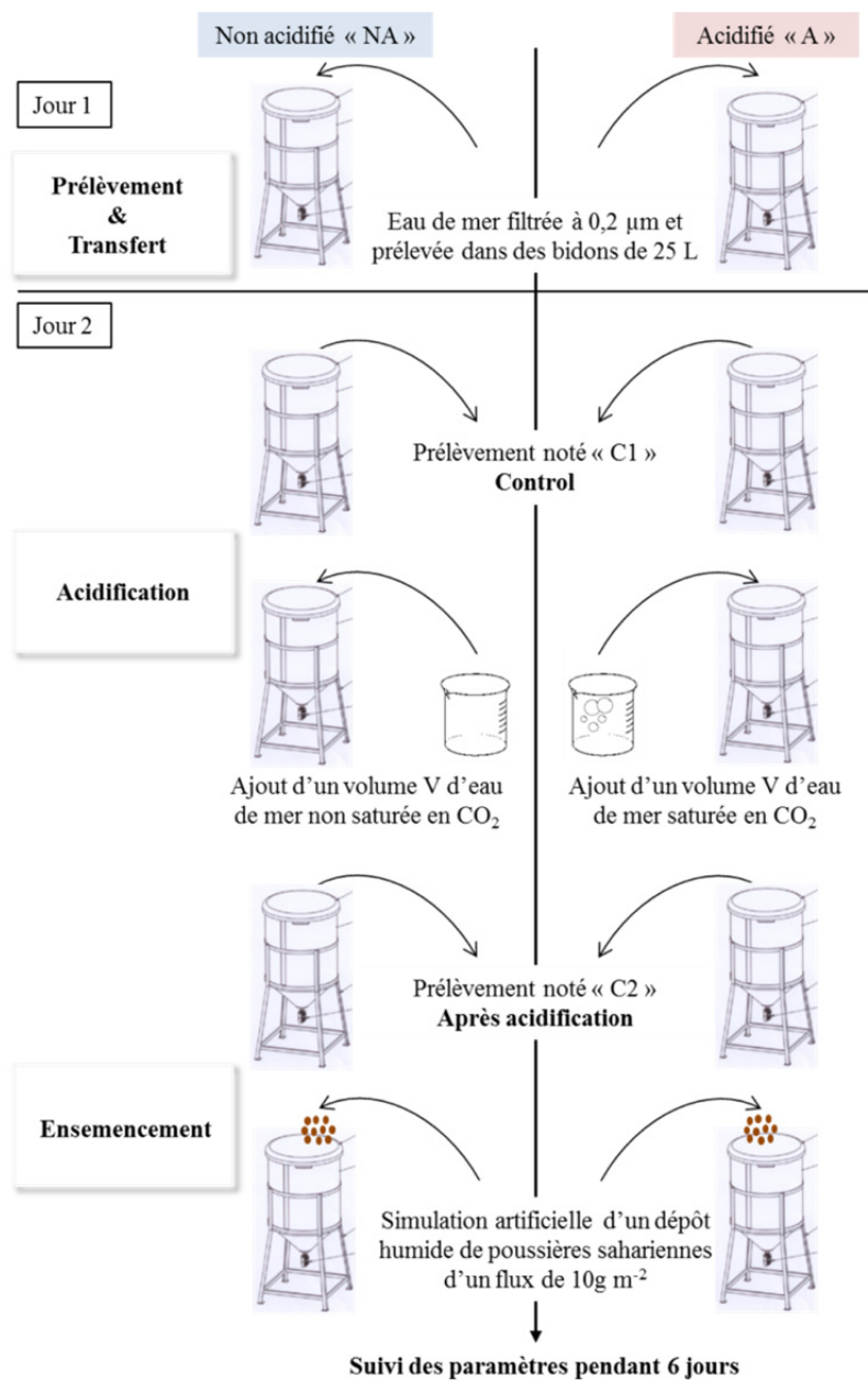
Figure II.13 : Méthodologie des expériences en minicosmes dans le cadre du projet CHIPIE
