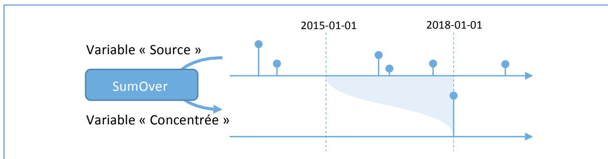
Figure 47 : Un exemple d'application de l'opération « SumOver »
