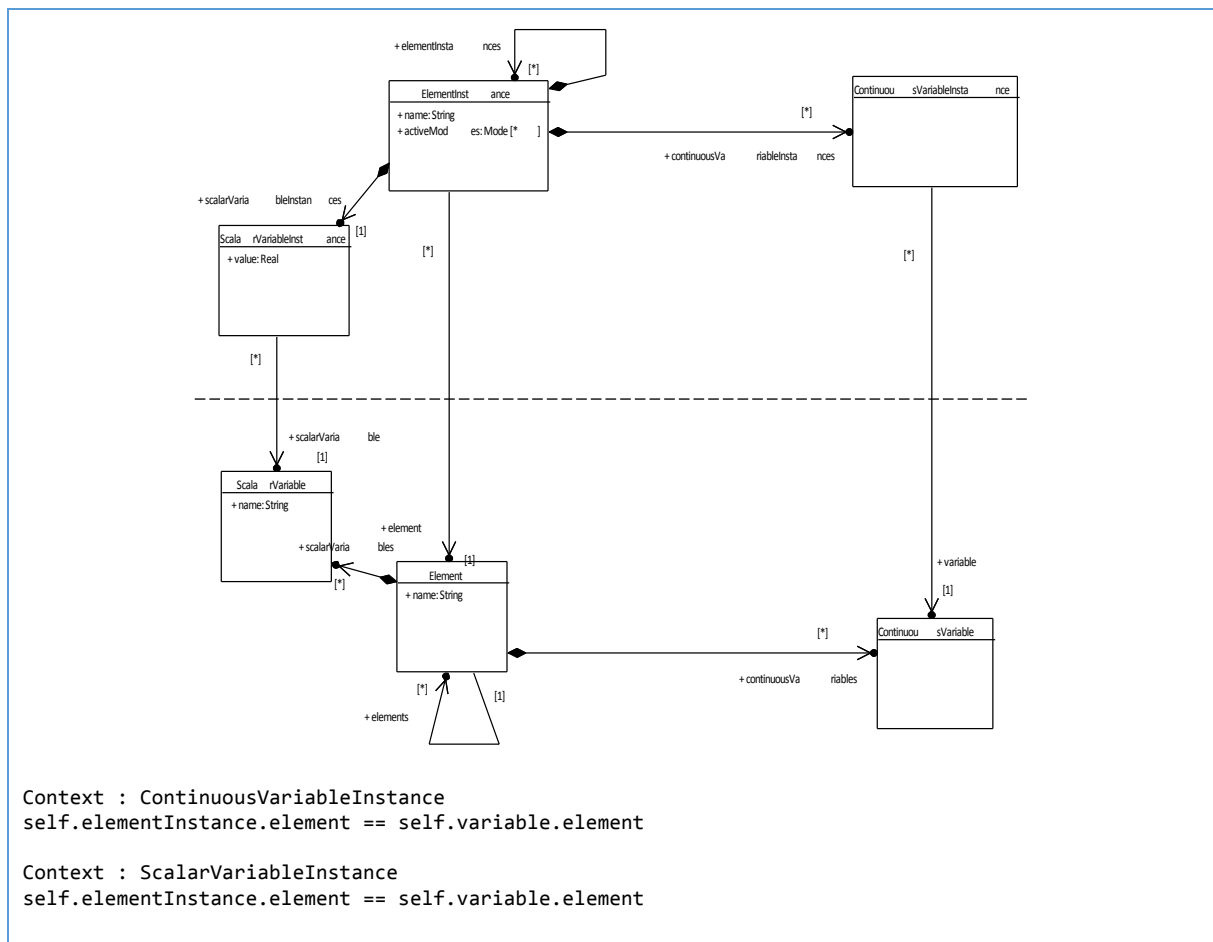
Figure 25 : La contrainte entre les variables d'instances et leur variable
