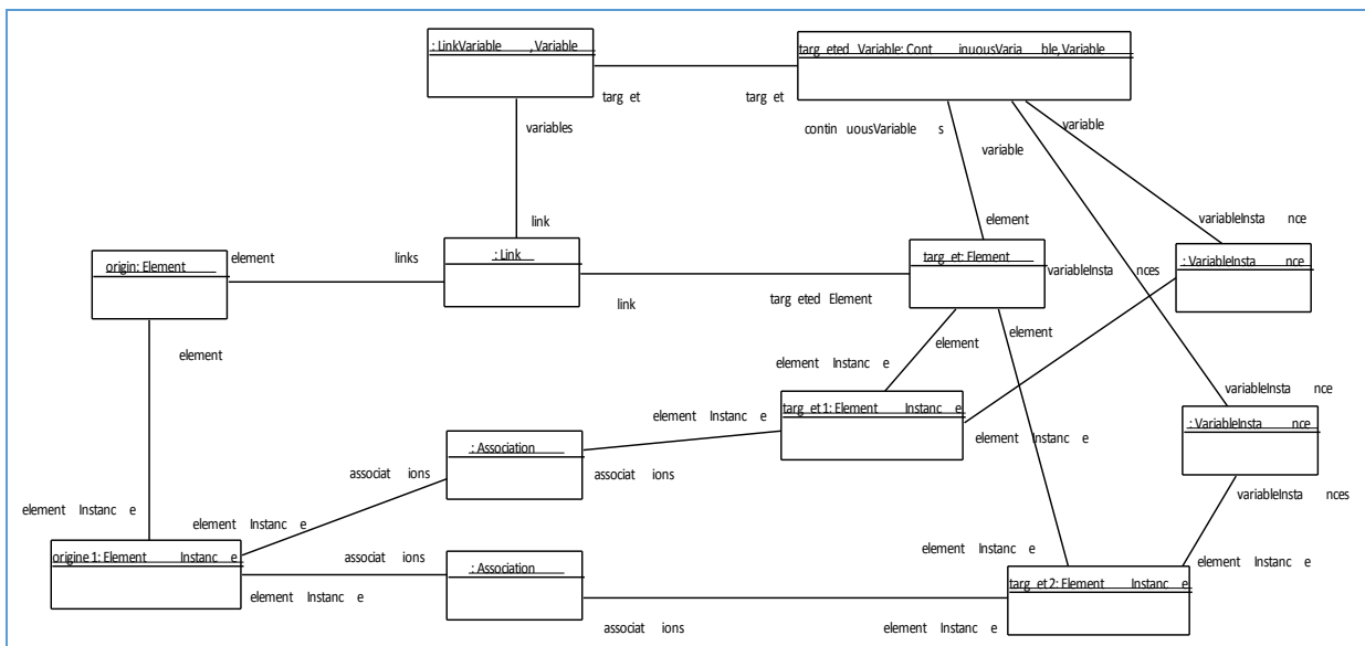
Figure 27 : Un diagramme d’instance illustrant le besoin d’agréger les variables de lien
