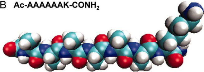
Figure I-6 : Structure de lipopeptides détergents 32
