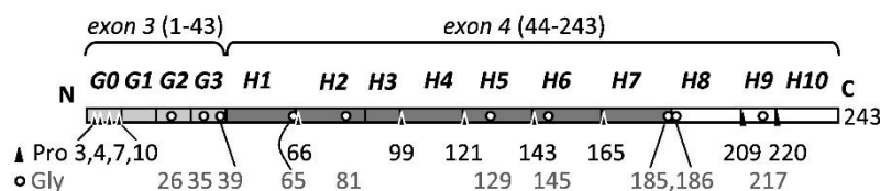
Figure I-8 : Organisation de la protéine Apolipoprotéine A-1. Les positions des prolines (triangles) et glycines (cercles) sont marquées par les nombres. 70
