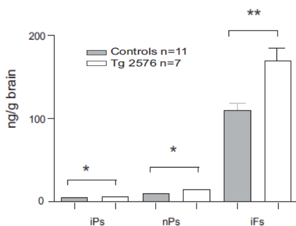
Figure 12 : Quantité d'IsoPs (iPs), NeuroPs (nPs) et NeuroFs (noté ici iFs) dans le cortex cérébral de souris transgéniques et de souris saines 59 * p < 0,05 ; ** p < 0,01
