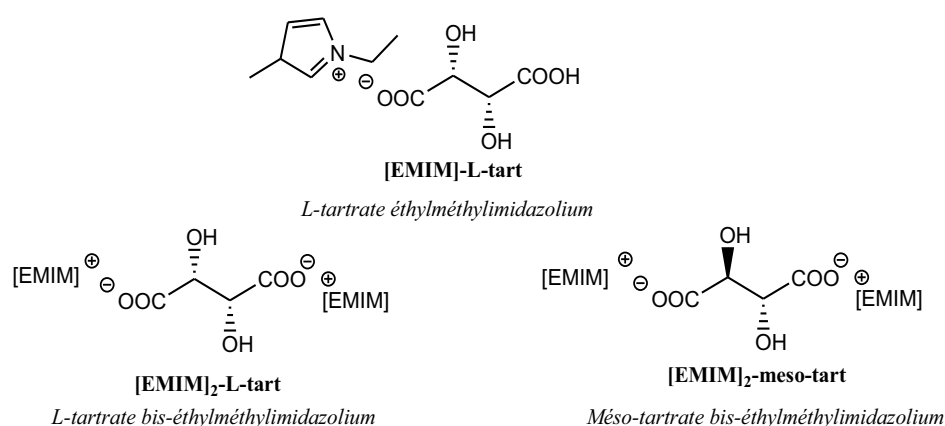
Figure 29 : Sels de tartrates étudiés
