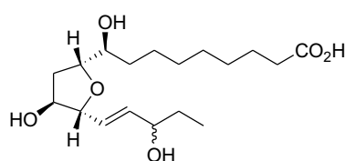
ent -16-( RS )-9- epi -ST- \Delta^{14} -10-PhytoF
