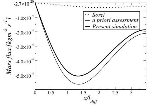
(D) Mass fluxes for O_2 species
