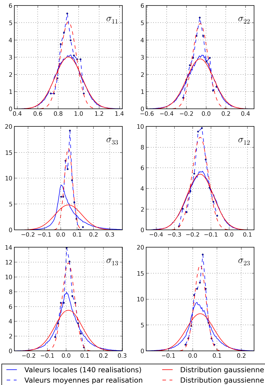
Figure 2-7: Distribution des contraintes au sein des N grains centraux d'orientation [B.O.B.] (valeurs normalisées par \langle \sigma_{11} \rangle_V ).
