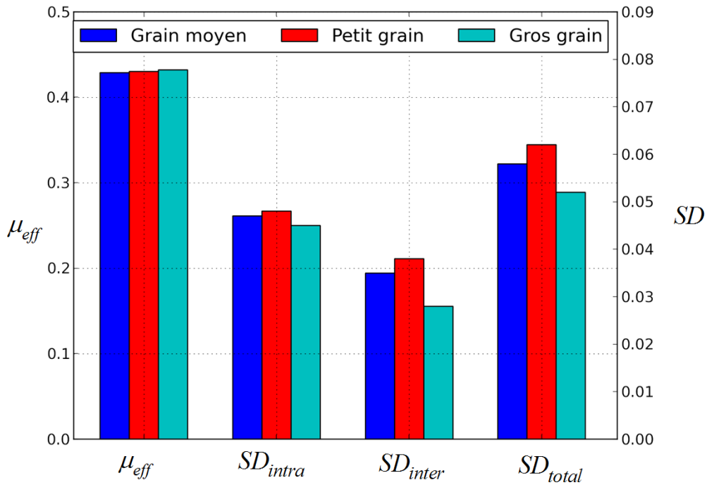
Figure 3-51 : Facteur de Schmid effectif et écarts-types associés au sein des N grains centraux dans les 3 cas étudiés.
