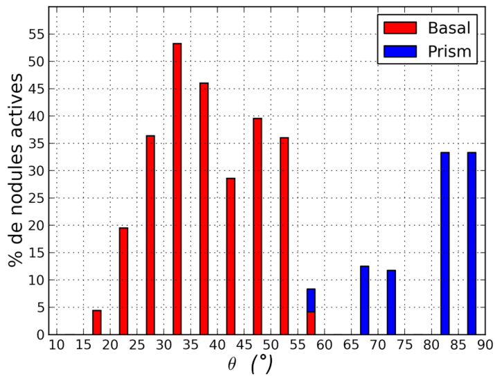
Figure 5-31 : Fraction totale de nodules activés par classe d'angle \theta .
