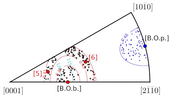
Figure 5-37 : Orientation des nodules analysés dans la zone 1 (observée à faible grandissement) associés à l'une des 4 orientations de référence considérées ([B.O.b.], [B.O.p.], [5] et [6]).
