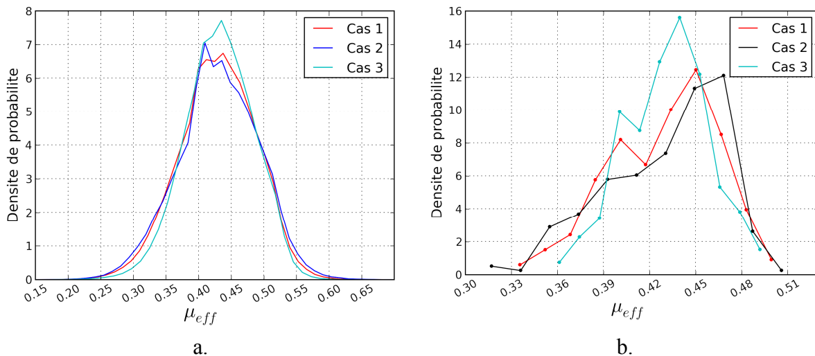
Figure 3-52: Distribution du facteur de Schmid effectif pour les 3 cas étudiés: a. valeurs locales ; b. valeurs moyennes par grain.
