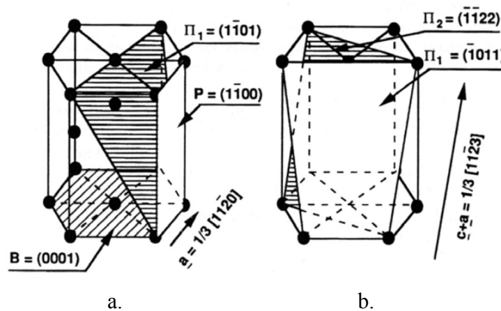
Figure 1-15 : Illustrations des systèmes de glissement des matériaux à structure cristalline hexagonale compacte (HC) : a. plans de glissement basal, prismatique et pyramidal de 1 ère espèce associés à une direction de glissement de type a; b. plans de glissement pyramidal de 1 ère et 2 ème espèce associés à une direction de glissement de type a+c.
