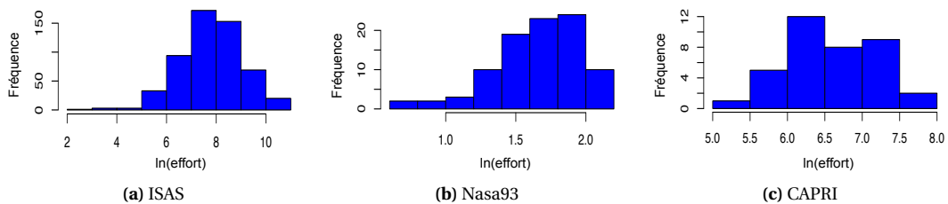
FIGURE 4.7 – Histogrammes des \ln(\text{effort}) des bases de données ISAS, Nasa93 et CAPRI
