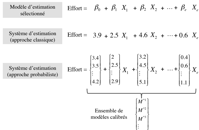
FIGURE 3.2 – Approche classique et approche probabiliste de construction de système d'estimation d'effort
