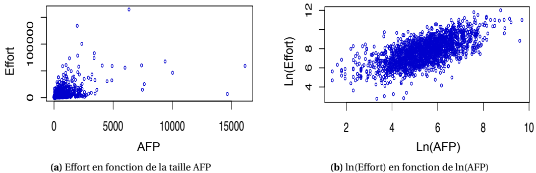
FIGURE 4.1 – Linéarisation de la relation entre l'effort et la taille (AFP) par l'application du logarithme
