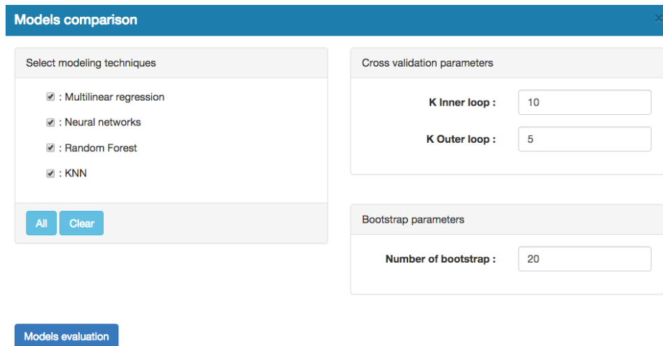
FIGURE 4.15 – Copie de l'écran de la fenêtre de sélection de modèles d'estimation
