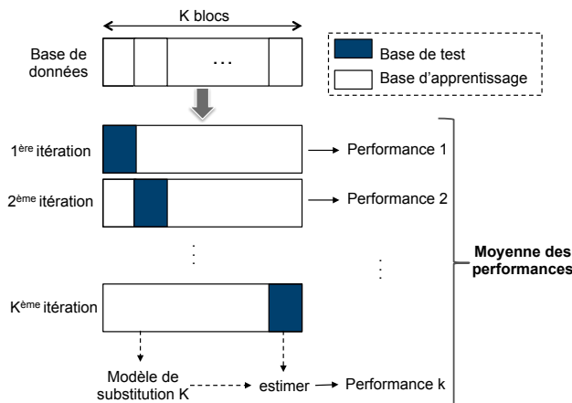
FIGURE 1.11 – Procédure de la validation croisée "k-fold"
