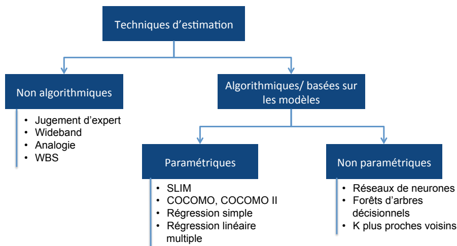
FIGURE 1.2 – Classification des techniques d'estimation d'effort
