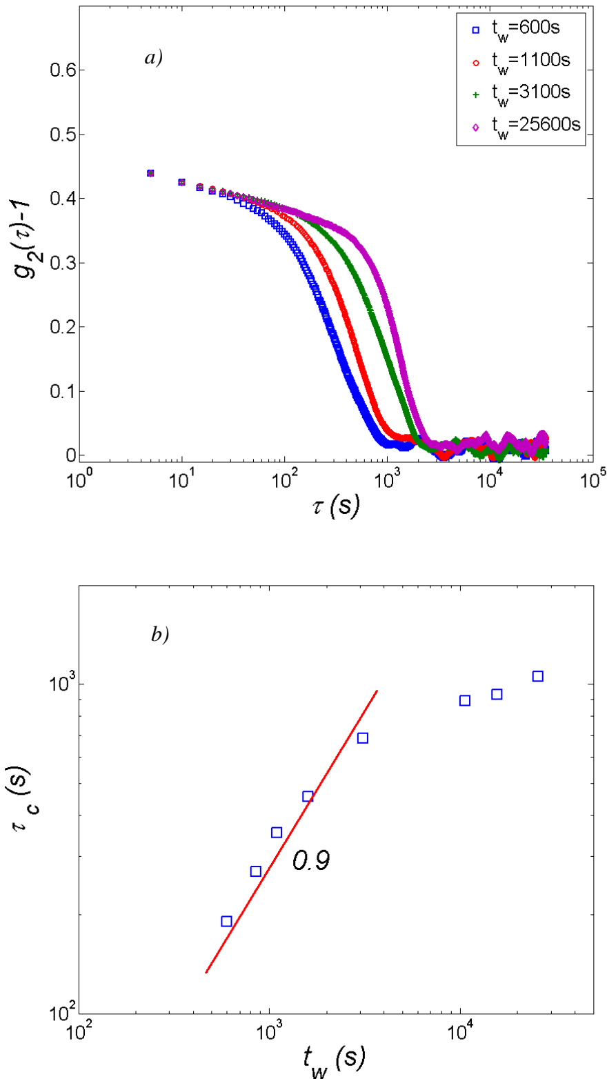
Figure 3-34. a) La fonction de corrélation d'intensité g_2(\tau) - 1 en fonction du retard \tau pour différents âges de l'échantillon t_w . Ces résultats sont issus de la moyenne temporelle de C_1(t, \tau) . b) Le temps de décroissance \tau_s du g_2(\tau) - 1 en fonction de l'âge de l'échantillon.
