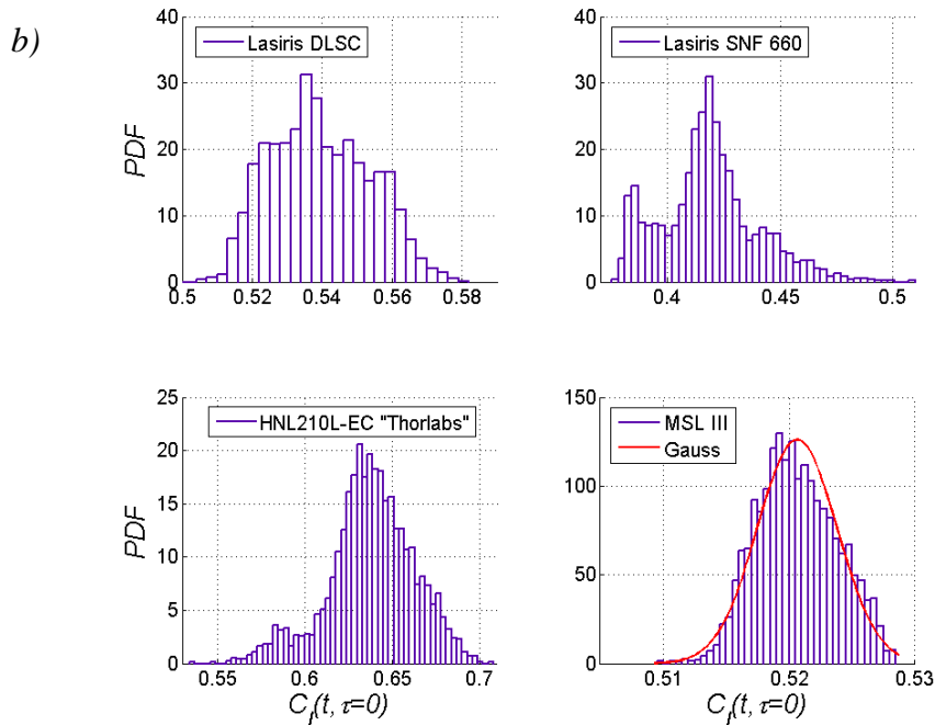
Figure 3-22. a) Degré de corrélation à retard nul C_f(t, \tau = 0) mesuré dans le cas d'un solide « PDMS » avec l'utilisation de plusieurs lasers. Encart : le spectre de Fourier issu de l'analyse fréquentielle du C_f(t, \tau = 0) pour chaque laser. b) Densité de probabilité pour un retard \tau = 0 . Température contrôlée à 23^\circ\text{C} \pm 0.15^\circ\text{C} .
