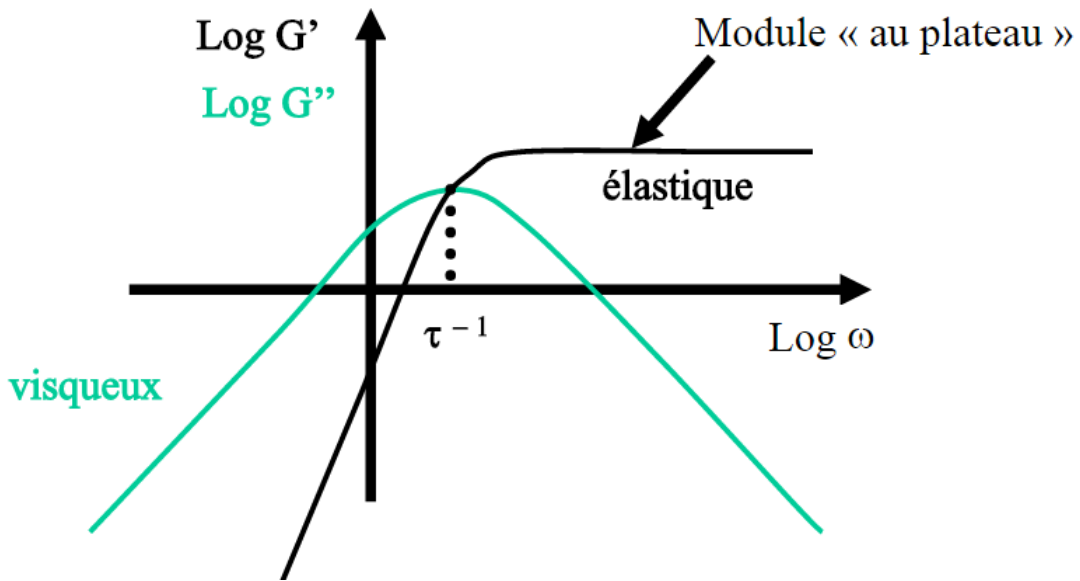
Figure 1-11. Représentation schématique des modules viscoélastiques d'un fluide de Maxwell [ http://slideplayer.fr/slide/2606449/ ].
