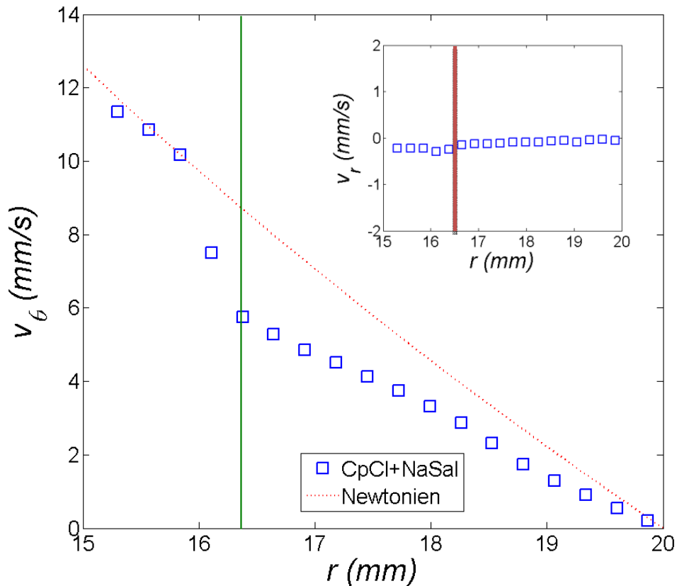
Figure 5-17. Vitesse orthoradiale en fonction du rayon à taux de cisaillement constant \dot{\gamma} = 3\text{s}^{-1} pour une solution concentrée du CpCl+NaSal (25+6% en poids) à 25°C. Données collecté à l'état stationnaire et moyenné sur un temps T_{\text{exp}}=0.5 s. pointillés en rouge : profil de vitesse théorique pour un fluide newtonien. Encart : vitesse radiale en fonction du rayon.
